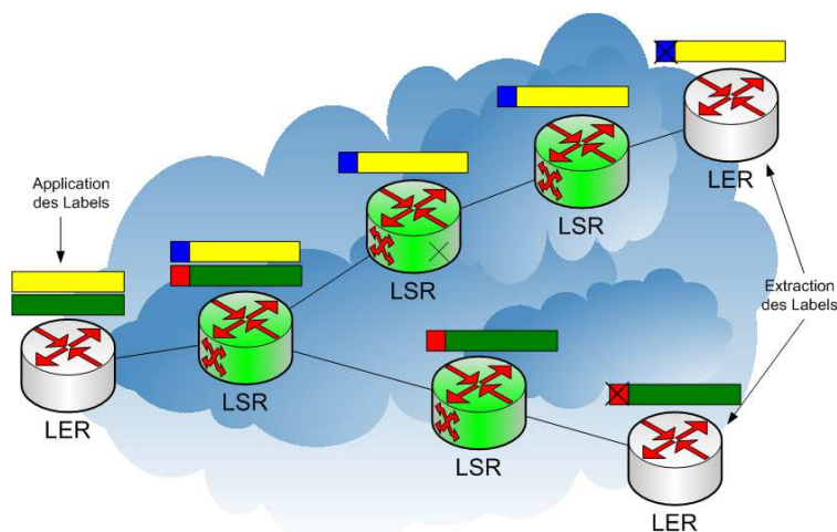
Figure 3 : Réseau MPLS
