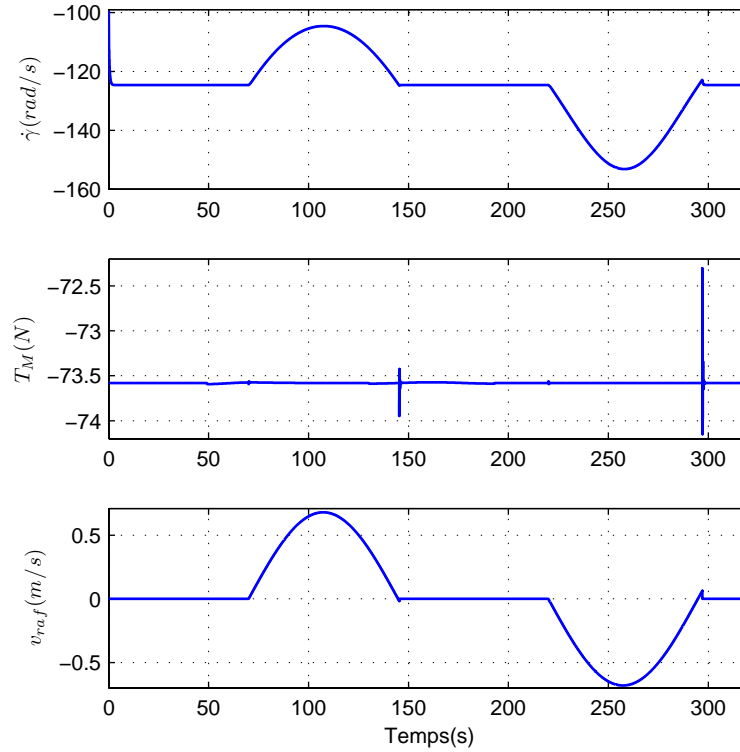
Fig. 4.5: Variations de \dot{\gamma} , de T_M et de v_{raaf}
