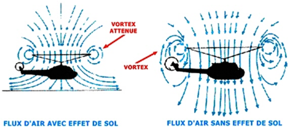
Fig. 2.26: L'effet de sol [4]
