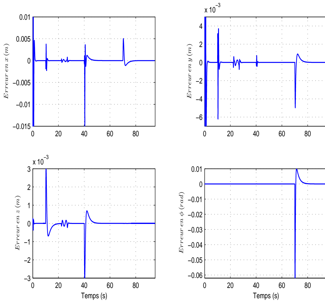
Fig. 5.13: Les erreurs de suivi en utilisant la commande AADRC
