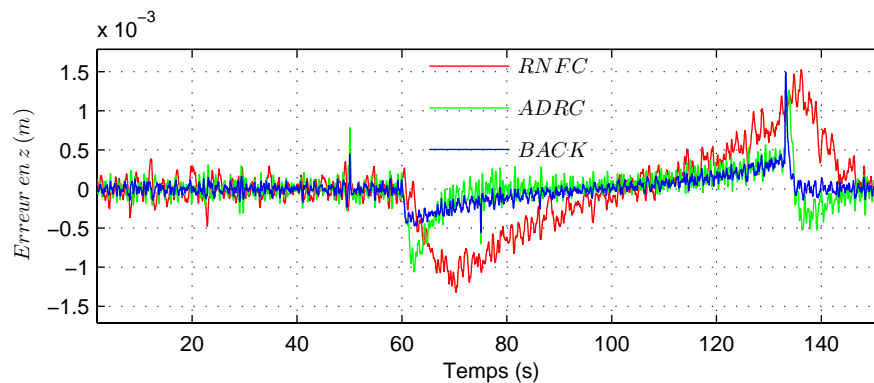
Fig. 4.29: Utilisation d'une rafale de vent importante v_{raf} = 3m/s
