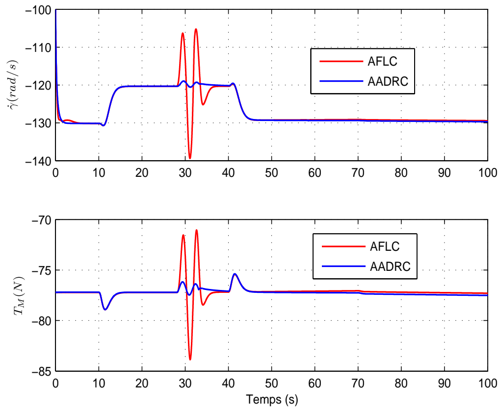
Fig. 5.17: La vitesse de rotation du rotor principal \dot{\gamma}(\text{rad/s}) et la force de poussée T_M
