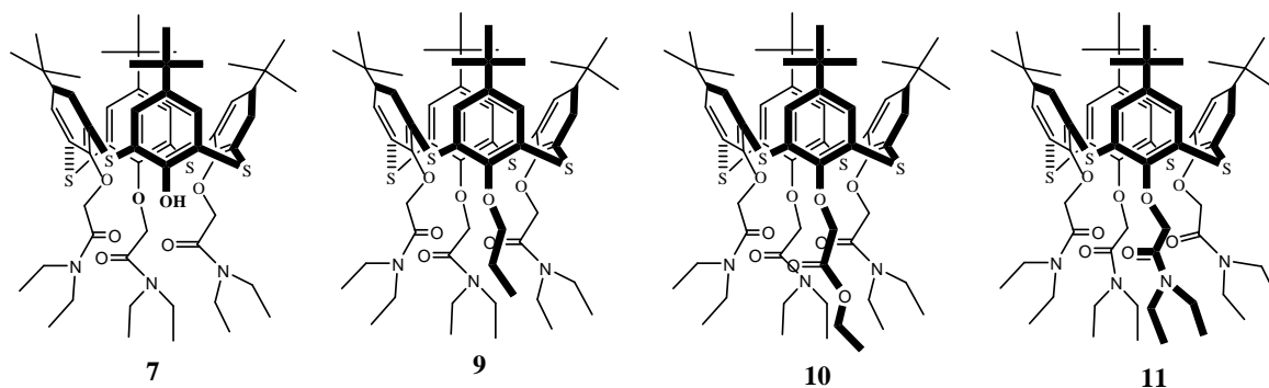
Figure III.10 : Ligands étudiés.
