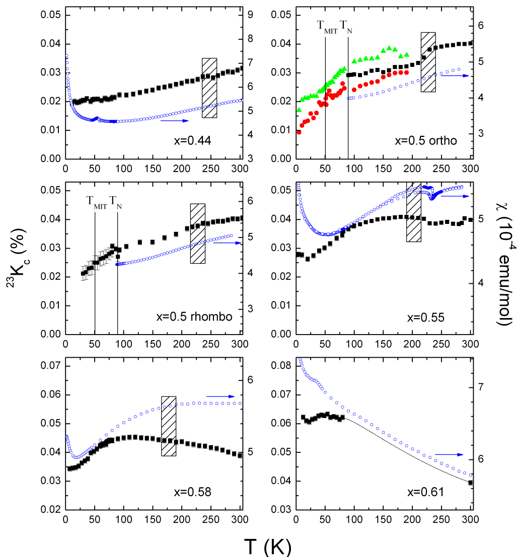
FIG. IV.11 – Dépendance en température du déplacement RMN du sodium, comparée à celle de la susceptibilité macroscopique. Pour x=0.5 orthorhombique, les carrés sont la mesure du centre de gravité de la raie, les ronds et triangles correspondant aux ajustements des sous-sites. Les échelles de déplacement RMN sont identiques à un décalage près. Les rectangles hachurés indiquent les régions d'affinement de la raie centrale par diffusion du sodium.
