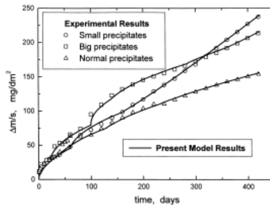
Figure I.29 : Ajustement des courbes cinétiques avec le modèle de Garcia [Gar-99].
