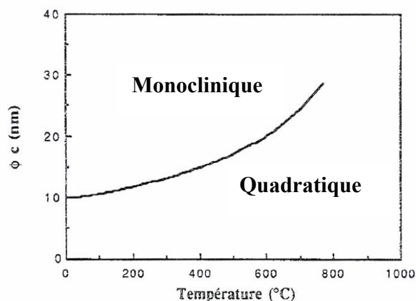
Figure I.19 : Diamètre critique en fonction de la température [Met-92].
