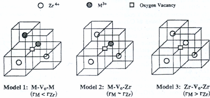
Figure 1.20 : Illustration des trois cas d'insertion cationique en solution solide dans la zirconite [Li-94]
