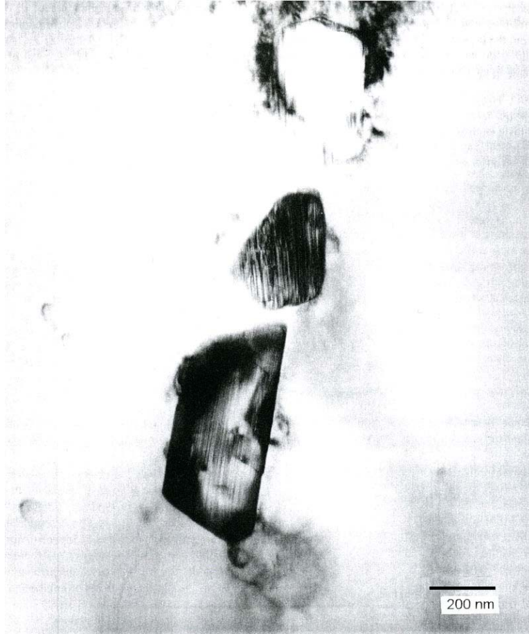
Figure I.13 : Microstructure des précipités Zr(Cr, Fe)_2 , d'après [IAEA-98]
