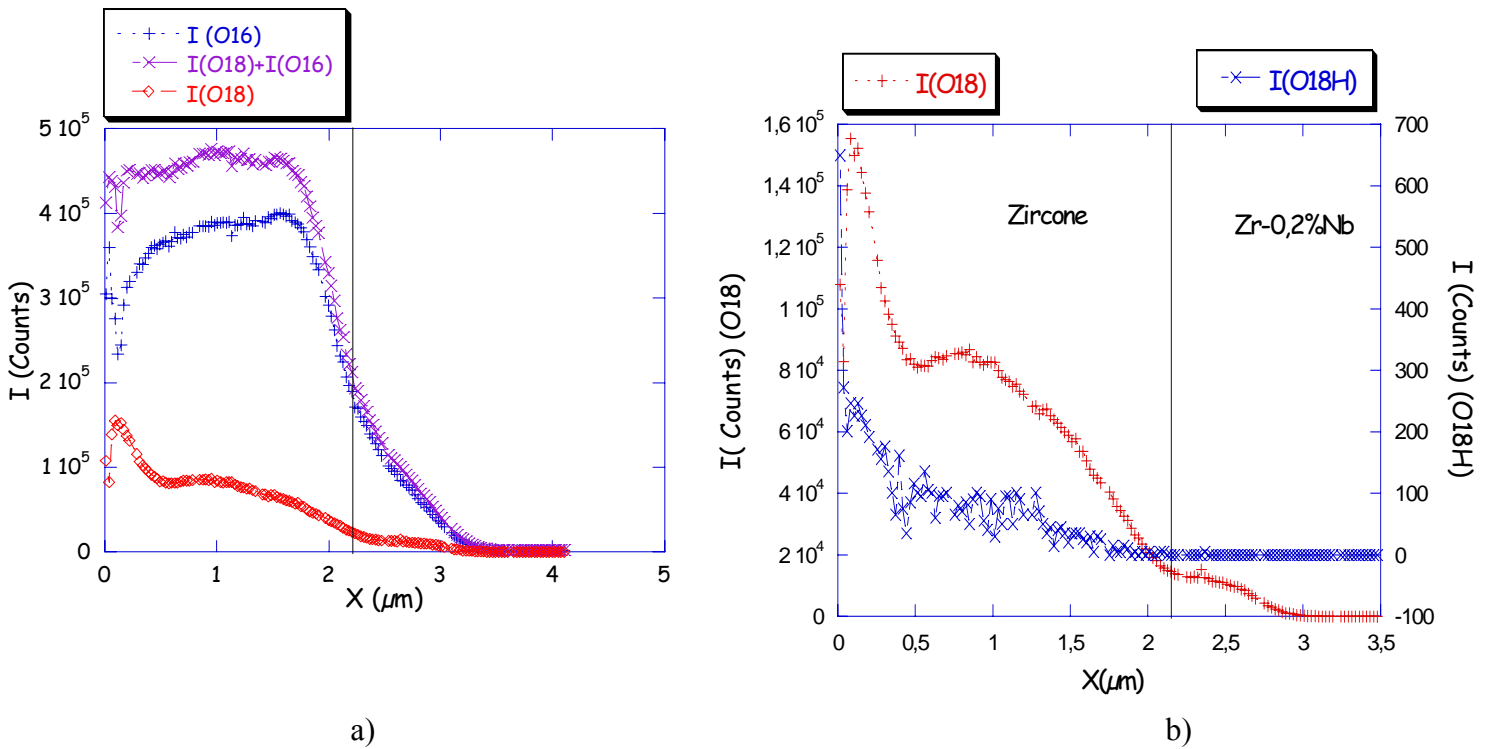
Figure IV.40 : Profils SIMS reconstitués, issus d'espèces présentes dans la couche d'oxyde formée sur Zr-0,2%Nb sous 100 bars de vapeur d'eau à 415°C : a) profil de ^{18}\text{O} , ^{16}\text{O} et ^{18}\text{O} + ^{16}\text{O} après 7 jours d'échange ; b) profil de ^{18}\text{O} , et ^{18}\text{OH} après 7 jours d'échange.
