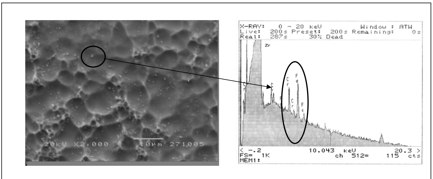
Figure II.2 : Précipités observés par MEB et analyse EDX : a) Zr-0,2%Fe-0,1%Cr, b) Zircaloy-4.
