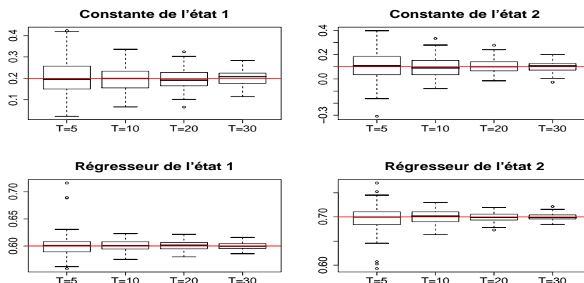
FIG. 3.2 – Boîtes à moustaches des estimations des paramètres des modèles linéaires généralisés pour N=50 individus et T=5, 10, 20 ou 30 temps pour chaque individu sur 100 simulations : cas Poisson - lien log - composantes moins bien séparées. Le trait rouge représente la vraie valeur pour chaque paramètre.
