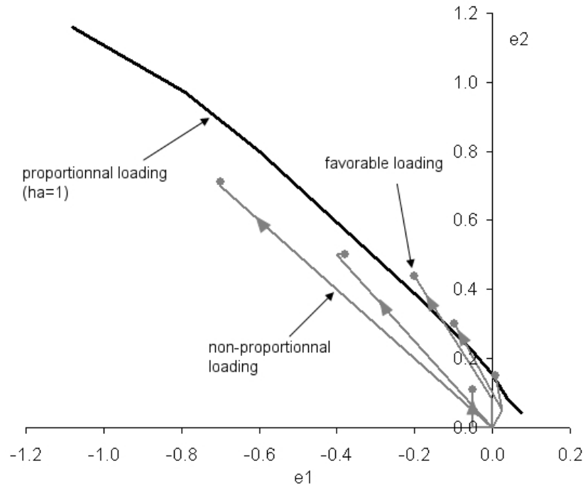
FIG. 4.17: Influence du trajet de chargement : cas sans refermeture des micro-défauts
