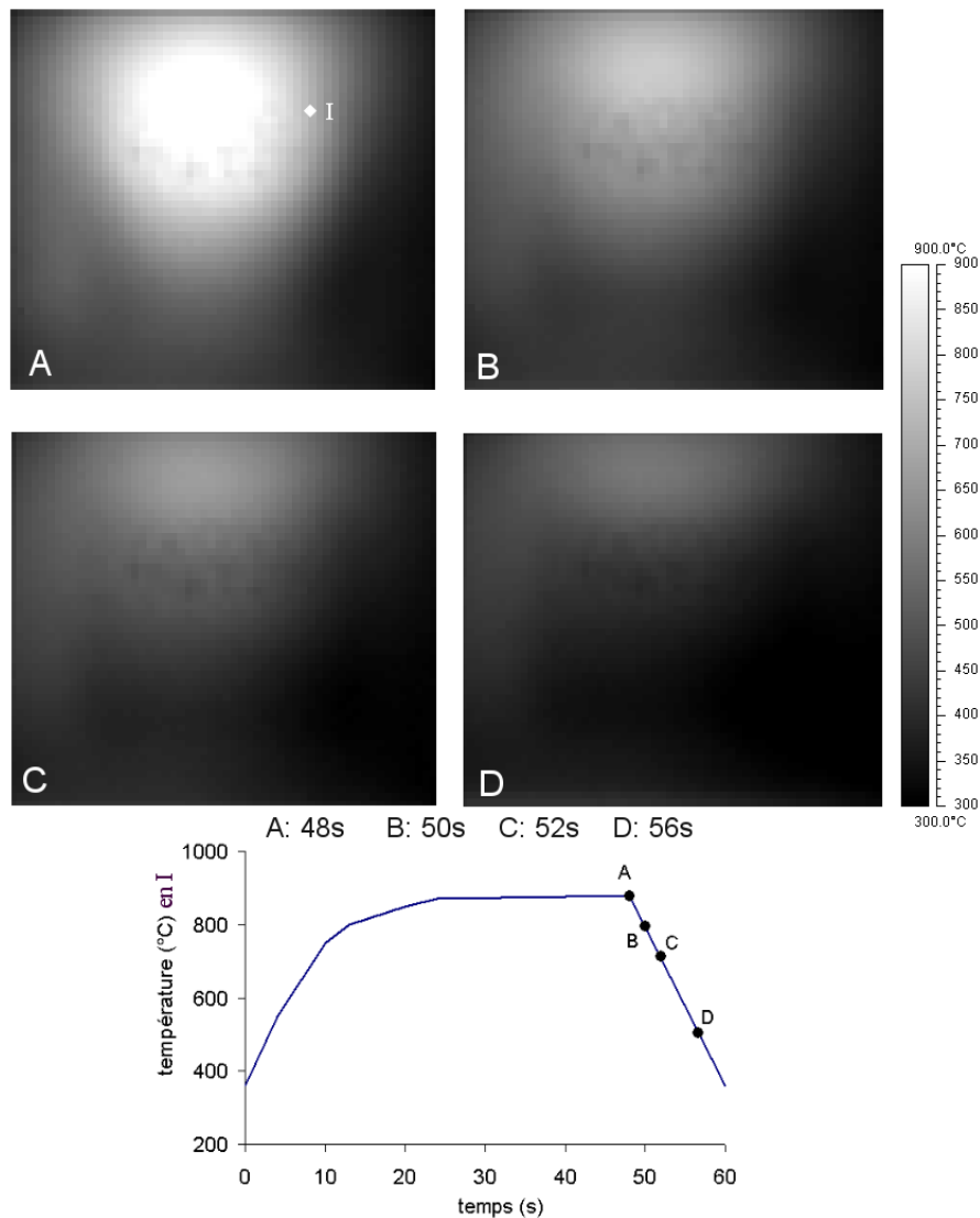
FIG. 5.11: Cartes de températures obtenues lors du refroidissement (chalumeau retiré) en face avant de l'éprouvette
