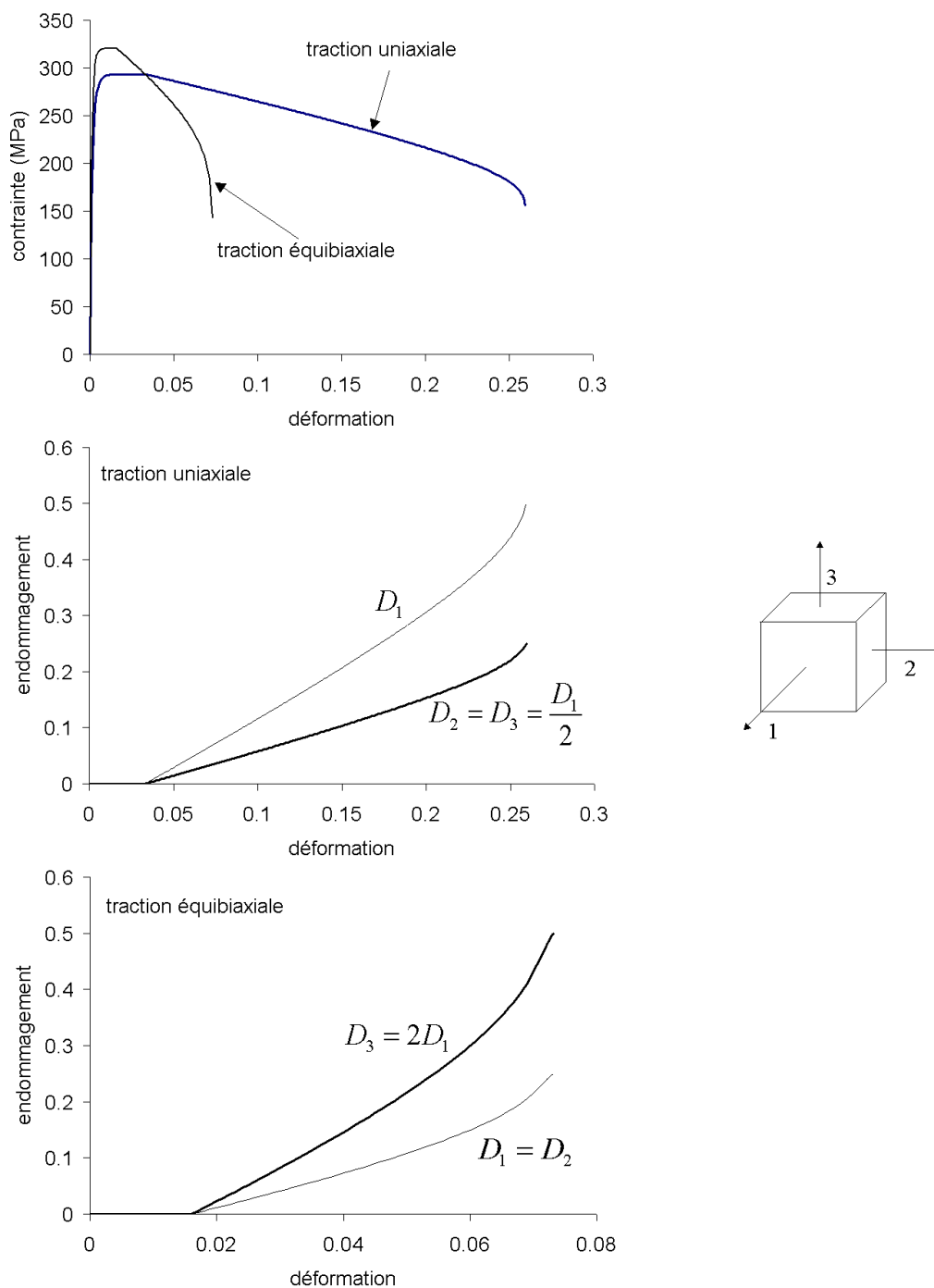
FIG. 4.16: Traction uniaxiale et traction équi-biaxiale, modèle anisotrope du Haynes 188 à 800°C
