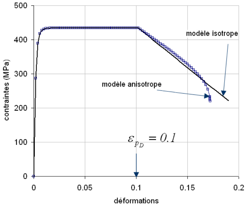
FIG. 1.3: Courbes de traction simulées avec les modèles isotrope et anisotrope d'endommagement (Haynes 188, 800°C, 10^{-4} s^{-1} )
