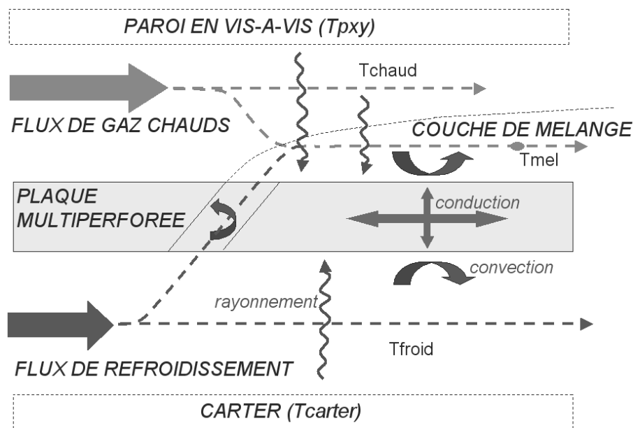
FIG. 5.12: Echanges thermiques dans les chambres de combustion
