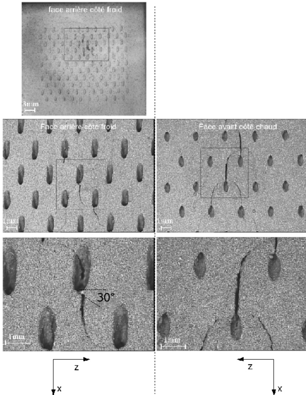
FIG. 5.23: Visualisation à la lunette binoculaire de l'apparition de fissures sur éprouvette expérimentale
