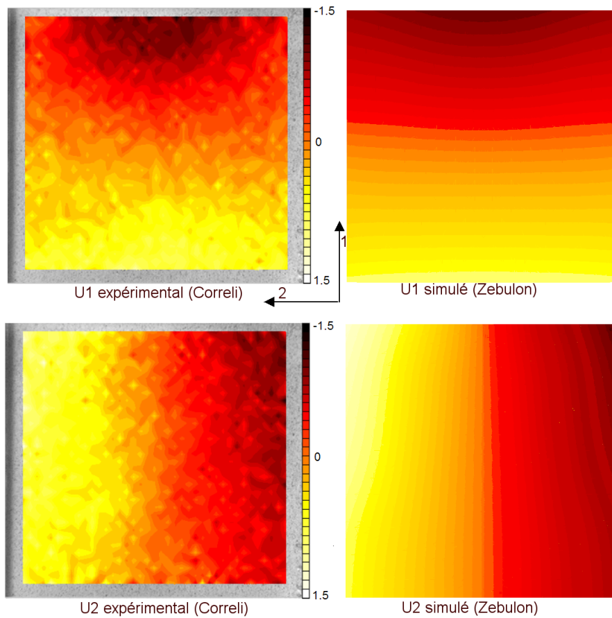
FIG. 5.17: Champs de déplacement expérimentaux et simulés, au point le plus chaud du cycle thermique.
