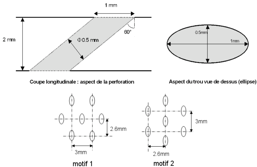
FIG. 5.2: Motifs de perçage pour multi-perforation sur chambre de combustion
