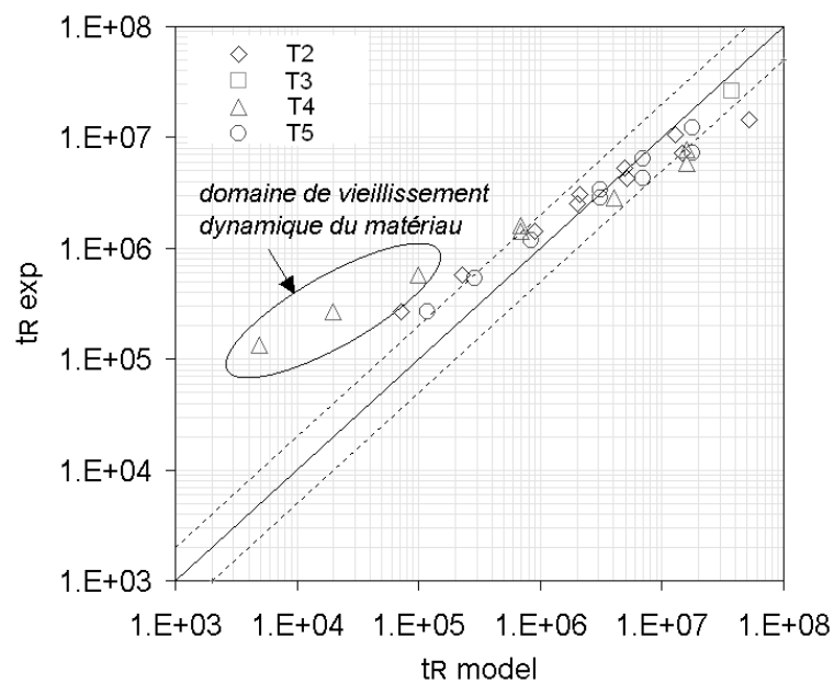
FIG. 3.13: Durée de vie théorique et durée de vie expérimentale en fluage du Haynes 188
