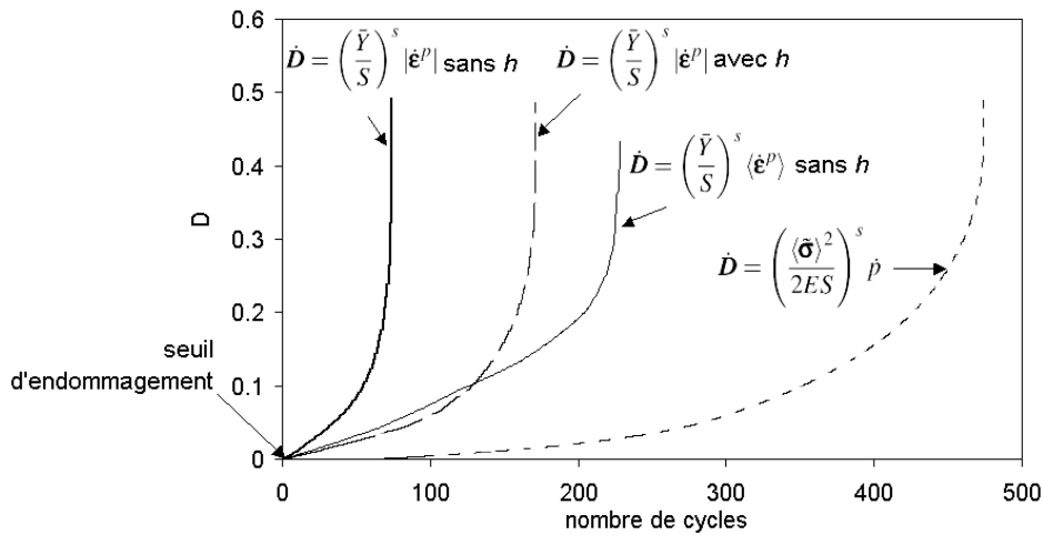
FIG. 4.12: Evolution de l'endommagement selon le modèle incrémental \dot{D} = (\bar{Y}/S)^s |\dot{\epsilon}^p| avec et sans h , lors de la simulation de l'essai thermomécanique.
