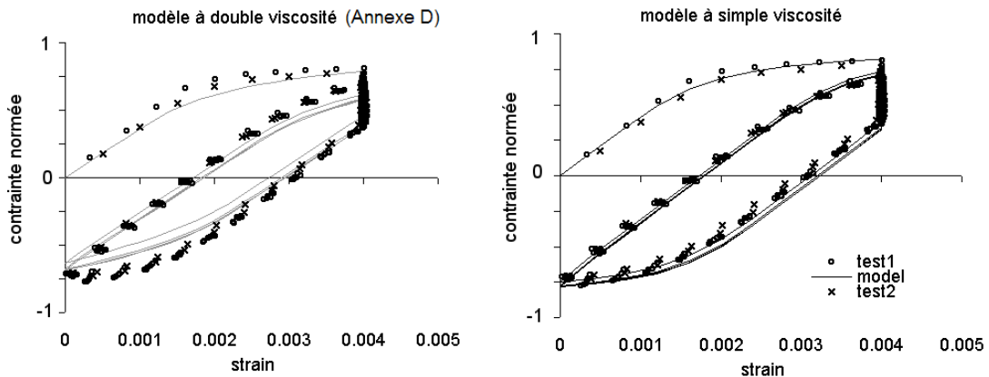
FIG. 3.18: Simulation et résultats expérimentaux du comportement du Haynes 188 à 800°C sous chargement de fatigue à temps de maintien.
