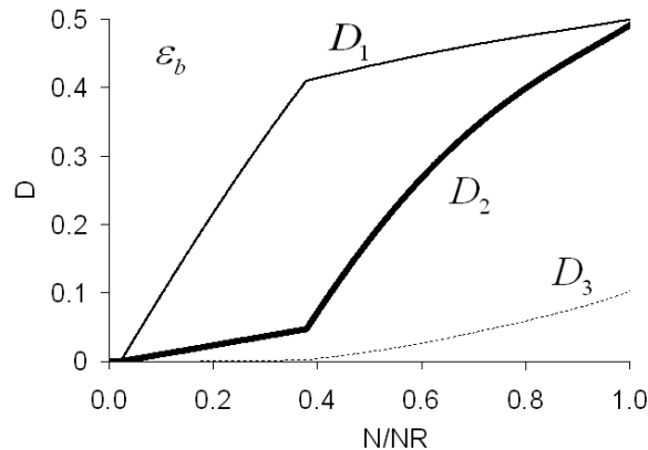
FIG. 4.22: Evolution de l'endommagement en bitraction alternée au point \varepsilon_a de la figure 4.20 pour la loi \dot{D} = (\langle \tilde{\sigma} \rangle^2 / 2ES)^s \dot{p}
