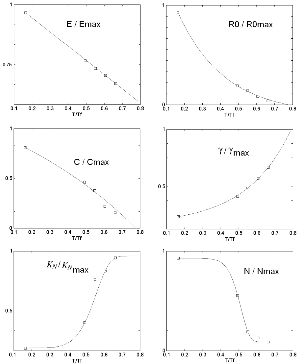
FIG. 3.9: Evolution des paramètres élasto-viscoplastiques en fonction de T/T_f (températures en Kelvin)
