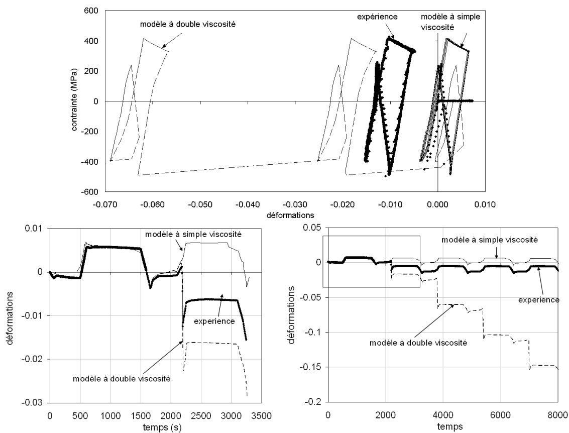
FIG. 4.6: Simulation de l'essai : modèle à simple viscosité et modèle à double viscosité
