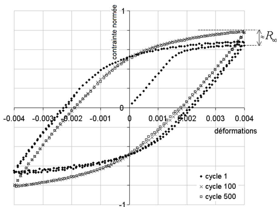
FIG. 3.4: Identification du paramètre R_\infty sur un essai de traction cyclique
