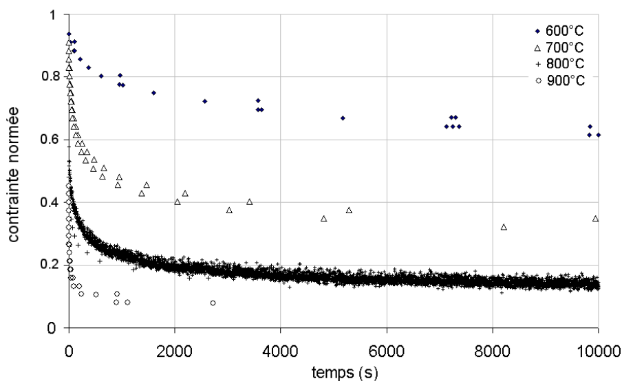
FIG. 3.2: Courbes de relaxation du Haynes 188
