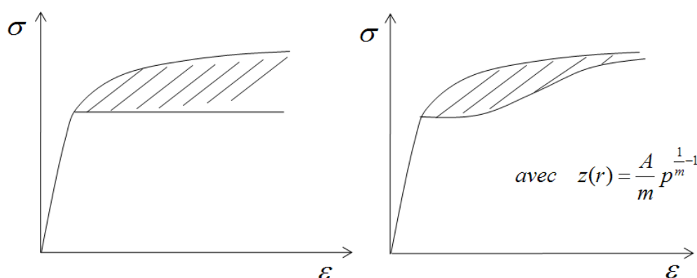
FIG. 1.2: Énergie stockée sur des courbes contrainte-déformation
