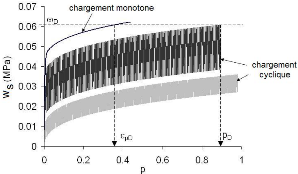
FIG. 1.1: Seuil en énergie stockée et en déformations plastique cumulée pour différents chargements
