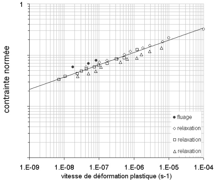
FIG. 3.3: Courbe de viscosité du Haynes 188 à 800°C
