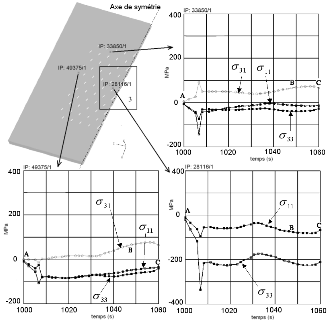
FIG. 5.21: Evolution des contraintes locales en 3 points de la structure multiperforée, lors d'un cycle thermique
