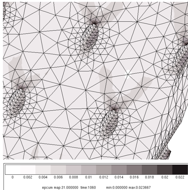
déformation plastique cumulée à l'instant C
