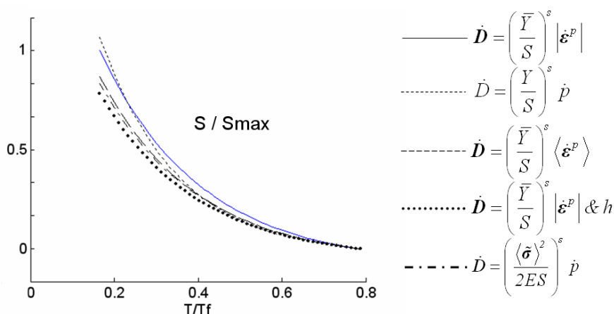
FIG. 3.17: S fonction de T/T_f pour les différentes lois d'endommagement
