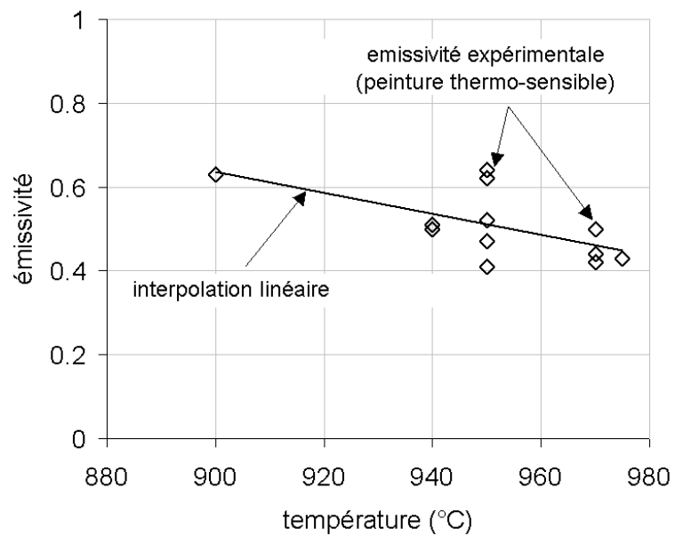
FIG. 5.10: Evolution de l'émissivité de la surface de l'éprouvette en fonction de la température
