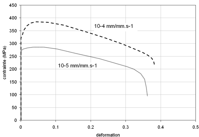
FIG. 4.13: Courbes de traction à rupture, 800°
