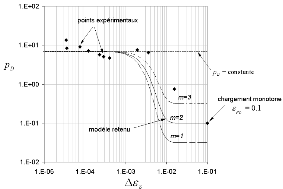
FIG. 3.12: Identification de A et m en fatigue oligocyclique à 800^{\circ}\text{C} , Haynes 188
