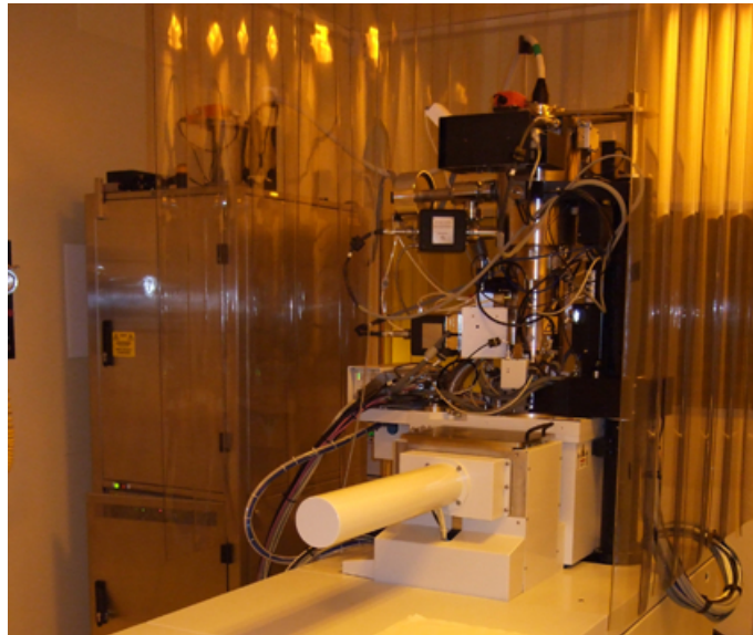
FIG. II.8 – Photographie du nanomasqueur EBPG 5000+ de Vistec lithography Inc.
