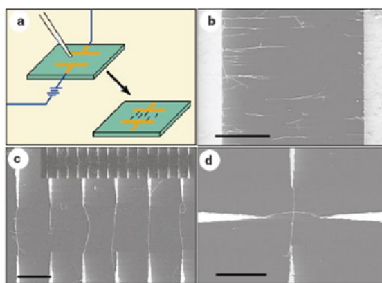
FIG. I.24 – Assemblage par diélectrophorèse [62]
