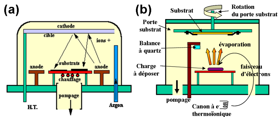
FIG. II.16 – Schémas représentant des bâtis de métallisation (a)Pulvérisation cathodique. [22] (b)Evaporation.
