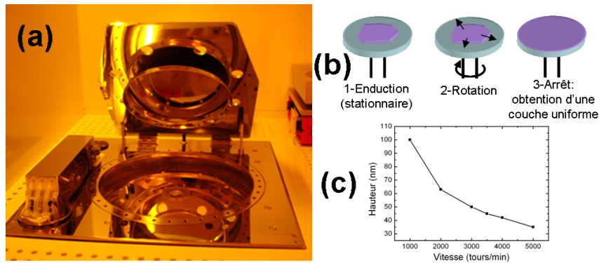
FIG. III.17 – (a) Photographie de la tournette. (b) Étapes de dépôt de résine. (c) Courbe d'étalonnage de l'épaisseur de HSQ (fox-12) en fonction de la vitesse de rotation (Enduction capot fermé, avec une accélération de 1000 tours/min/s pendant 60s).
