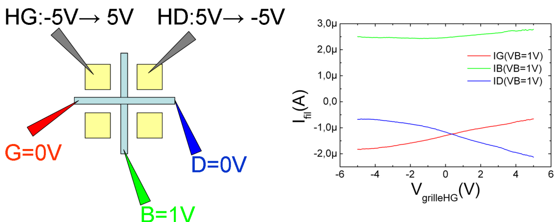
FIG. V.20 – Schéma montrant les tensions appliquées et mesure obtenue sur une croix de 20 nm de large ayant subi un traitement au plasma O_2 .
