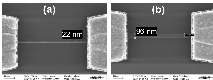
FIG. V.21 – Images MEB des nanofils fabriqués pour la réalisation de capteurs biologiques. (a) Fil de 20 nm de large. (b) Fil de 100 nm de large.
