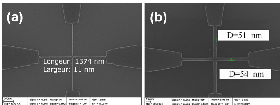
FIG. V.16 – Images MEB montrant des croix de 10 nm de large (a) et 50 nm de large (b).
