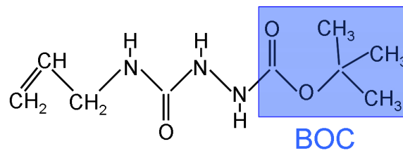
FIG. V.23 – Formule chimique du semicarbazide protégé avec un groupement BOC (ButyloxyCarbonyl).
