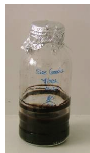
Figure II-8 : Flaçon à plasma de 250 mL recouvert d'une feuille d'aluminium pour représenter une condition en présence d'oxygène ou aérobie.
