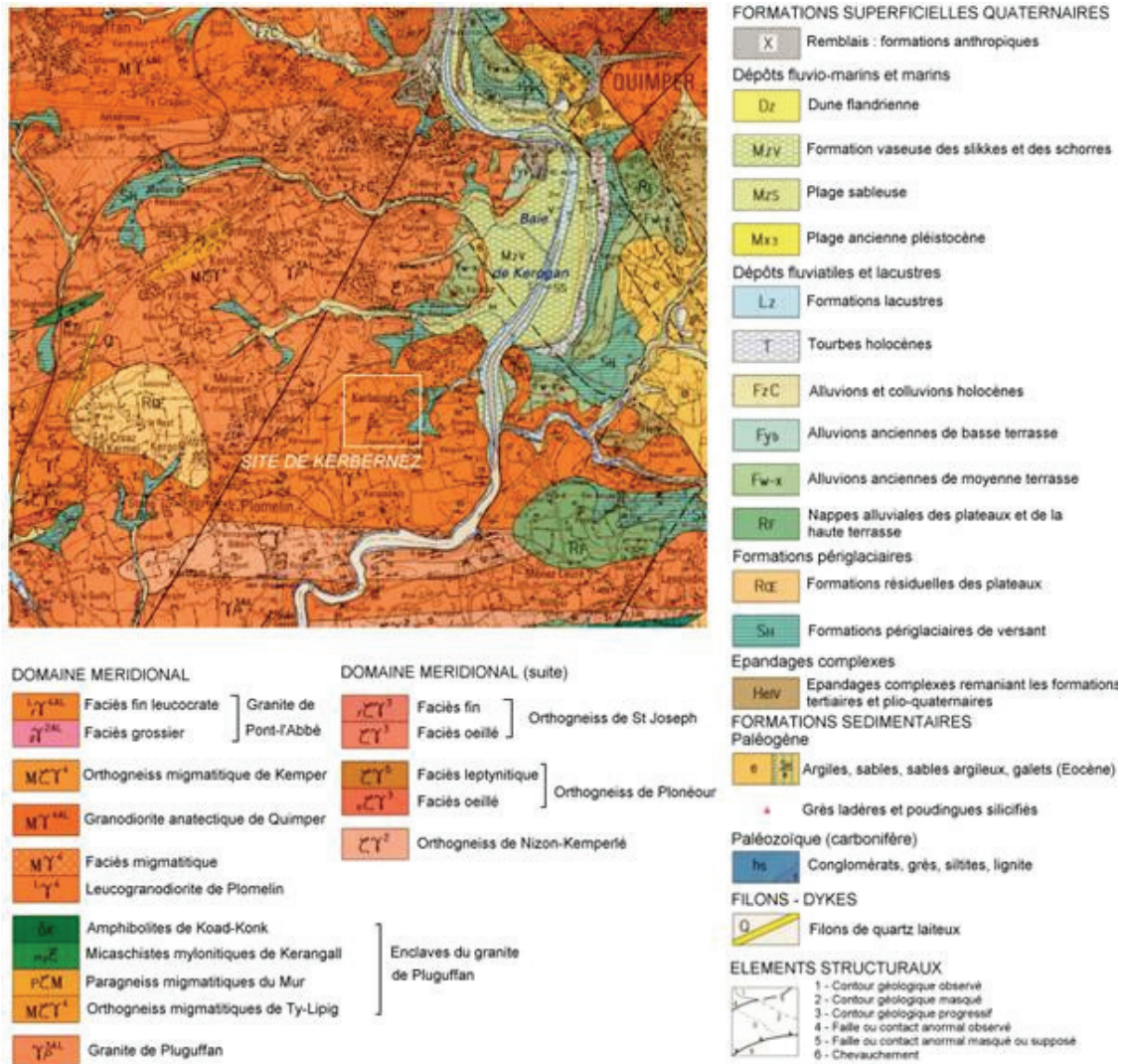
Figure II-6 : Extrait de la carte géologique de Quimper (Feuille 1/50000) incluant la zone d'étude. (Dans Martin, 2003 ; d'après Béhenec et al., 1999)
