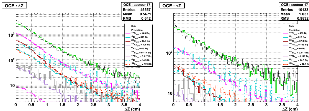
FIG. 4.23 – Distributions des différences de positions longitudinales des vertex reconstruits dans la source pour les électrons traversants le secteur 17. A gauche l'électron traverse la source et à droite il est rétrodiffusé vers l'arrière.
