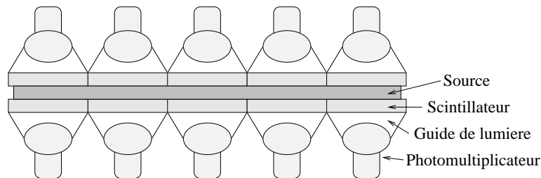
FIG. 6.4 – Schéma de principe du design de BiPo1.
