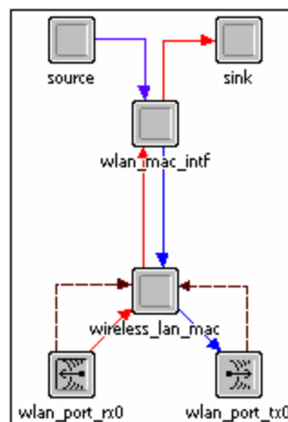
Fig. 4.4 Modèle wlan_station d'OPNET
