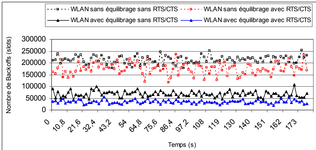
Fig. 4.23 Nombre de slots de Backoff de M14
