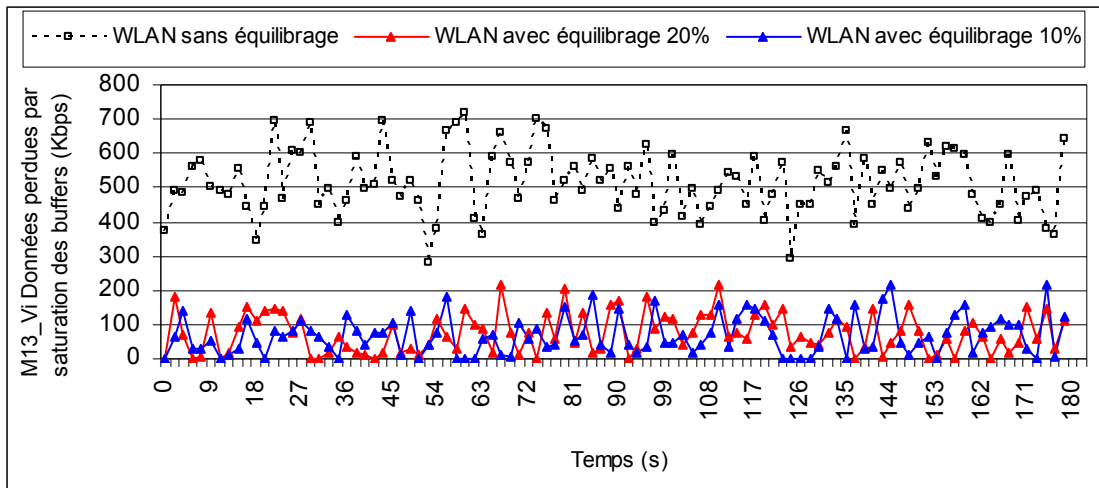
Fig. 4.38 Données perdues par saturation des buffers M13_Vidéo
