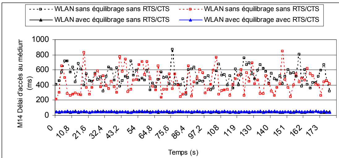
Fig. 4.24 Délai d'accès au médium M14
