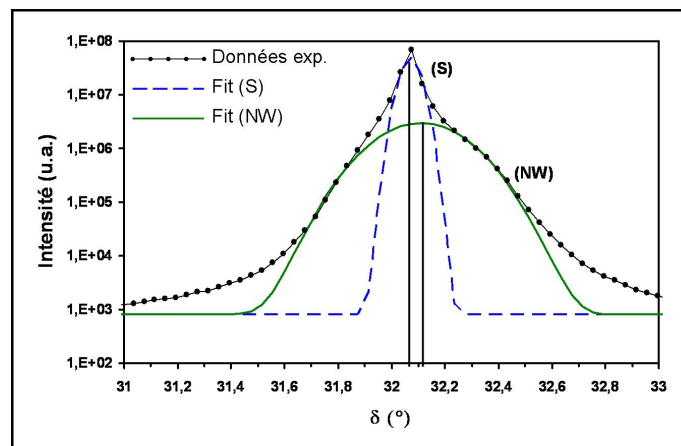
Fig. 4.18: Intensité diffractée autour de la réflexion (2\bar{2}0) du silicium. Le pic (S) correspond au substrat et le pic (NW) aux nanofils. Les fits sont faits uniquement pour déterminer les maxima respectifs des deux pics.
