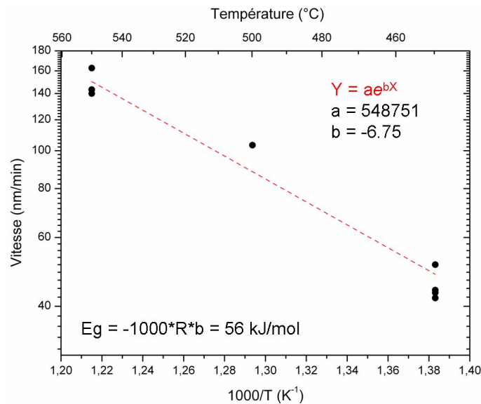
Fig. 4.34: Évolution de la vitesse de croissance des nanofils en fonction de la température, sous 3.7 L/mn de dihydrogène et 25 mL/mn de silane. En déterminant la pente de la droite, on peut déduire une énergie d'activation.
