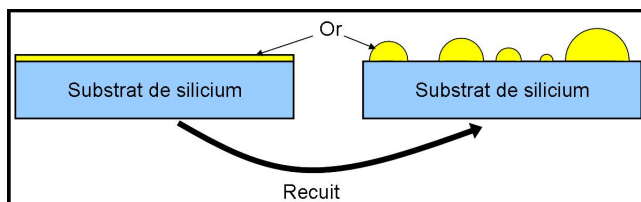
Fig. 3.1: Schéma expliquant le phénomène de démoillage d'une fine couche d'or en gouttelettes lors d'un recuit.
