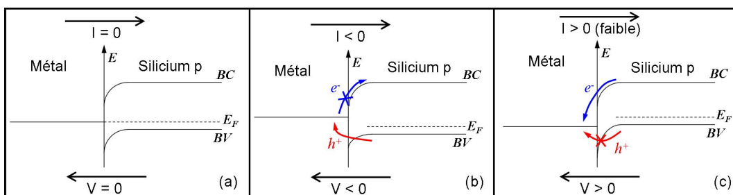
Fig. 4.46: Diagrammes d'énergie d'une jonction Schottky entre un métal et du silicium dopé p. A tension nulle (a) les bandes de valence et de conduction du silicium sont courbées au voisinage de la jonction et on a un réservoir de trous dans le silicium et d'électrons dans le métal. Avec une tension négative (b), les trous peuvent contribuer à faire apparaître un courant négatif non négligeable. Avec une tension positive (c), les trous ne passent plus du silicium vers le métal puisque la barrière qu'ils doivent traverser a augmenté. Seuls quelques électrons minoritaires peuvent passer dans le sens d'un courant positif très faible.
