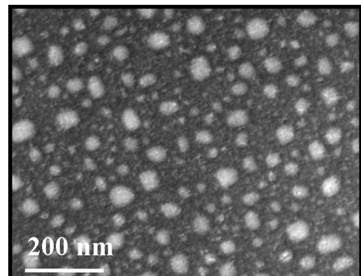
Fig. 3.2: Exemple d'une image MEB de gouttelettes obtenues par démoillage lors d'un recuit d'une fine couche d'or déposée par évaporation sur le substrat de silicium.
