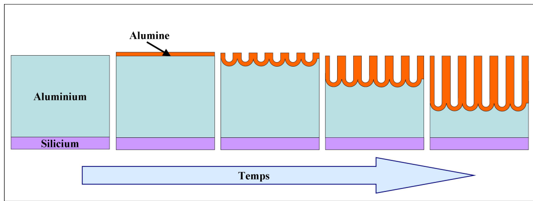
Fig. 2.11: Schéma de la croissance des pores et de la couche d'alumine poreuse lors de l'oxydation anodique de l'aluminium en solution acide.
