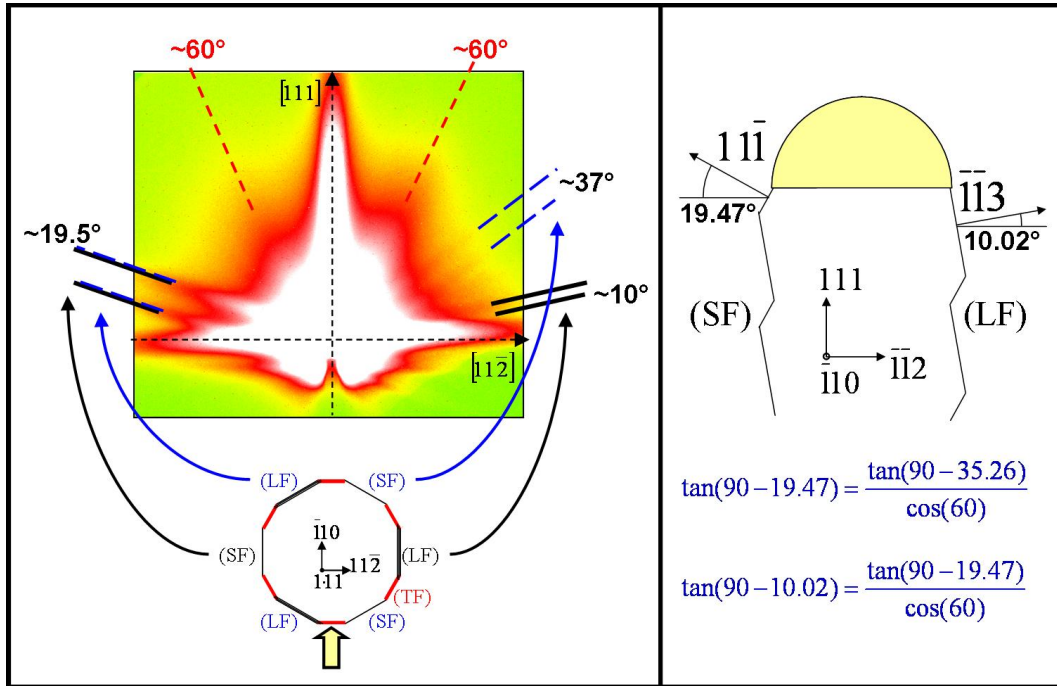
Fig. 4.26: Correspondance entre l'image GISAXS dans la direction [\bar{1}\bar{1}0] et le modèle proposé. Seules les facettes tournées vers le haut sont visibles en GISAXS, le signal des autres se perdant dans le substrat. À gauche, les relations entre les traînées de l'image GISAXS et les faces du modèle présentant les facettes correspondantes. Celles sans correction sont représentées en noir, celles avec correction d'après l'équation 4.5 en bleu, et celles avec une correction inconnue en rouge. Sur la droite de l'image, le modèle en coupe verticale vue dans la direction [\bar{1}\bar{1}0] avec les directions des facettes et les angles calculés.
