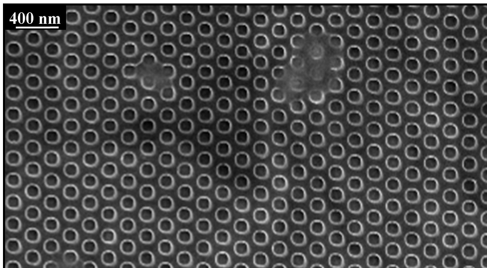
Fig. 2.25: Images MEB d'un échantillon d'aluminium recouvert de résine et ayant été imprimé. Les motifs sont bien visibles et la résine semble n'avoir que quelques défauts locaux probablement dus à des légers problèmes d'adhérence de la résine sur le moule.
