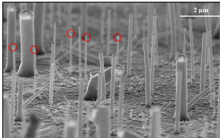
Fig. 4.10: Image MEB inclinée (10°) d'un échantillon après croissance. Les extrémités de fils cerclées de rouge révèlent un arrêt prématuré de la croissance par perte ou encapsulation du catalyseur.
