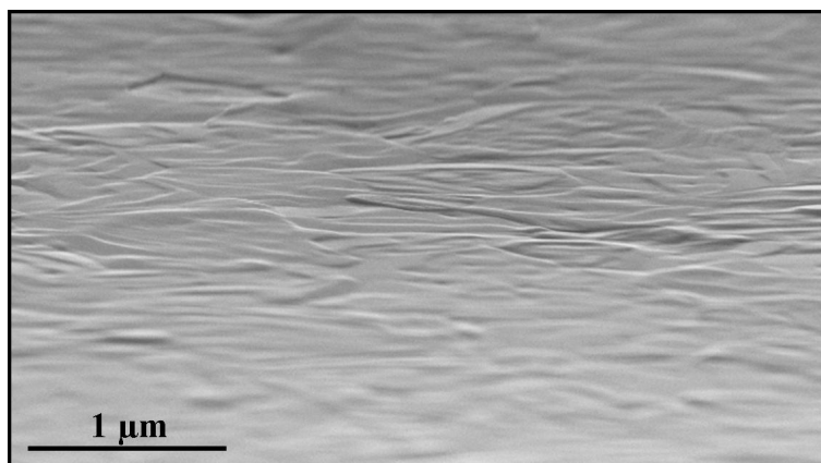
Fig. 2.7: Exemple d'image MEB d'une belle surface d'aluminium déposé par évaporation sur silicium, le substrat étant chauffé in situ à 200 °C pendant le dépôt et sans recuit d'adhérence ensuite.
