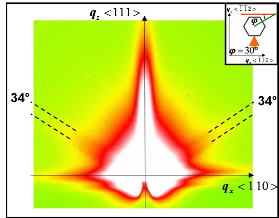
Fig. 4.23: Image GISAXS obtenue avec le faisceau le long de la direction [\bar{1}\bar{1}2] (en insert, une vue de haut de l'orientation d'un fil vis-à-vis du faisceau et du plan de la caméra). Chaque famille de facettes donne une trainée inclinée par rapport à l'horizontale. Les angles mesurés sur l'image \alpha_M de ces trainées sont indiqués. La droite et la gauche de l'image sont bien symétriques.
