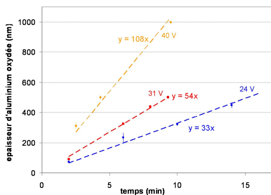
Fig. 2.14: Courbes de l'épaisseur d'aluminium oxydé en fonction du temps pour différentes tensions (acide oxalique, température ambiante).
