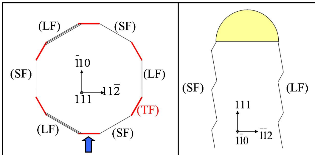
Fig. 4.25: Modèle des nanofils. À gauche, la section des nanofils présente les six faces habituelles, toutes dentelées. La moitié d'entre elles (les faces (LF)) avec les grandes facettes tournées vers le haut, et l'autre moitié (les faces (SF)) avec les petites facettes tournées vers le haut. Les six faces supplémentaires apparaissant en haut des gros nanofils sont représentées en rouge et dentelées (TF) d'un facettage incliné différent. À gauche, une coupe verticale du nanofil vue selon la flèche bleue (direction [\bar{1}\bar{1}0] ). Les deux faces opposées sont de type respectivement (SF) et (LF), expliquant la dissymétrie de l'image GISAXS obtenue sous cette incidence.
