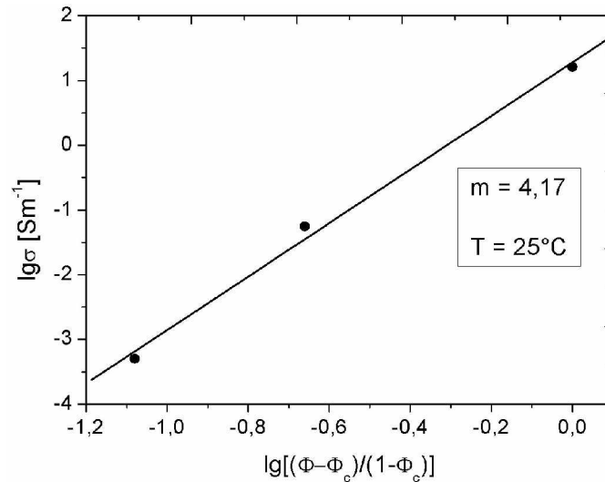
Figure V.19 : Evolution de \lg(\sigma_{\text{eff}} - \sigma_{\text{CeO}_2}) en fonction de \lg\left[\frac{(\Phi_{\text{VRuO}_2} - \Phi_c)}{(1 - \Phi_c)}\right] pour une température 100°C et \Phi_c = 0,04 . Les figures pour toutes les températures sont données dans l'annexe.
