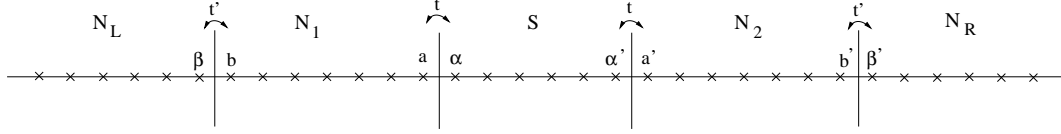
FIG. 1.21 – Jonction N-N-S-N avec le modèle de liaisons fortes.
