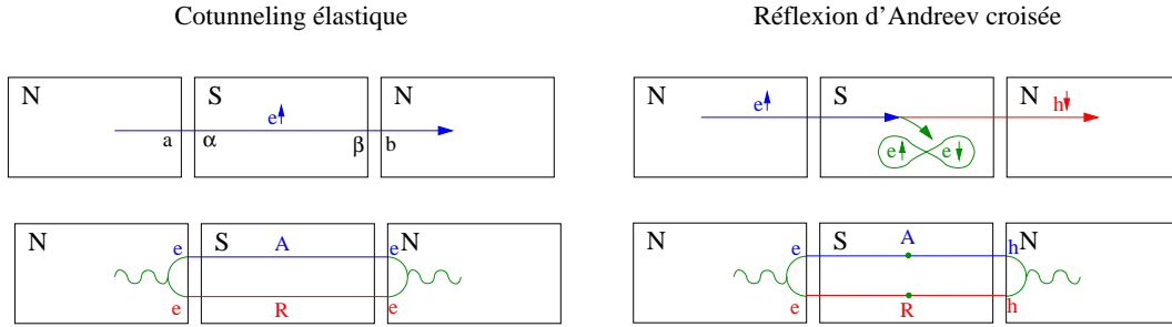
FIG. 1.18 – Processus de cotunneling élastique et de réflexion d'Andreev croisée, en haut. En bas les diagrammes. Les indices des sites sont sur le premier schéma. Les lignes bleues des diagrammes correspondent aux fonctions de Green avancées, les lignes rouges aux fonctions de Green retardées et les lignes ondulées vertes aux densités d'état.
