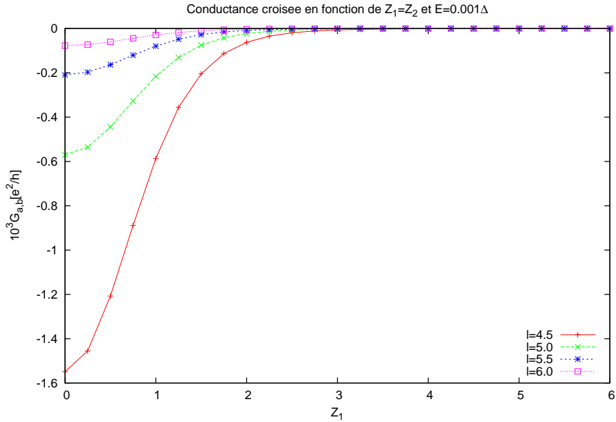
FIG. 1.4 – Conductance non locale, en unité de e^2/h , en fonction de la barrière Z_1 = Z_2 dans le cas où l'énergie, E = 0.001\Delta , est bien au-dessous du gap, en fonction de différentes longueurs du supraconducteur. La longueur du supraconducteur est en unité de \xi , avec \epsilon_F/\Delta = 1000 (où \epsilon_F est l'énergie de Fermi).
