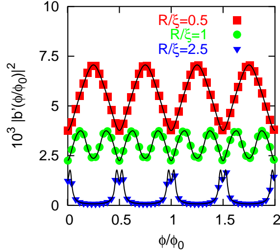
FIG. D.4 – Coefficient de transmission d'un anneau formé d'un isolant à bande interdite avec la relation de dispersion BCS en fonction du flux magnétique \Phi enroulé dans la boucle, normalisé par le quantum de flux \phi_0 = h/e . Les différentes courbes correspondent à différentes valeurs de R/\xi . La valeur de \lambda_F = 2\pi/k_F est petite comparée à \xi .
