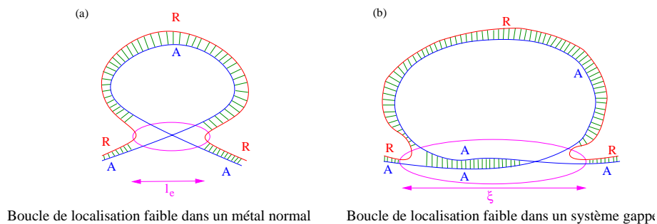
FIG. 4.9 – (a) Croisement d'un diffuseur pour un métal normal. (b) Croisement d'un mode de transmission pour un système avec une bande d'énergie interdite, lorsque l'énergie est inférieure au gap.
