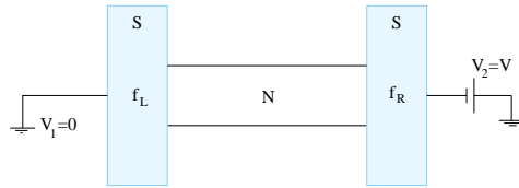
FIG. 3.4 – Jonction S-N-S.
