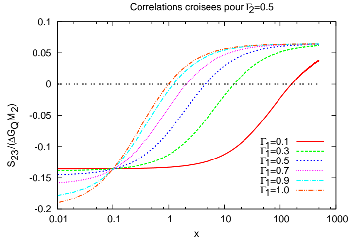
FIG. 3.18 – Corrélations croisées \tilde{S}_{23} renormalisées par M_2 G_Q \Delta en fonction du facteur x = M_1/M_2 . Attention, ici nous normalisons par \Delta au lieu de eV comme dans le cas normal. Les courbes ne se croisent pas toutes au même endroit, cette impression n'est due qu'à l'échelle.
