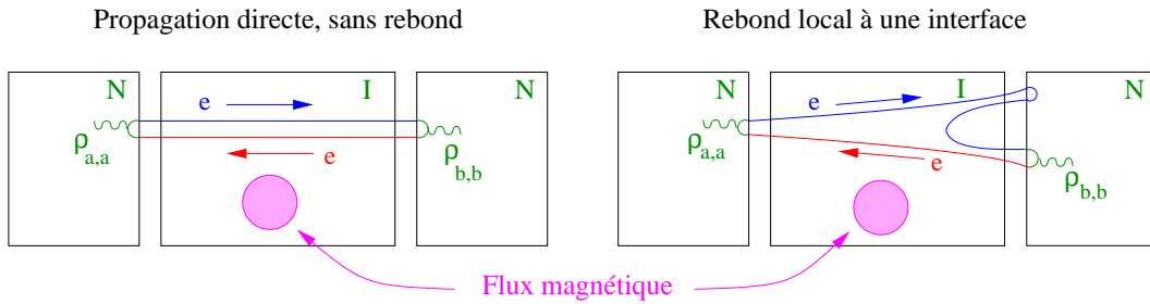
FIG. 1.15 – Processus ne se couplant pas au champ magnétique.
