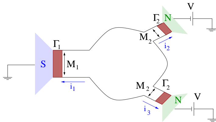
FIG. 3.14 – Schéma de la jonction Y avec un réservoirs supraconducteur pour un système incohérent assimilable à un point quantique.
