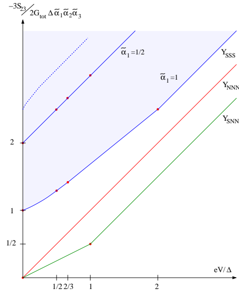
FIG. 3.7 – Schéma de la fonction \frac{-3S_{23}}{2G_{tot}\tilde{\alpha}_1\tilde{\alpha}_2\tilde{\alpha}_3} en fonction de eV/\Delta . La surface bleue correspond à la zone possible pour les corrélations croisées de la jonction avec trois réservoirs supraconducteurs pour différentes valeurs de \tilde{\alpha}_1 .
