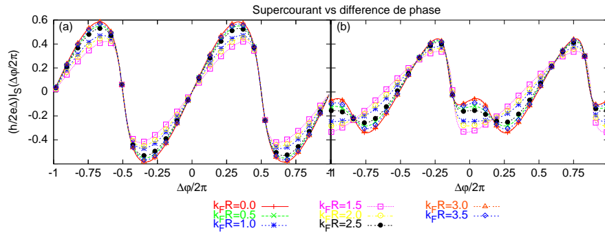
FIG. 2.10 – Supercourant en fonction de la différence de phase \Delta\varphi , avec des processus non locaux \mathcal{C}_0 = 1 , pour différentes valeurs de k_F R_{\alpha\beta} , et pour T_\alpha = T_\beta = 0.8 , (a) sans champ magnétique \phi = 0 et (b) avec un flux magnétique \phi = 2 .
