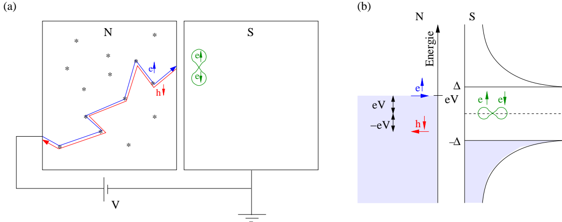
FIG. 1 – Schéma du processus de réflexion d'Andreev à une interface N-S, où un électron est injecté dans une électrode normale. On a création d'une paire de Cooper qui part dans le condensat du supraconducteur et rétrodiffusion d'un trou (charge et spin opposés à ceux de l'électron) dans l'électrode normale (a). Schéma en énergie pour la réflexion d'Andreev (b). e\uparrow représente un électron de spin up et h\downarrow un trou dans la bande de spin down.
