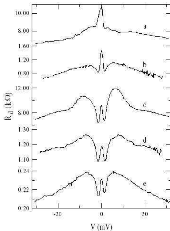
FIG. 4.3 – Résistance différentielle ( R_d(V) ) en fonction de la tension appliquée pour un point de contact supraconducteur (Nb) - ondes de densité de charge ( NbSe_3 ) de différentes sortes mesurées à T = 3.6K . Les courbes (a) et (b) sont pour des jonctions avec une barrière tunnel isolante à l'interface S-ODC. Les courbes (c)-(e) sont pour des points de contacts avec une conductivité directe (sans barrière isolante) [71].
