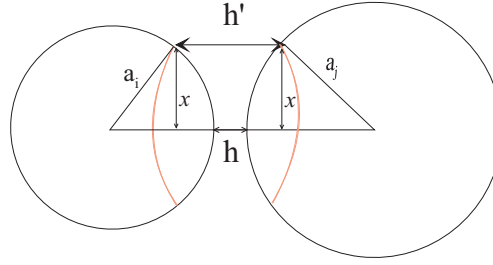
Fig. 1.6. Principe d'intégration suivant l'approximation de Derjaguin.
