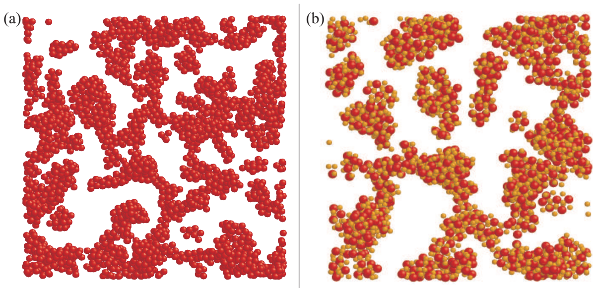
Fig. 4.19. Image à t = 5 s des simulations de dynamique Brownienne : (a) pour des particules d'alumine non chargées et (b) pour le système mixte à R = 22\% .
