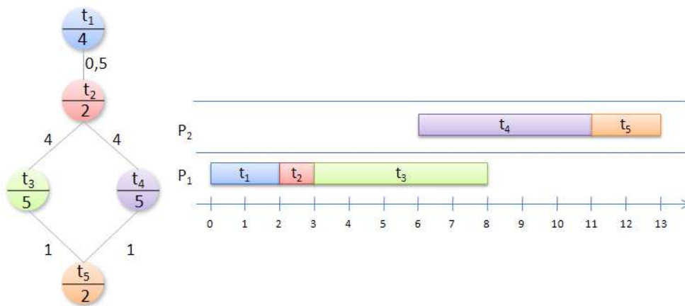
Figure 5.6 – Exemple d'ordonnement d'un graphe de tâches sur 2 processeurs.
