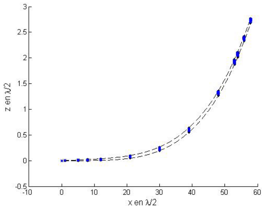
FIG. 5.3: Estimés à la fin de l'algorithme d'autocalibration de l'antenne 4 avec N_s = 12000 , RSB= 20dB.
