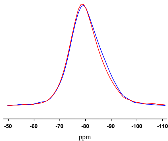
Figure 12.8. Spectres RMN ^{29}\text{Si} du 46S6 et du 46S6 Sup
