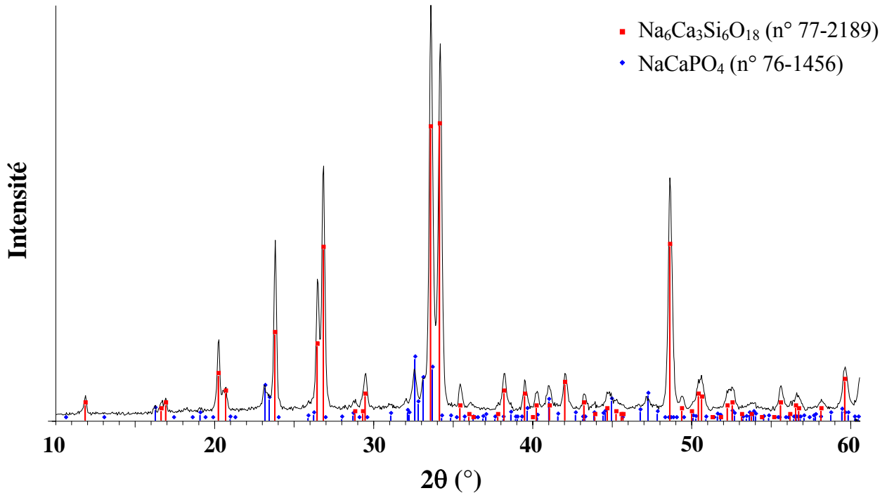
Figure 17.7. Diffractogramme de l'échantillon 1110^{\circ}\text{C} - 5 min
