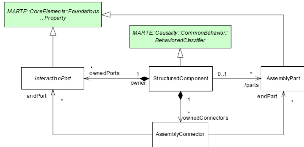
Figure 3.9. Méta-modèle de description structurelle des composants en MARTE [MARTE2007].
