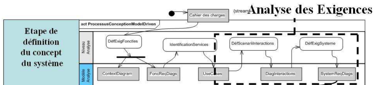
Figure 9.5. Le processus d'analyse des exigences appliqué à SysML étendu.
