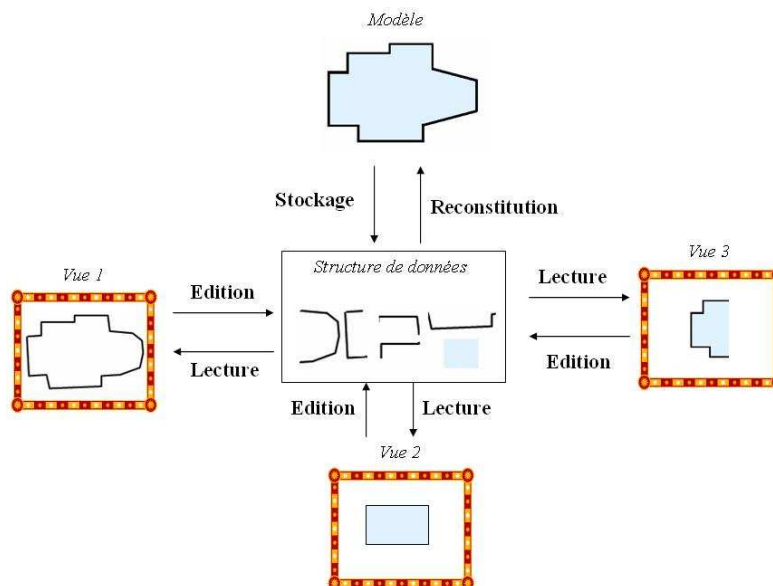
Figure 1.2. Un modèle peut être vu sous plusieurs angles.
