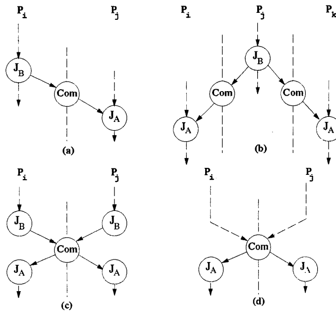
FIG. 5.1 - Différents graphes de dépendance.
