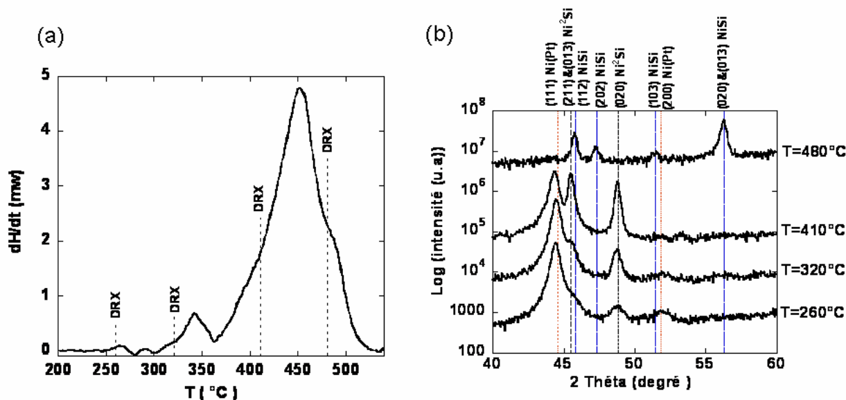
Figure 30 : (a) Thermogramme de DSC pour une rampe de 75 K/min avec les températures d'arrêt des recuits réalisés sur 80 nm de \text{Ni(5\%Pt)/Si} et (b) Diagrammes de DRX après chaque arrêt ( \lambda = 1.54 \text{ \AA} ).
