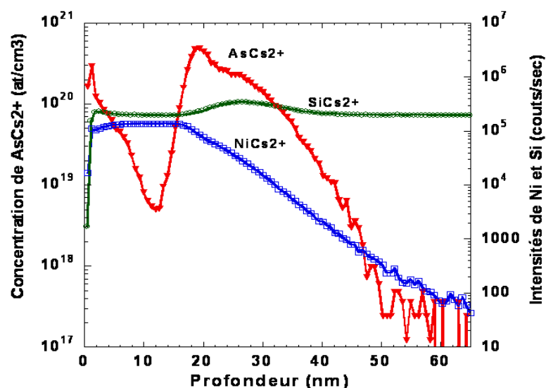
Figure 19 : Profils SIMS, en profondeur, de la concentration de l'arsenic \text{AsCs}_2^+ , les intensités de nickel, le silicium et le césium après dépôt de 8nm de nickel et siliciuration à 400°C par RTP. Le substrat de silicium est implanté avec une énergie de 7keV et une dose de 1^{15} \text{ at/cm}^2 .
