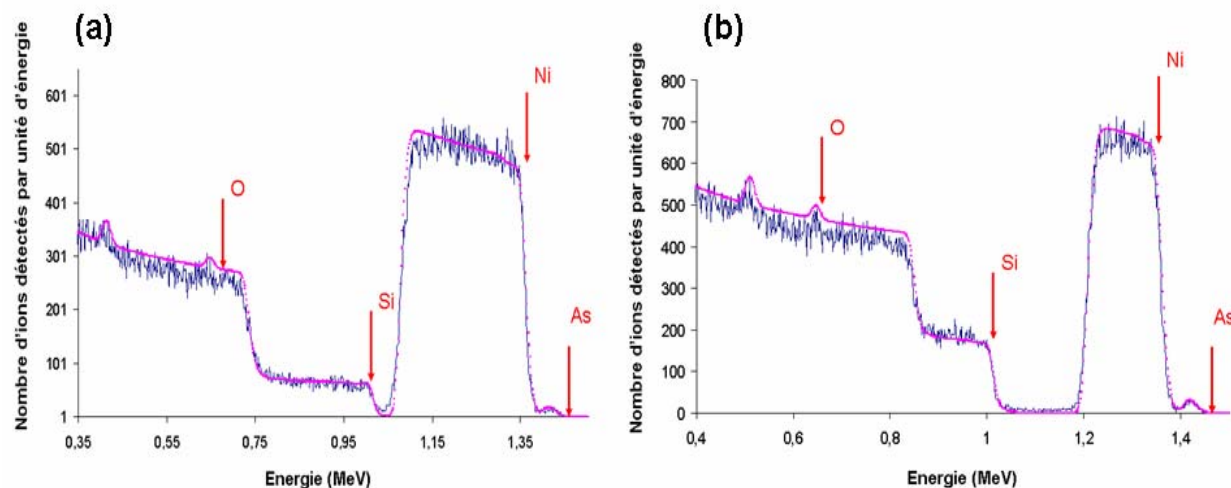
Figure 57 : Spectres RBS des échantillons de \text{Ni}_2\text{Si} (a) et \text{NiSi} (b) (Données expérimentales et simulation).
