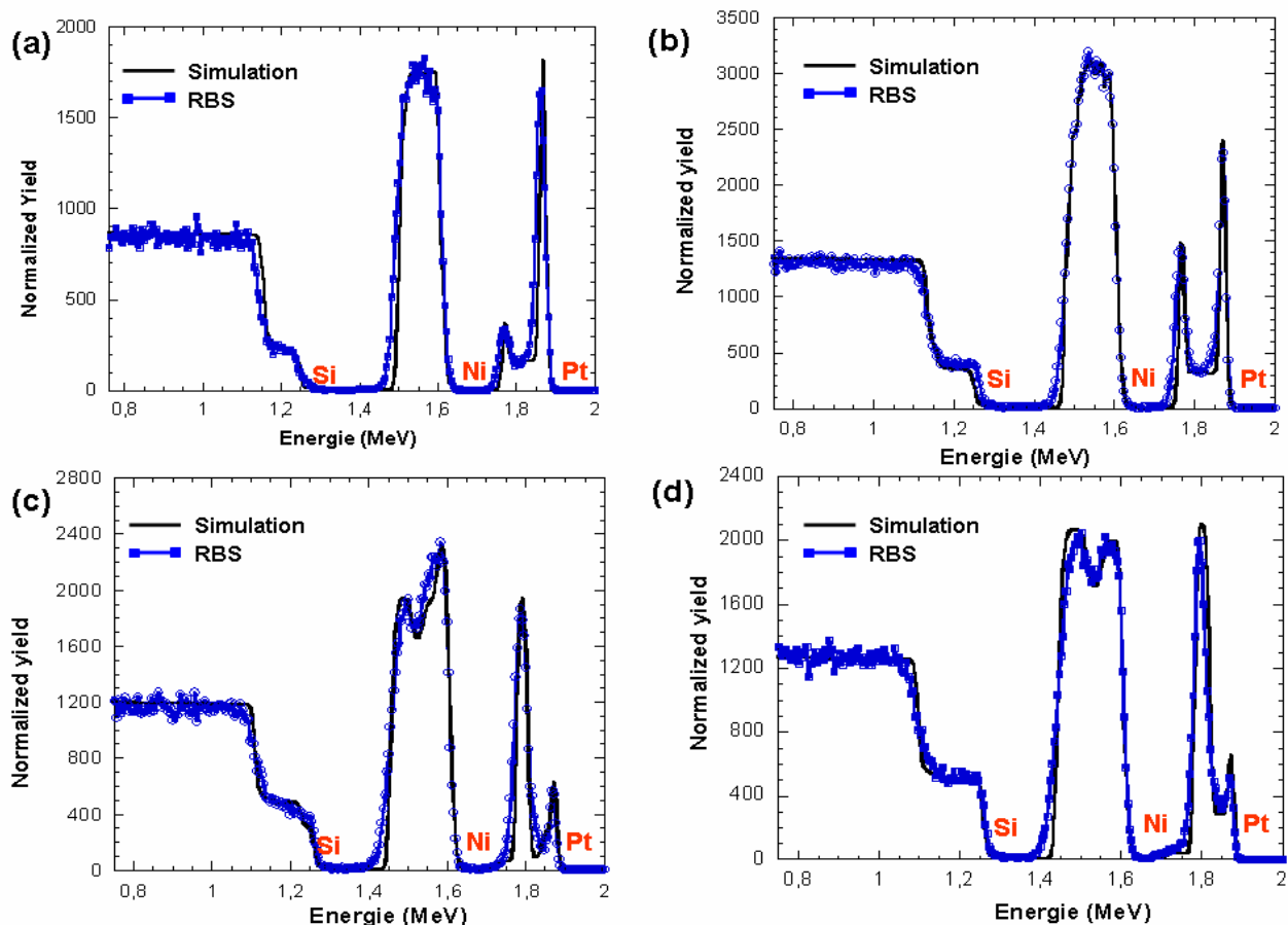
Figure 32 : Spectres RBS de Ni(5%Pt)/Si(100) après différents recuits correspondant à différentes étapes de siliciuration : (a) recuit à 230°C pendant 8 h, formation simultanée de \text{Ni}_2\text{Si} et NiSi en présence de nickel allié, (b) recuit à 230°C pendant 12 h, formation simultanée de \text{Ni}_2\text{Si} et NiSi en présence de nickel allié, (c) recuit à 245°C pendant 10 h, présence de \text{Ni}_2\text{Si} et NiSi et (d) recuit à 270°C pendant 14 h, présence de NiSi uniquement.
