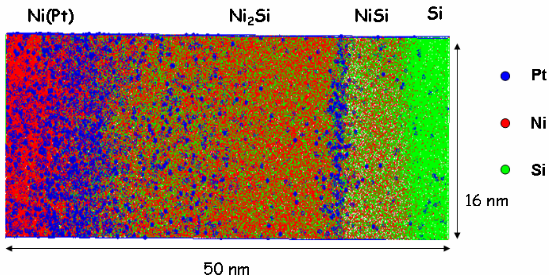
Figure 16 : Volume reconstruit ( 15 \times 15 \times 52 \text{ nm}^3 ) des atomes de Ni, de Si et de Pt obtenu par sonde atomique tomographique à grand angle assistée par un laser femtoseconde. Ce volume est extrait d'un échantillon de Ni(5%Pt)/Si recuit à 290^\circ\text{C} pendant 1h.
