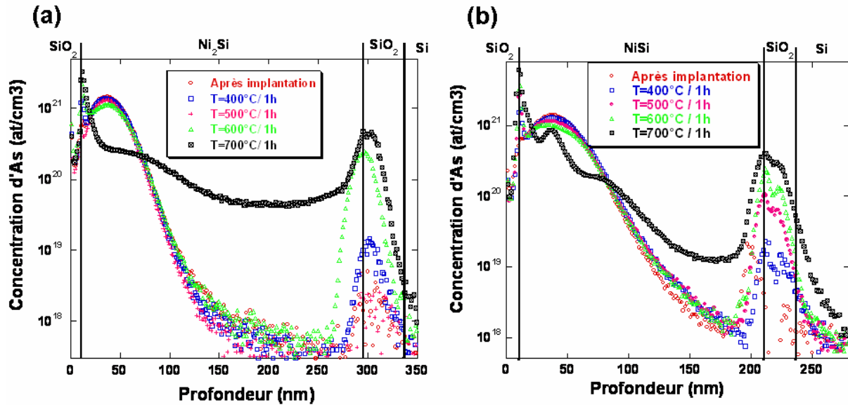
Figure 20 : Profils SIMS de la concentration d'arsenic après implantation et après recuit à 400, 500, 600 et 700°C pendant 1 heure. (a) la phase \text{Ni}_2\text{Si} dans la structure suivante \text{SiO}_2/\text{Ni}_2\text{Si}/\text{SiO}_2/\text{Si} et (b) la phase \text{NiSi} dans la structure suivante \text{SiO}_2/\text{NiSi}/\text{SiO}_2/\text{Si} . Les conditions d'implantation de l'arsenic sont : (a)
