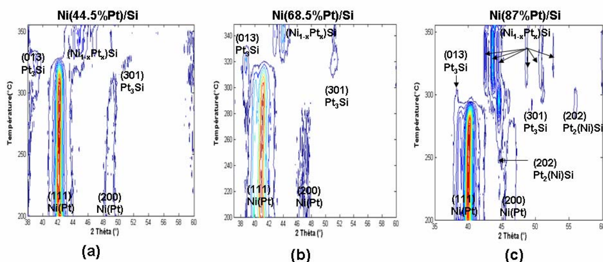
Figure 45 : Diagrammes de DRX in situ lors d'un recuit par paliers isothermes tous les 10°C entre 200°C et 350°C (avec \lambda=1.54\text{\AA} ) sur 50 nm de (a) \text{Ni}(44.5\%\text{Pt})/\text{Si}(100) , (b) \text{Ni}(68.5\%\text{Pt})/\text{Si}(100) et (c) \text{Ni}(87\%\text{Pt})/\text{Si}(100) .
