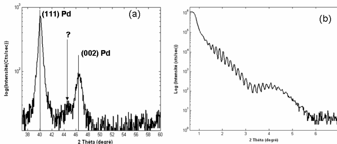
Figure 11 : Caractérisation de l'échantillon Pd/Si(100) après dépôt par pulvérisation cathodique, (a) diagramme de DRX et (b) spectre de RRR ( \lambda=1.54\text{\AA} ).
