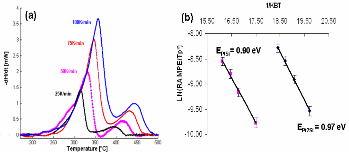
Figure 21 : (a) Thermogrammes de DSC obtenus par recuit à 25, 50, 75 et 100 K/min lors de la réaction d'un film de 50 nm de Pt/Si(100) et (b) Représentation de Kissinger (analyse permettant de déterminer l'énergie d'activation à partir des températures maximales des pics pour chaque rampe pour les différents pics de DSC).
