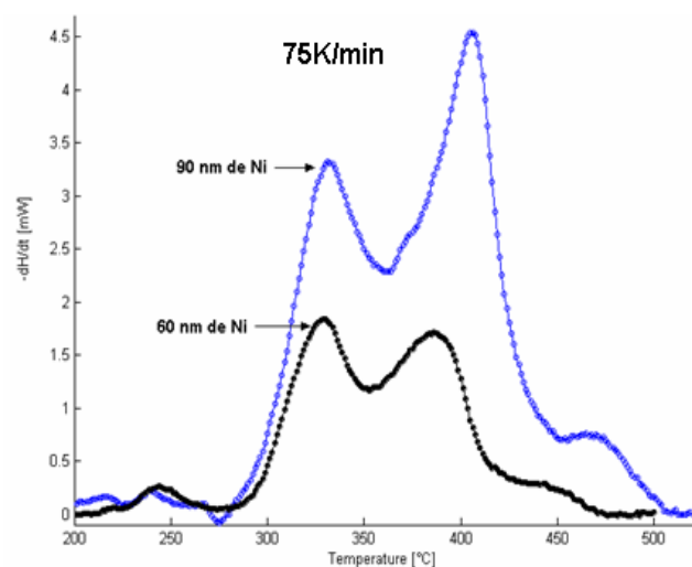
Figure 9 : Thermogrammes de DSC obtenus par recuit à 75 K/min lors de la réaction d'un film de 60 nm et de 90 nm de Ni avec un substrat de silicium (100) de 100 \mu\text{m} d'épaisseur.
