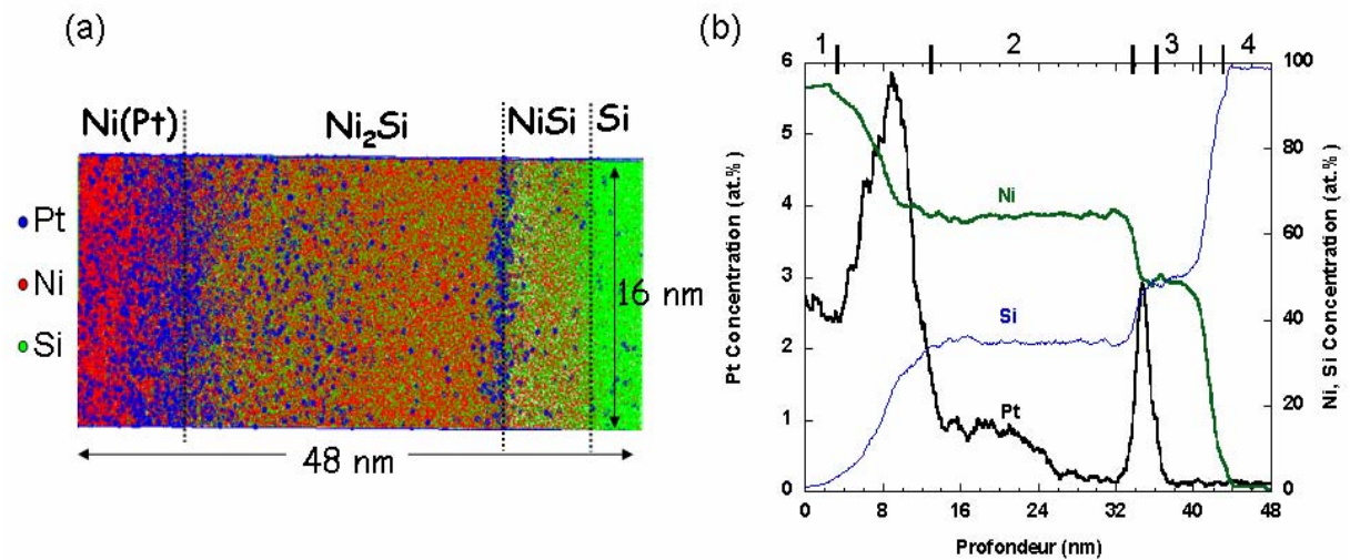
Figure 42 : (a) Reconstruction en 3D par SAT à grand angle assistée par un laser femtoseconde, de 80 nm \text{Ni}(5\%\text{Pt}) déposé sur des plots de silicium (100) après recuit à 290^\circ\text{C} pendant 1h (b) Profils de concentration du nickel, du silicium et du platine à travers les différentes phases présentes. Les concentrations locales sont calculées pour de petites boîtes (de 0.1 nm d'épaisseur et 15 nm de largeur d'une zone perpendiculaire aux interfaces).
