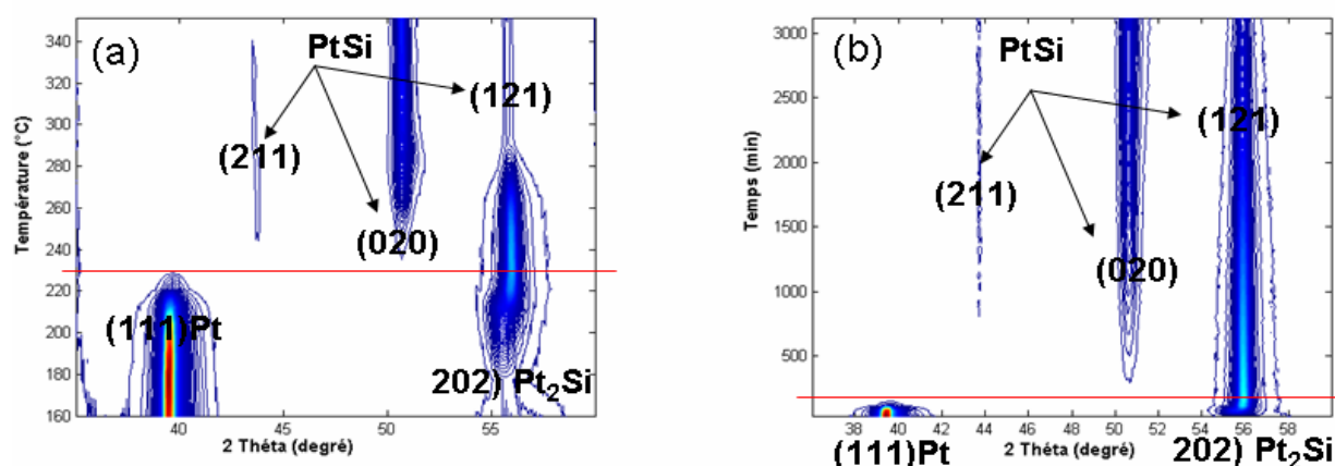
Figure 16 : Diagrammes de DRX in situ en géométrie Bragg-Brentano réalisés sur 60 nm de Pt/Si(100) (a) lors d'un recuit par paliers isothermes tous les 10^\circ\text{C} entre 160 et 350^\circ\text{C} , (b) lors d'un recuit isotherme à 210^\circ\text{C} avec \lambda=1.54\text{\AA} .
