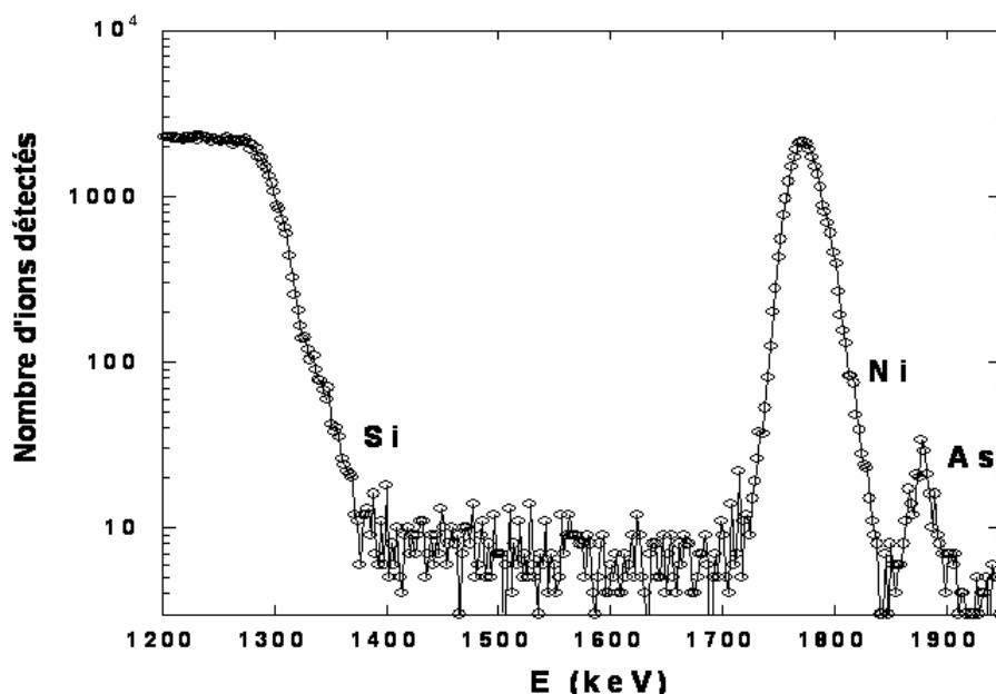
Figure 56 : Spectre RBS en échelle logarithmique obtenu sur un échantillon de 8 nm de Ni/Si(100) dopé en arsenic, après recuit par RTP à 400^\circ\text{C} (avec un flux d'ions \text{He}^+ d'énergie égale à 2.3 MeV).
