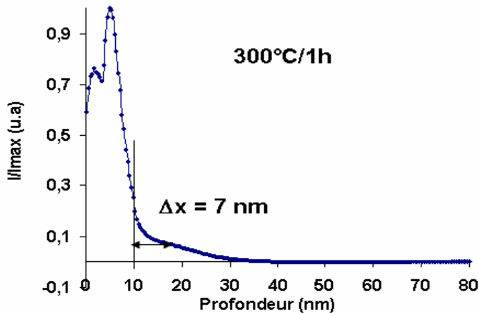
Figure 14 : Profil SIMS du platine dans la phase \text{Ni}_2\text{Si} après dépôt de 10 nm de platine et recuit sous vide à 300^\circ\text{C} pendant 1h.
