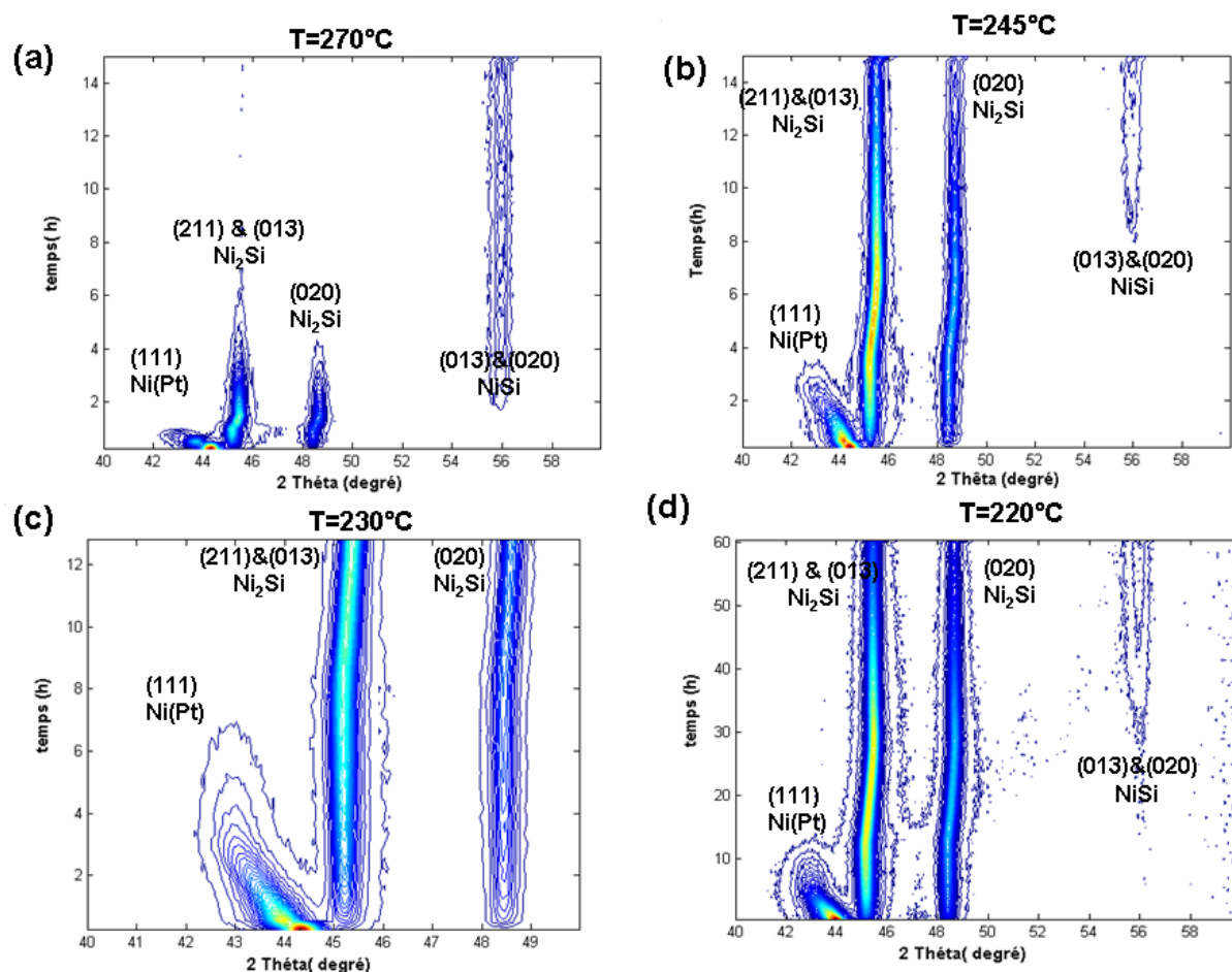
Figure 23 : Diagrammes de DRX in situ en géométrie Bragg-Brentano ( \lambda=1.54\text{\AA} ) réalisé sur 50 nm de \text{Ni(5\%Pt)/Si(100)} (a) lors d'un recuit isotherme à 270^\circ\text{C} , (b) lors d'un recuit isotherme à 245^\circ\text{C} , (c) lors d'un recuit isotherme à 230^\circ\text{C} et (d) lors d'un recuit isotherme à 220^\circ\text{C} .
