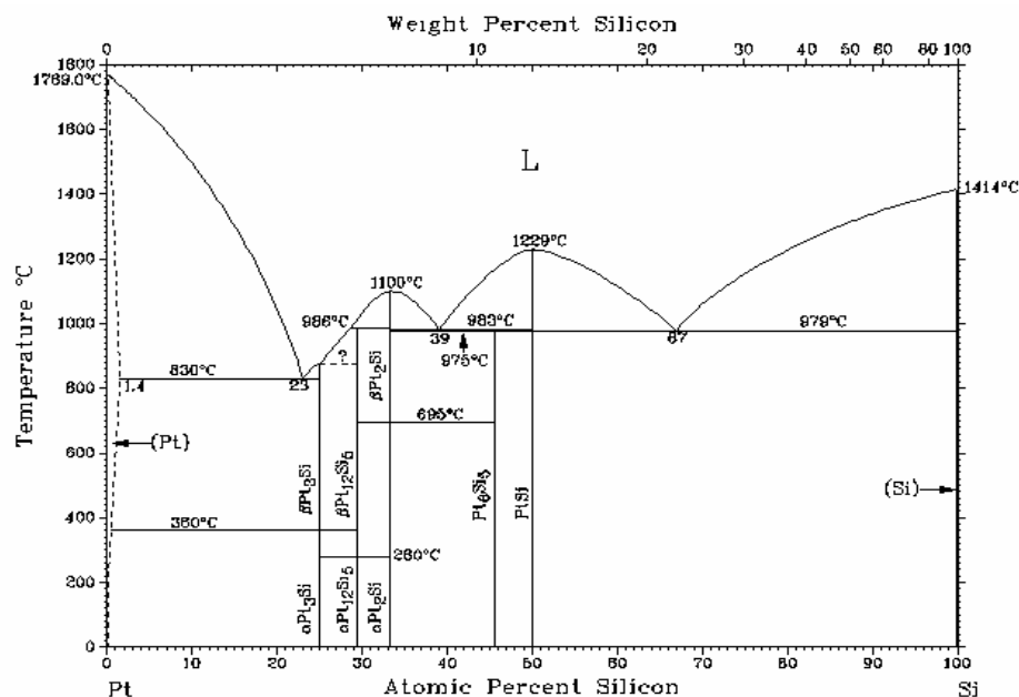
Figure 14 : Diagramme d'équilibre de phases du système binaire platine-silicium 63
