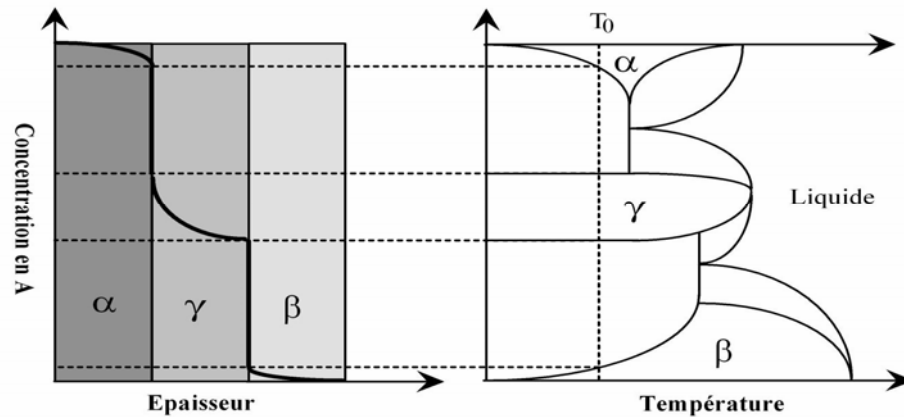
Figure 4 : Profil de concentration de l'élément A (partie gauche) prédit par le diagramme de phases (partie droite) pour le couple A/B après traitement thermique à une température T_0 .
