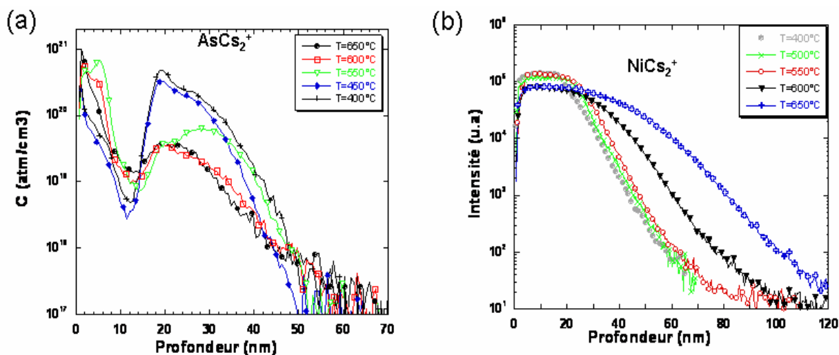
Figure 55 : (a) Profils SIMS en profondeur de la concentration d' \text{AsCs}_2^+ après siliciuration à différentes températures, (b) Signal du \text{NiCs}_2^+ après siliciuration à différentes températures.
