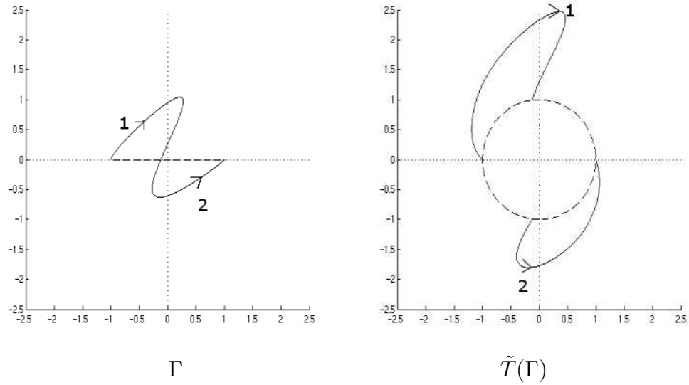
FIGURE 2 : \Gamma intersecte [-1, 1] en un point
