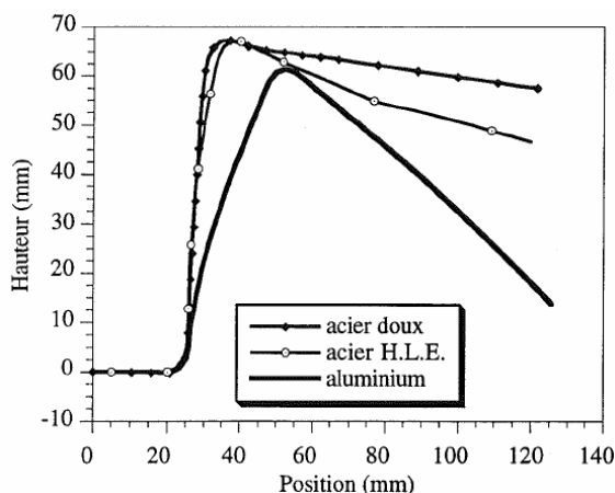
Figure 6.5 – Influence du matériau sur la forme de la pièce après retour élastique [19].
