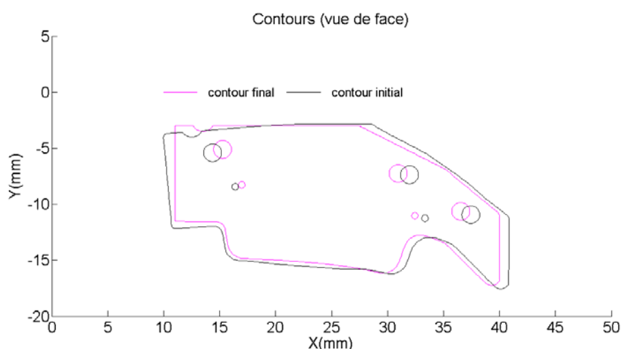
Figure 3.25 – Vue de dessus du contours de la pièce (avant et après mise en forme).
