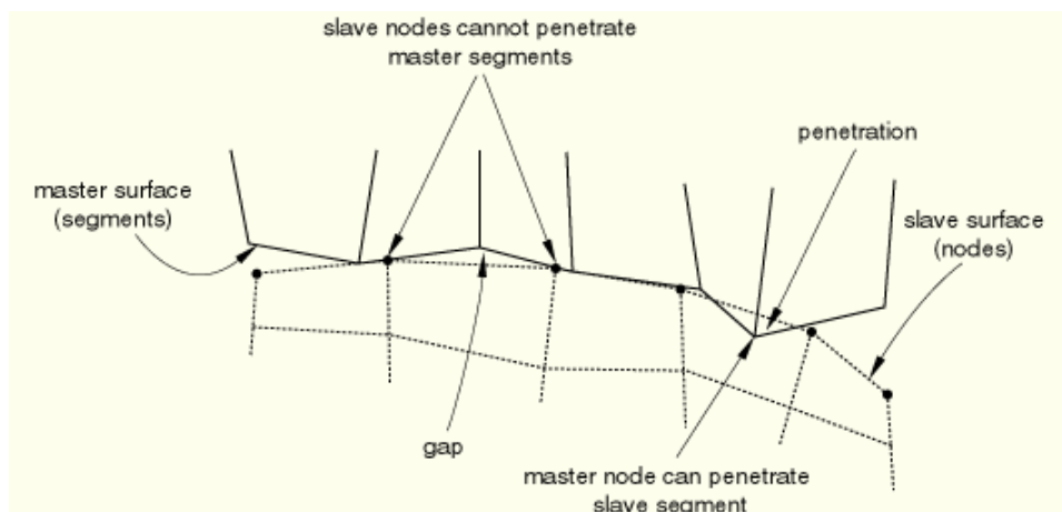
Figure 3.2 – Condition d'impénétrabilité [2].
