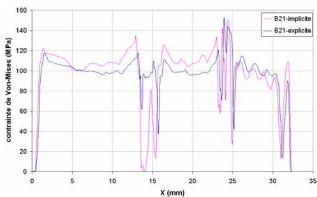
(b) – Contrainte de Von-Mises en MPa au niveau de la surface du bas après retour élastique.
