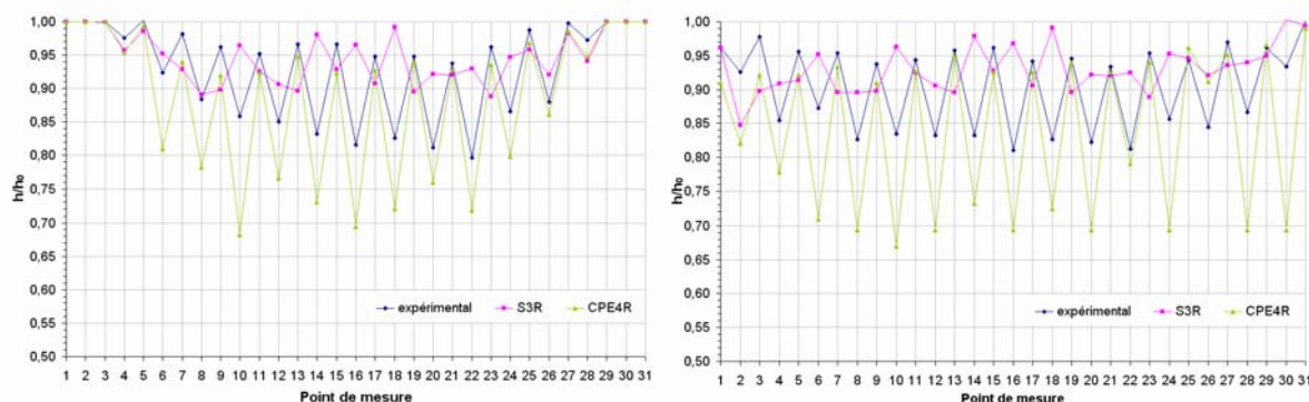
(c) – Variations d'épaisseur – passe n°3.
