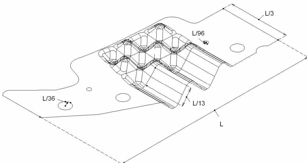
Figure A.2 – Forme de la pièce et données dimensionnelles en vue isométrique.
