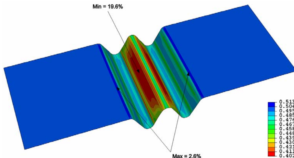
Figure 3.13 – Variations d'épaisseur.
