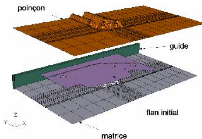
Figure 3.24 – Outils d'emboutissage.
