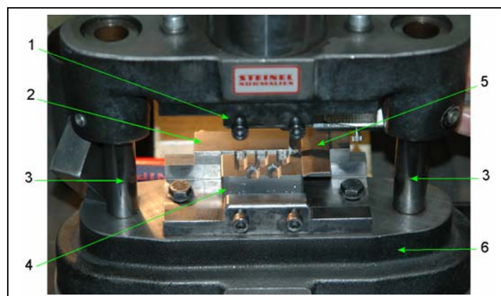
1 : poinçon - 2 : guide - 3 : colonne de guidage - 4 : matrice - 5 : butée - 6 : bâti.
