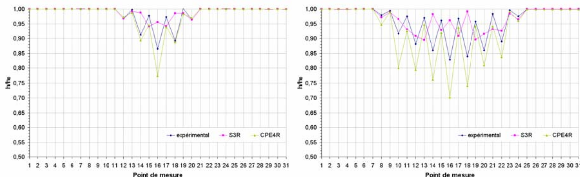
(a) – Variations d'épaisseur – passe n°1.
