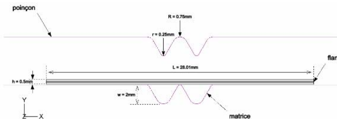
Figure 3.9 – Outils d'emboutissage.
