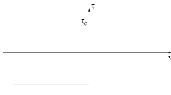
Figure 3.3 – Représentation du modèle de Coulomb.
