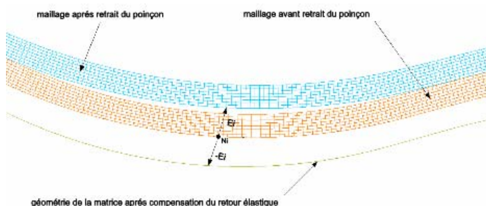
Figure 6.30 – Compensation du retour élastique.
