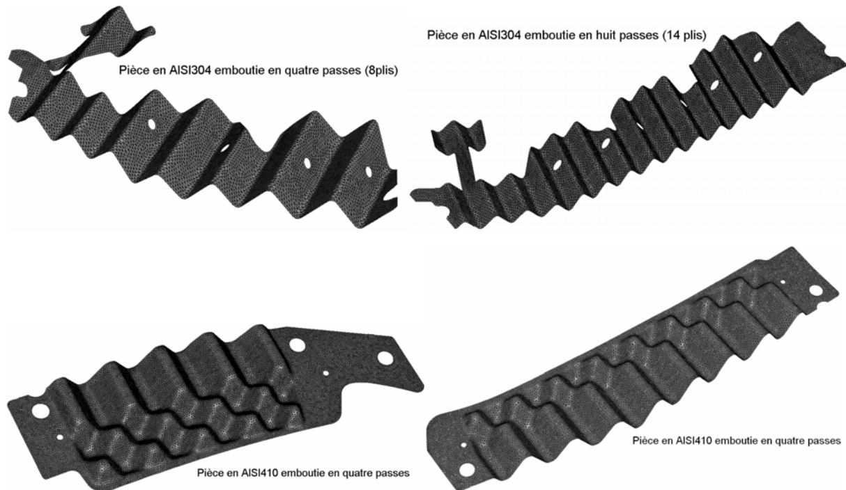
Figure 5.25 – Géométrie de pièces obtenues par optimisation heuristique.
