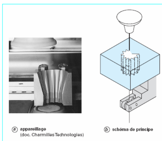
Figure 2.3 – Principe de la découpe par fil [1].
