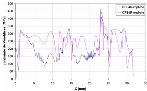
(c) – Contrainte de Von-Mises en MPa au niveau de la surface supérieure avant retour élastique.
