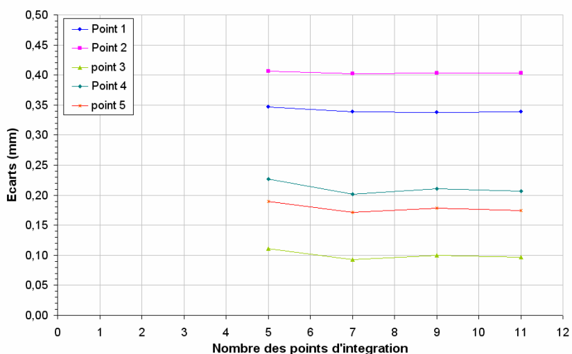
Figure 3.31 – Evolution des écarts de forme en fonction du nombre de points d'intégration.
