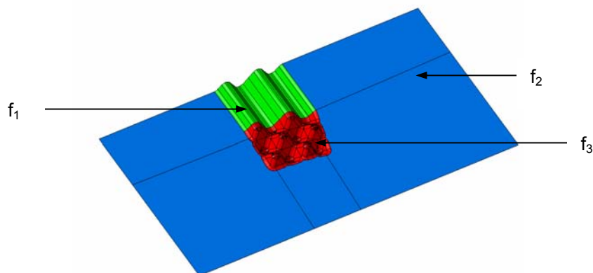
Figure 3.33 – Partition de la surface de l'outil en fonction de l'état de surface.
