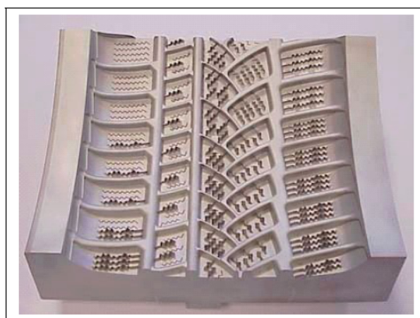
Figure 1.2 – Emplacement des lamelles dans le moule.
