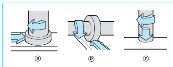
Figure 2.5 – Méthodes de fraisage [2].
