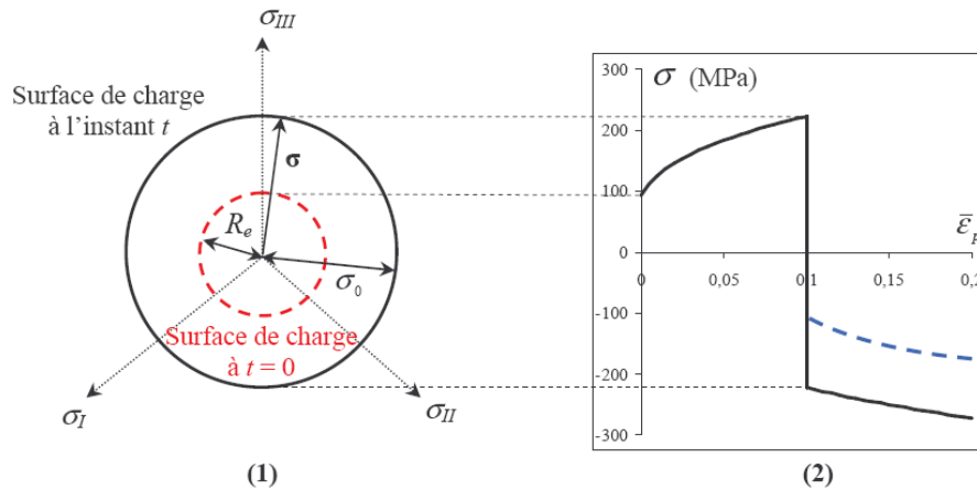
Figure 3.5 – Représentation de l'écroutissage isotrope sans l'effet Bauschinger [4].
