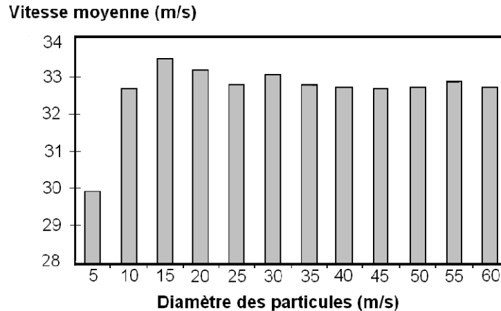
Figure I-24 : Vitesse moyenne en sortie de l'injecteur des particules de zircone -45+22 \mu\text{m} en fonction de leur diamètre
