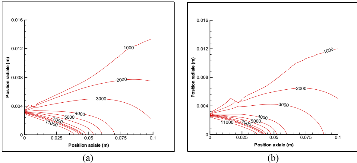
Figure IV-18 Iso-temperatures dans le plan axial contenant l'injecteur pour des jets Ar-H 2 25% vol de débits respectifs (a) 50 L.min -1 et (b) 70 L.min -1
