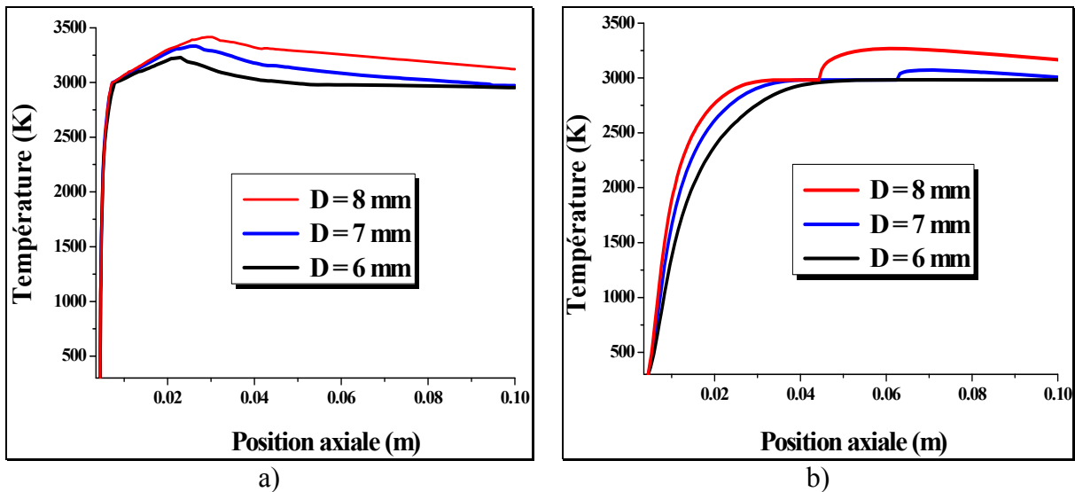
Figure IV-28 : Comparaison (a) des température à la surface et (b) au centre d'une particule de zircone de 25 μm de diamètre injectée dans des jets Ar-H 2 25% vol. pour différents diamètres de tuyère
