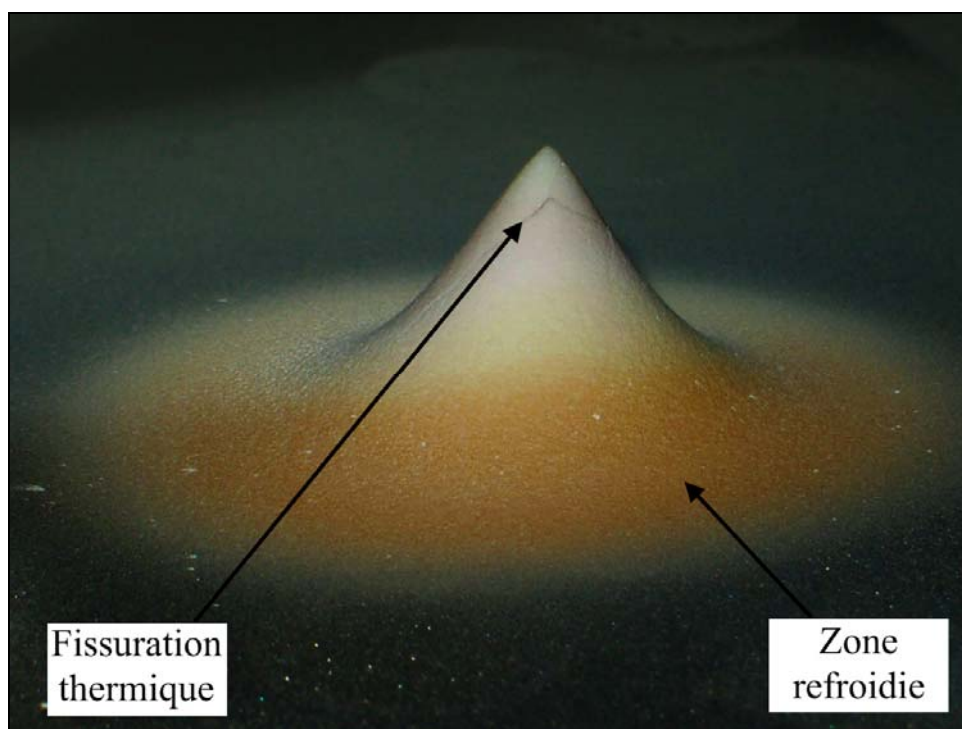
Figure A3- 1 : Recouvrement réalisé avec une poudre hydroxyapatite ( 16 \text{ g}\cdot\text{min}^{-1} ) pendant 2 min
