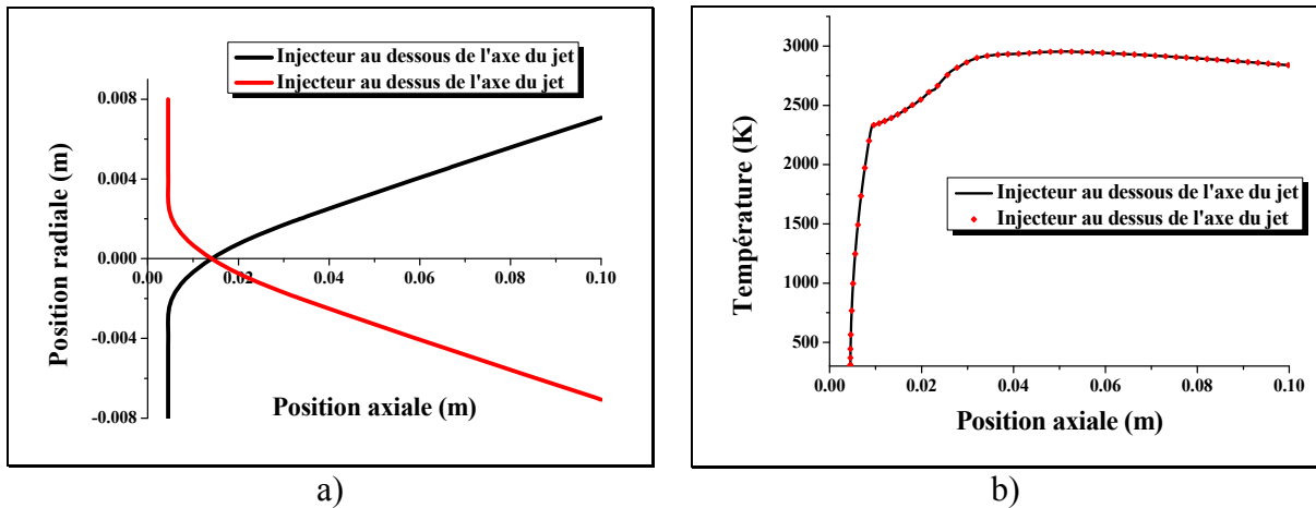
Figure IV-13 : Comparaison (a) des trajectoires et (b) des températures d'une particule d'alumine de 30\ \mu\text{m} de diamètre injectée au-dessus et au-dessous de l'axe de la torche, dans les conditions de projection de référence
