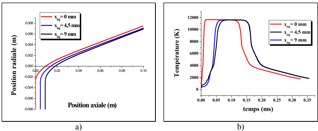
Figure IV-14 : Comparaison des (a) Trajectoires et (b) Températures de plasma vues par des particule d'alumine de 30\ \mu\text{m} de diamètre injectées à différentes positions axiales, dans les conditions de projection de référence
