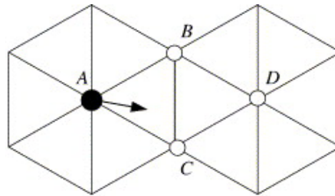
Figure I-31 : Mouvement d'une particule dans un réseau de Lattice-Boltzmann selon Zhang et al. [117, 118]
