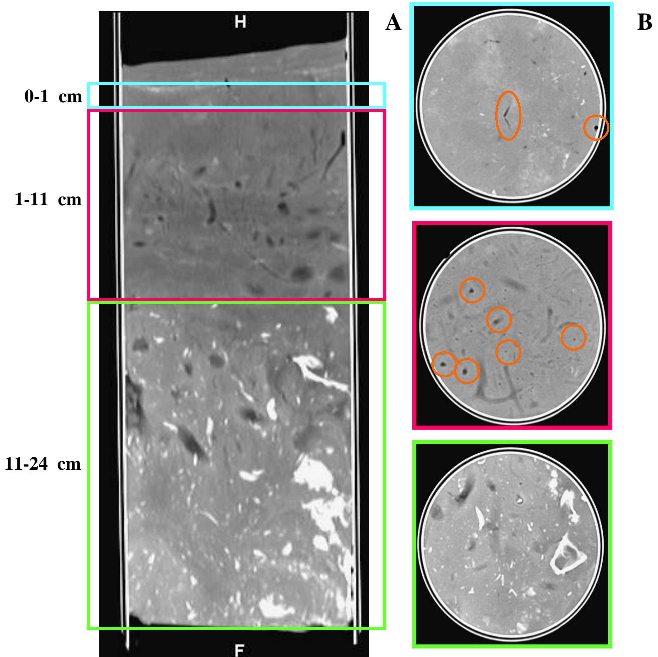
Figure 6 : Coupes longitudinale (a) et transversales (b) de la carotte sédimentaire prélevée dans la station R4 de Rivedoux obtenues grâce à l'utilisation de la tomodynamométrie axiale (rond orange : polychètes cirratulidés)
