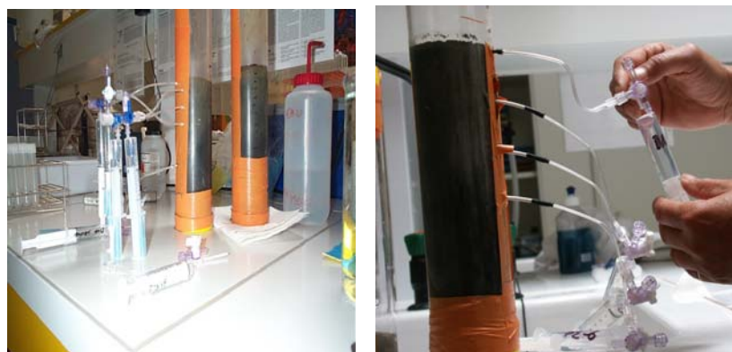
Figure 8 : Extraction de l'eau interstitielle à l'aide de rhizons
