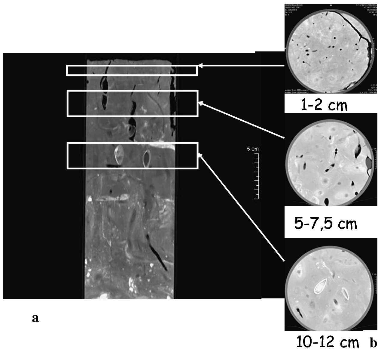
Figure 4 : Coupes longitudinale (a) et transversales (b) de la carotte sédimentaire prélevée dans la station d'Esnandes obtenues grâce à l'utilisation de la tomographie axiale.
