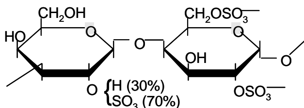
Figure 2.5: Structure chimique du carraghénane de type \lambda .
