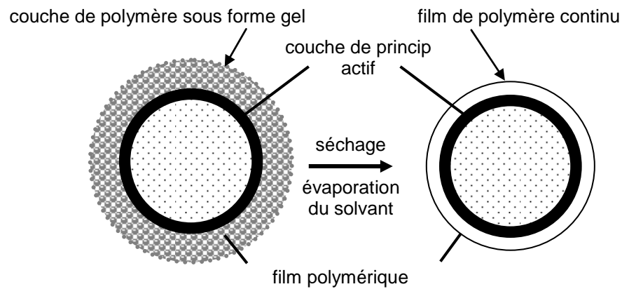
Figure 2.2: Représentation schématique du mécanisme de formation du film à partir de solutions organiques polymériques.
