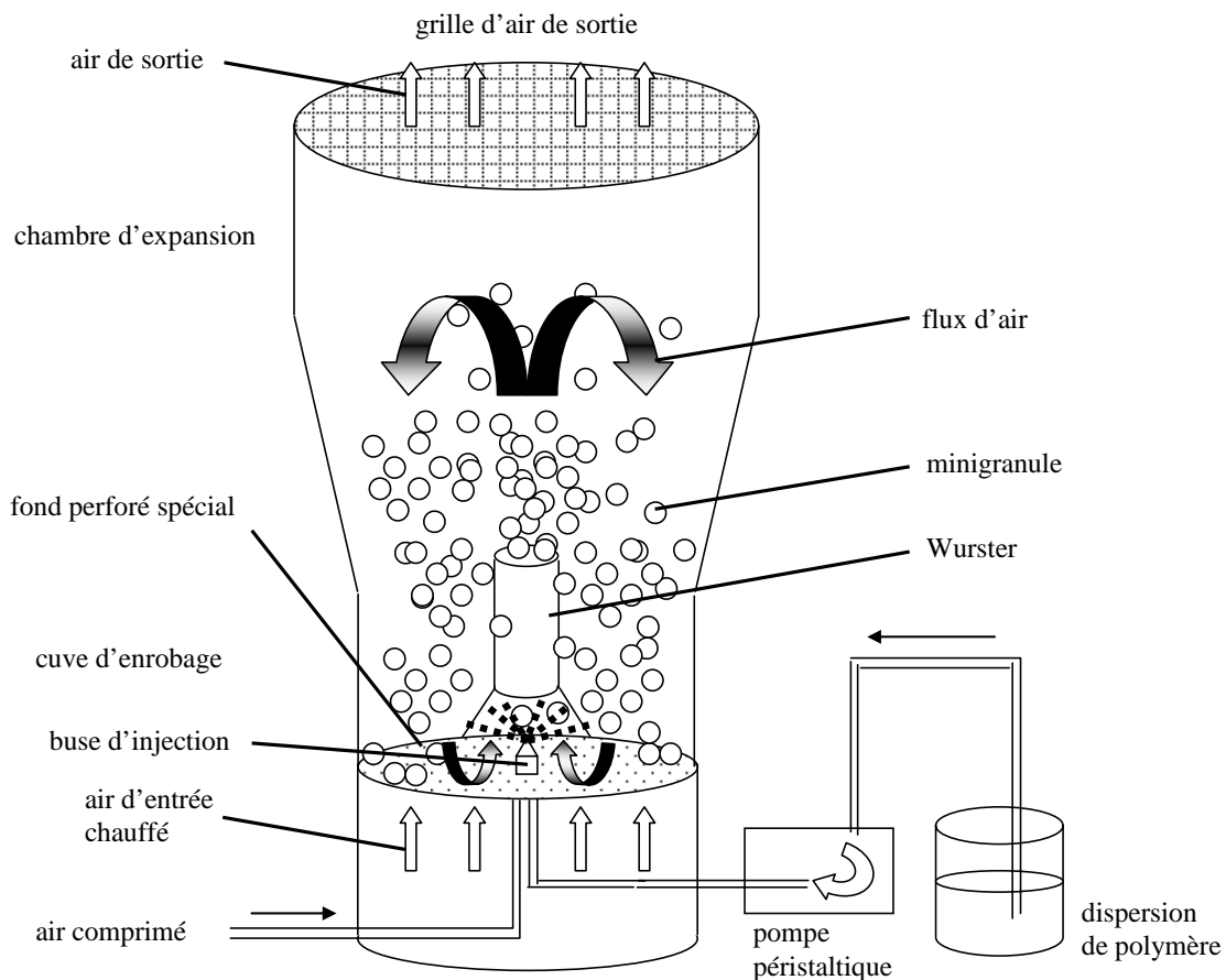
Figure 2.1: Représentation schématique d'un lit d'air fluidisé équipé d'un Wurster.
