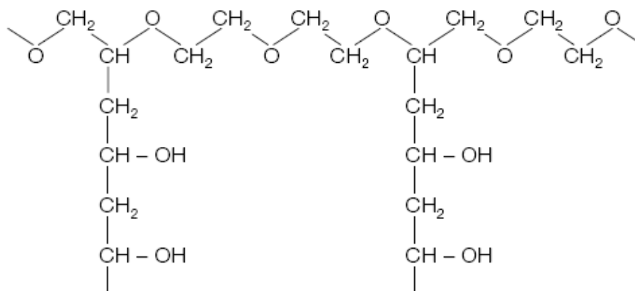
Figure 2.7: Structure chimique du copolymère d'acide polyvinylique et de polyéthylène glycol.
