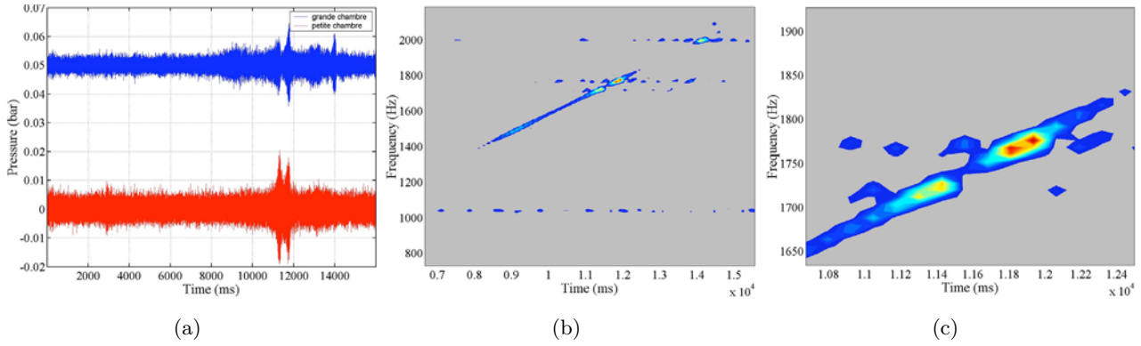
Fig. A.6: Amplitude des oscillations dans les 2 cavités au cours d'une excitation en rampe ( 100 \text{ Hz}\cdot\text{s}^{-1} ) avec une fréquence d'acquisition de 8192 \text{ Hz} (a) et la Transformée de Fourier du signal de pression dans la grande cavité (b) lors de la modulation linéaire en fréquence (c : zoom sur les pressions de forte amplitude). On utilise ici la plaque perforée à 60 trous.
