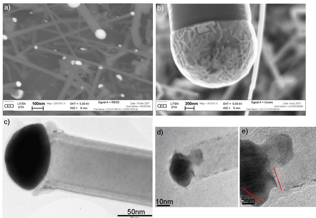
Figure 3.15 – Observations de gouttes d'or vues a) en MEB rétrodiffusé, b) en MEB, c) en MET conventionnel et d-e) en HR-MET. L'aspect polycristallin est visible sur la goutte d'or des images d) et e).
