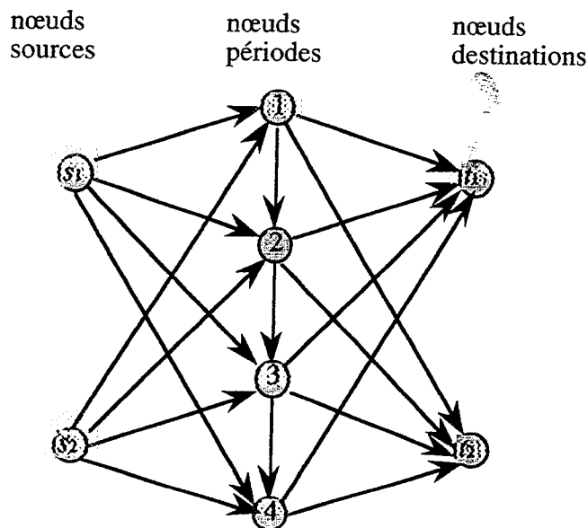
Figure I.2 Stockage optimal de produits saisonniers.
