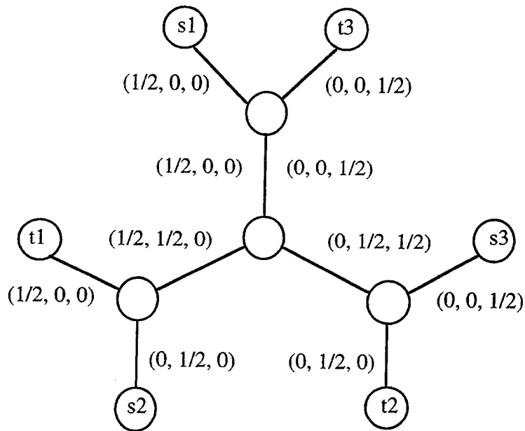
Figure III.2 Triflot maximum (toutes les capacités sont égales à 1.) Le flot maximum est de 1.5, la coupe minimum est de 2.
