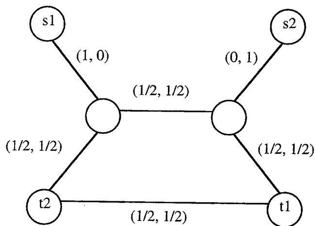
Figure III.1 Biflot maximum, avec flots fractionnaires.
