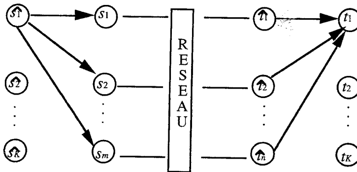
Figure II.4 Exemple de réseau (EPPS) .
