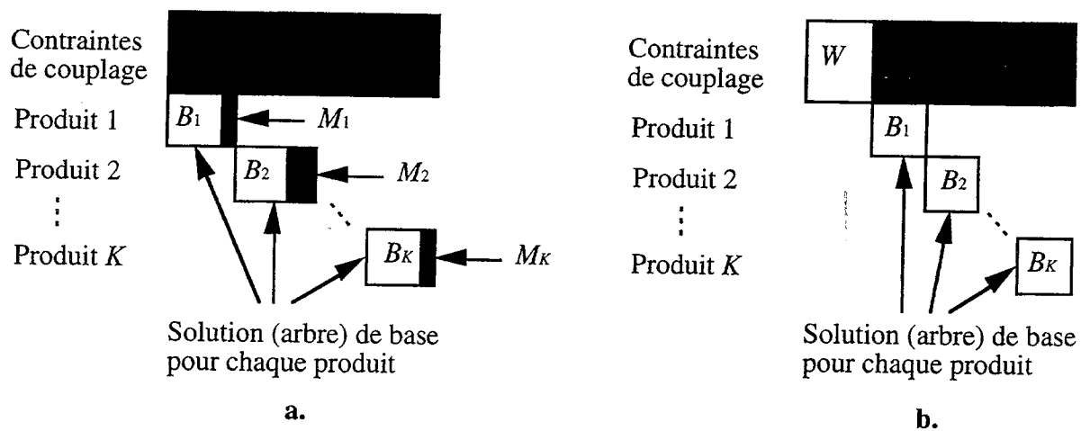
Figure II.7 Partitionnement de la base pour un problème de multiflot:
