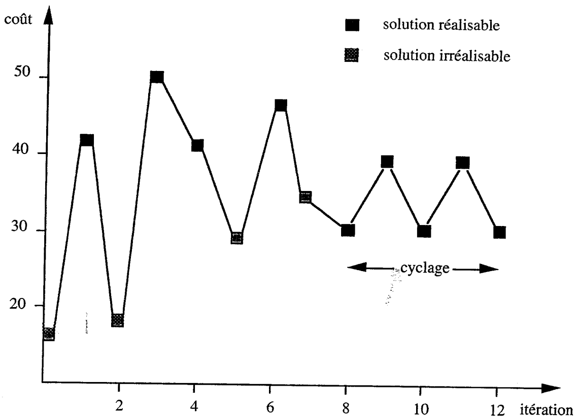
Figure IV.5 Exemple de cyclage.
