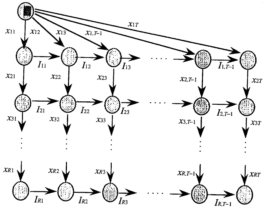
Figure I.4 Modèle de planification production-stockage.
