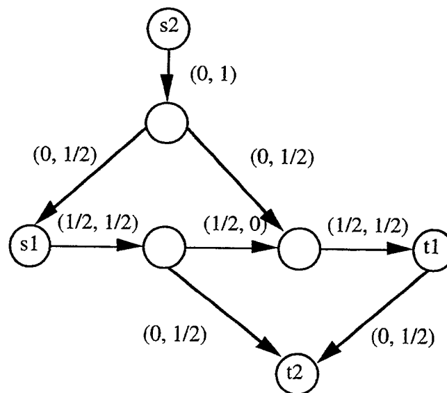
Figure III.4 Le flot maximum est inférieur à la coupe minimale.
