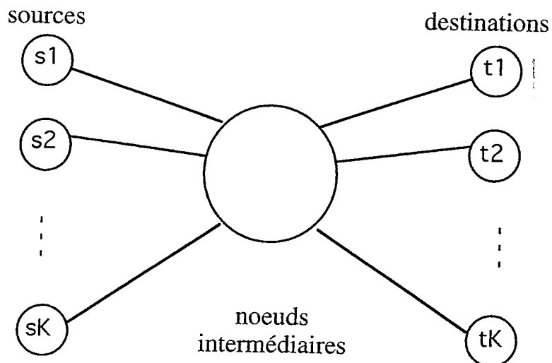
Figure III.6 Structure requise pour un multiflot complètement planaire.
