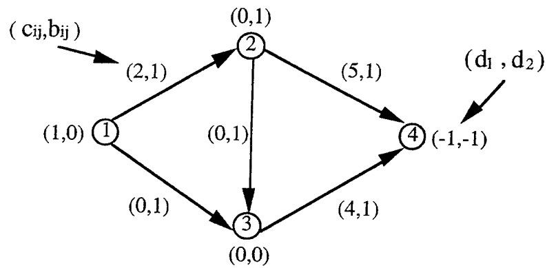
Figure IV.1 Exemple de biflot.
