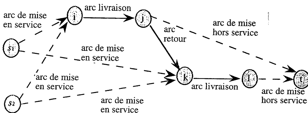
Figure I.3 Ordonnancement d'une flotte de navires-citernes.
