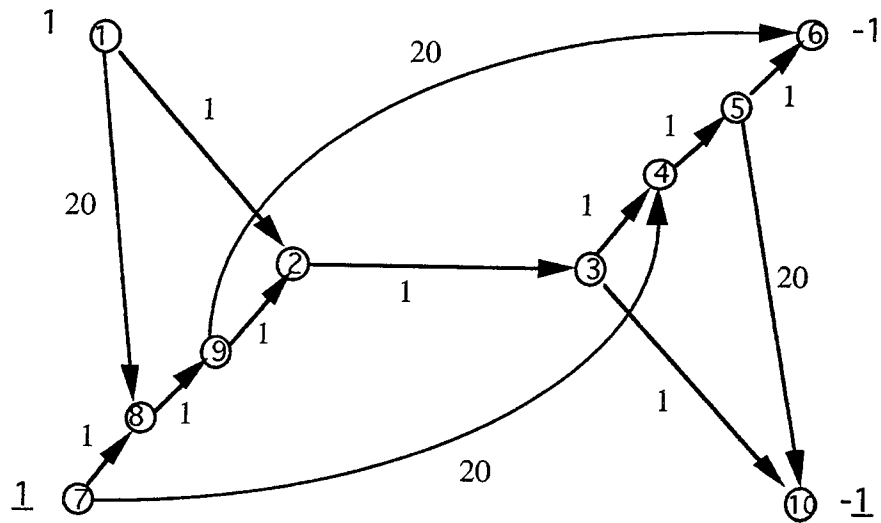
Figure IV.4 Exemple de biflot.
