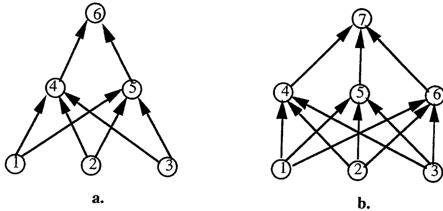
Figure II.2 Énumération de points extrêmes pour les chemins et les arbres.
