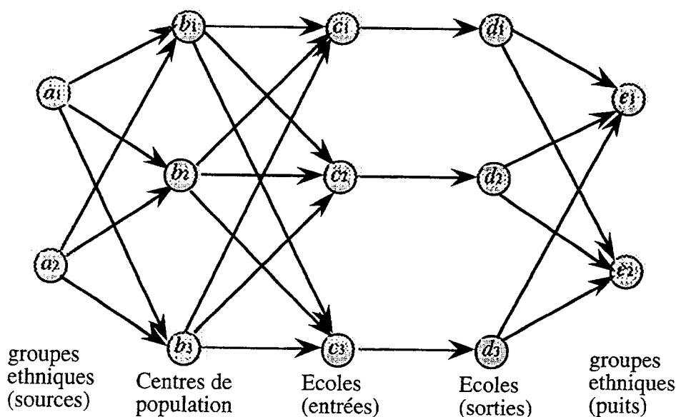
Figure I.5 Modèle de multiflots pour le problème d'équilibre racial dans une école.
