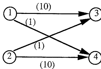
Figure II.3 Exemple de réseau.
