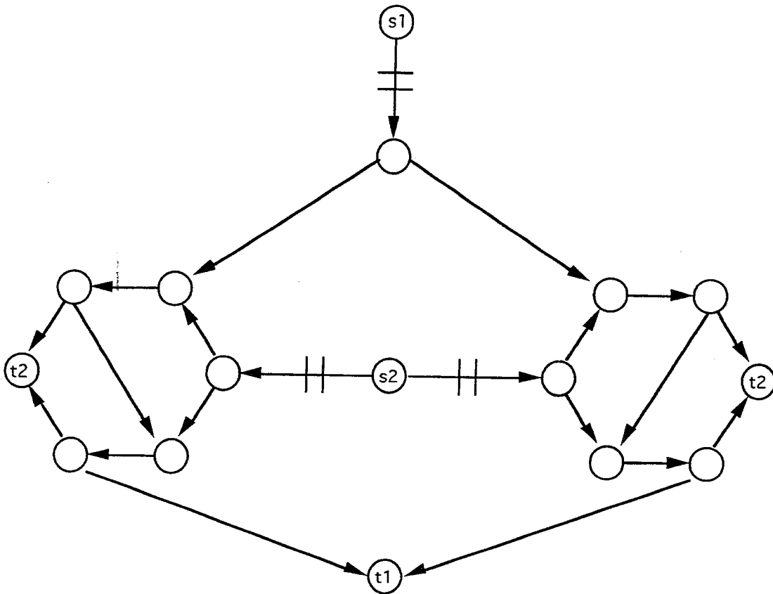
Figure III.7 Le flot maximum est réalisé pour d^1 = 1 , d^2 = 2 , la capacité de la coupe minimale est égale à 3 (toutes les capacités sont égales à 1). Mais les flots sur les arcs sont de 0,5.
