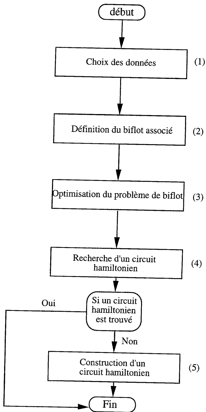
Figure V.6 Schéma global d'optimisation du problème de voyageur de commerce.
