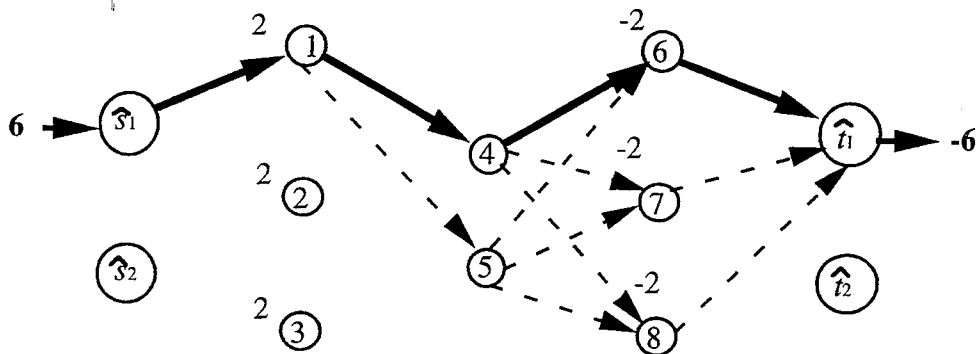
Figure II.5 Exemple de sous-problème ( EPPS ).
