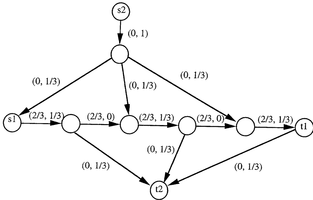
Figure III.5 Biflot à valeurs rationnelles (les capacités sont égales à 1.)
