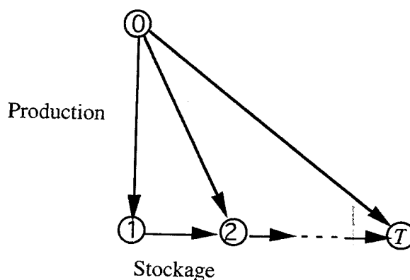
Figure II.10 Réseau de production dynamique à une seule période
