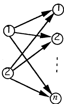
Figure II.9 Réseau de transport à 2 sources.
