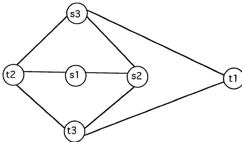
Figure III.3 Multiflot à coût minimum. (les capacités sont égales à 2).
