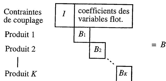
Figure II.1 Base initiale formée des bases individuelles des sous-problèmes.
