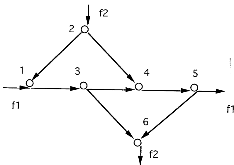
Figure I.1 Exemple de multiflot.
