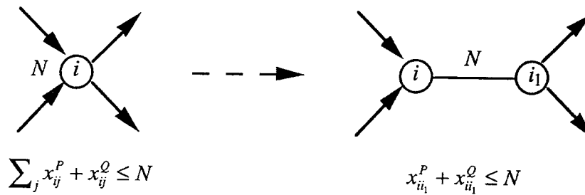
Figure V.1 Transformation de la contrainte de flot sur les sommets en contrainte de capacité sur les arcs.
