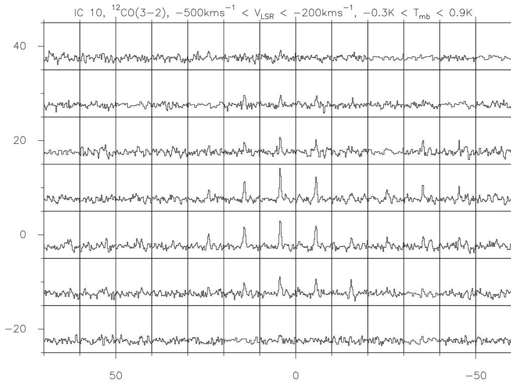
FIG. 3.15 – Carte de spectres de la galaxie IC 10. Voir la légende de la Fig. 3.4.
