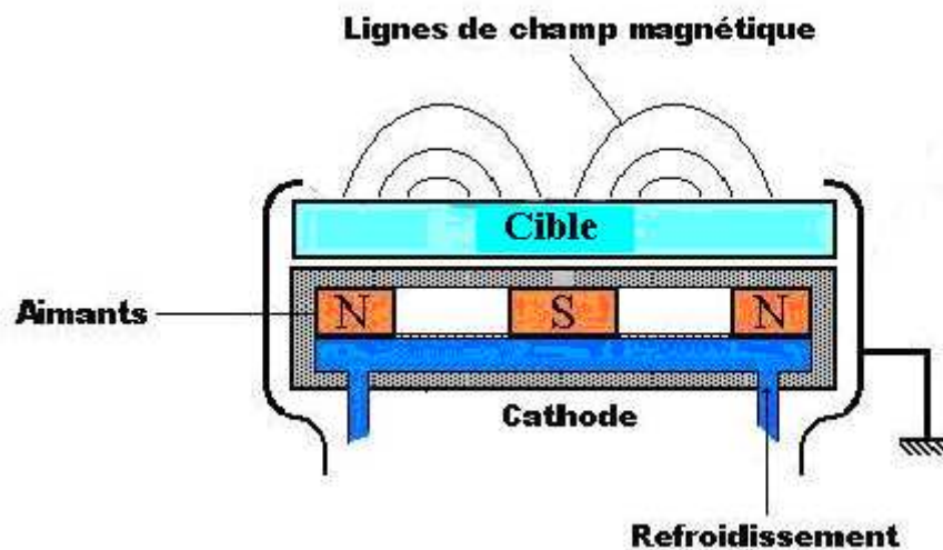
Figure II-3 : Schéma d'une cathode magnétron.
