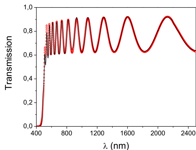
Figure V-2 : Spectres de transmission optique expérimental (trait plein) et simulé (cercles) d'un film déposé à P_{RF} = 150 W pendant 15 min. L'ajustement des données expérimentales et simulées a été réalisé avec le logiciel SCOUT.
