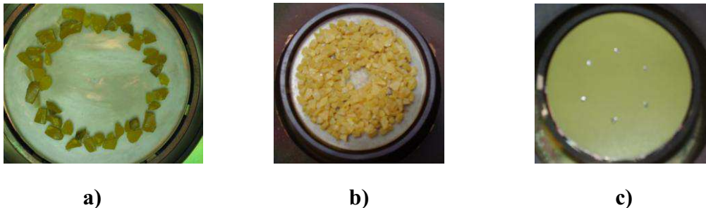
Figure II-5 : Photos des cibles utilisées, a) cible de \text{SiO}_2 recouverte de chips de ZnSe (rapport surfacique \text{ZnSe}/\text{SiO}_2 = 30\% ) ; b) cible de \text{SiO}_2 recouverte de chips de ZnSe et de Cr (rapport surfacique \text{ZnSe}/\text{SiO}_2 = 80\% ) ; c) cible de ZnSe massive recouverte de chips de Cr.
