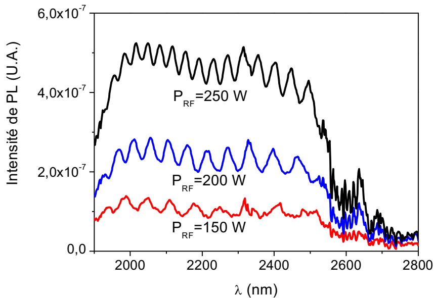
Figure V-8 : Spectres de photoluminescence de films de \text{Cr}^{2+}:\text{ZnSe} ( M_{\text{Cr}}=0.17 \text{ g} ) déposés pour différentes valeurs de P_{\text{RF}} en excitant à 1.85 \mu\text{m} à température ambiante. Les spectres ont été normalisés par leur épaisseur et corrigés de la réponse du montage.
