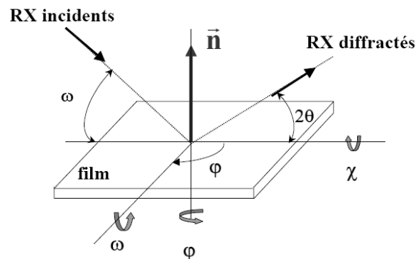
Figure II-12: Définition des angles \chi , \varphi et \theta par rapport à la surface du film repérée par sa normale \vec{n} .
