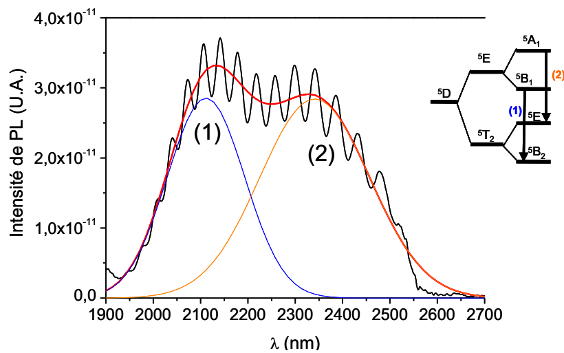
Figure V-11 : Spectre de photoluminescence à 10 K décomposé par deux gaussiennes centrées vers 2110 et 2340 nm qui correspondent respectivement aux transitions {}^5B_1({}^5E) \rightarrow {}^5B_2({}^5T_2) et {}^5A_1({}^5E) \rightarrow {}^5E({}^5T_2) .
