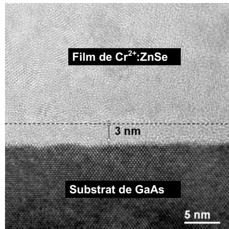
Figure IV-21 : Image de MET en haute résolution montrant la couche amorphe (environ 3 nm d'épaisseur) à l'interface du substrat de GaAs avec le film déposé à P_{RF} = 100 \text{ W} pendant 1 h.
