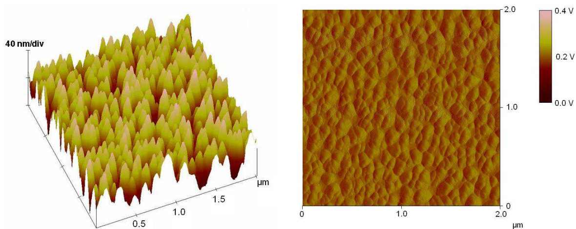
Figure IV-6 : Micrographies AFM 3D et 2D d'un film déposé sur substrat de GaAs pour P_{RF} = 250 \text{ W} durant une heure. Sur cette surface de 2 \text{ \mu m} \times 2 \text{ \mu m} , la rugosité ( \sigma_{AFM} ) a été estimée à 13 nm.
