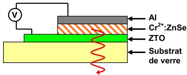
Figure 1 : Dispositif en vue de l'optimisation des propriétés d'électroluminescence des films déposés.
