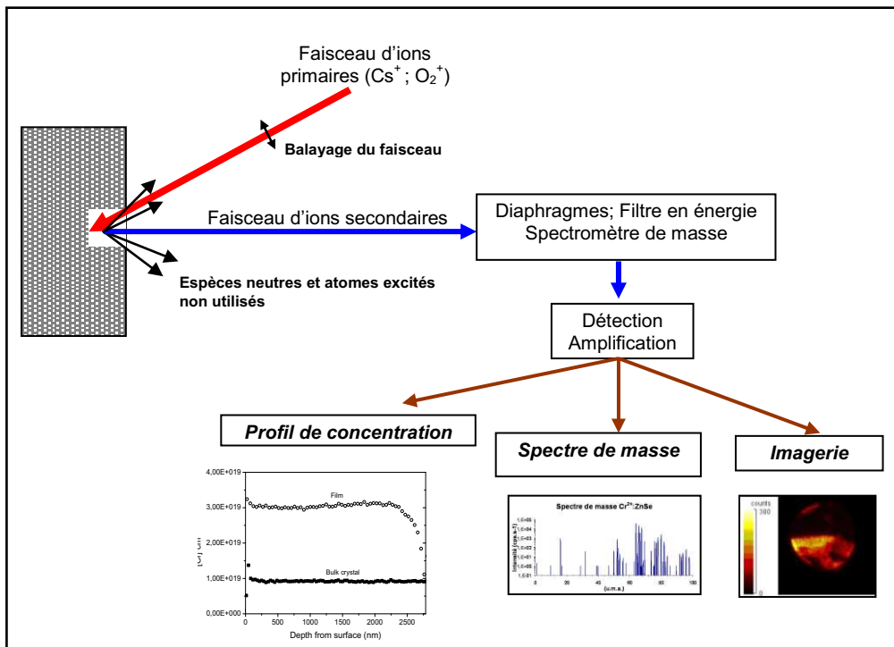
Figure II-19 : Principe de la spectroscopie de masse d'ions secondaires.
