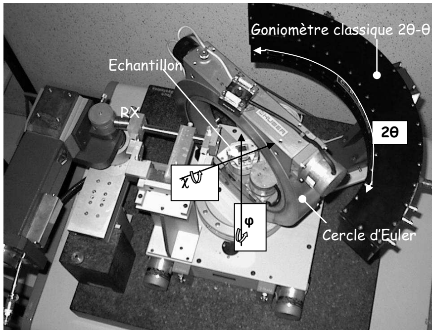
Figure II-13 : Vue de dessus du goniomètre quatre cercles du laboratoire CRISMAT.
