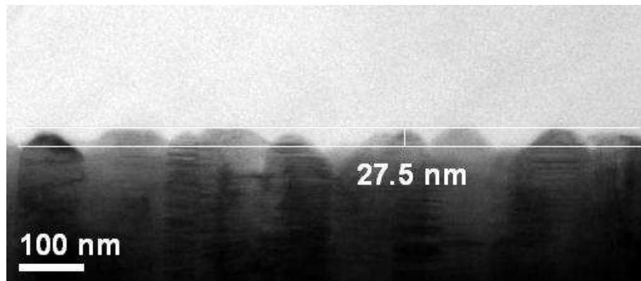
Figure IV-7 : Image de MET d'un film déposé sur substrat de GaAs ( P_{RF} = 100 W, durée = 1 h) qui met en évidence la présence de bosses à la surface de l'échantillon en accord avec la valeur de rugosité de surface élevée mesurée en AFM ( \sigma_{AFM} = 13 nm) et XRR ( \sigma_2 = 12,4 nm).
