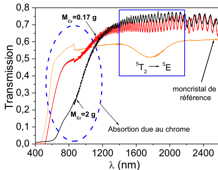
Figure V-3 : Spectres de transmission optique du monocristal de référence ( e = 500 \mu\text{m} ) et de deux films ( e = 18 \mu\text{m} environ) de \text{Cr}^{2+}:\text{ZnSe} déposés avec M_{\text{Cr}} = 0.17 \text{ g} et M_{\text{Cr}} = 2 \text{ g} . Les oscillations observées proviennent des réflexions multiples sur les faces du film. Le décrochement observé vers 850 nm est dû au changement de détecteur du spectromètre.
