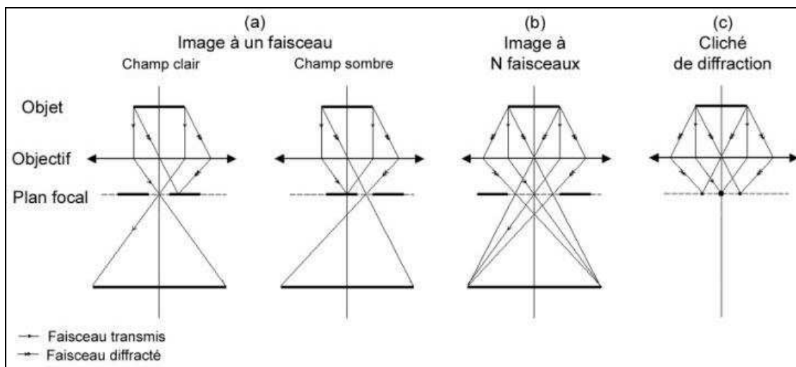
Figure II-14: Formation des différents modes d'observations en microscopie électronique.
