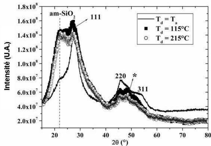
Figure III-9 : Spectres de diffraction X asymétriques normalisés pour des films déposés sur substrat de a-SiO 2 à P_{RF} = 100 W, d = 7 cm et T_d comprise entre T_a et 215 °C. La contribution amorphe du substrat (am-SiO 2 ) est d'autant plus marquée que T_d augmente.
