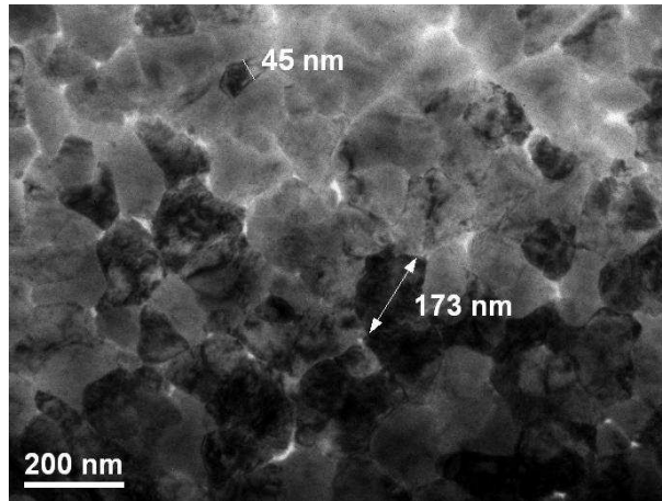
Figure IV-20 : Image de MET en vue plane d'un film déposé sur substrat de GaAs ( P_{RF} = 150 \text{ W} , durée = 1 h).
