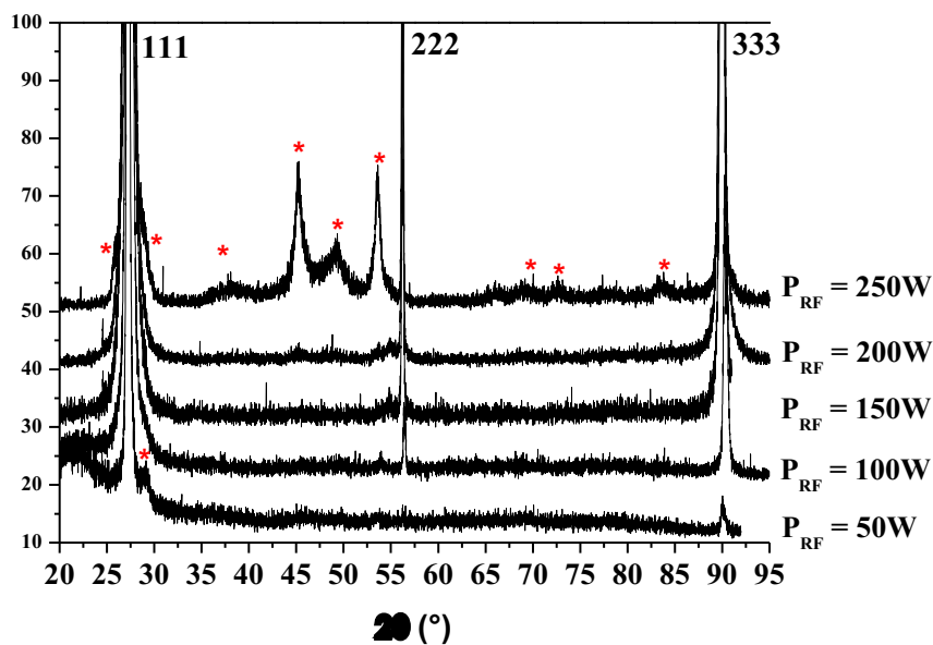
Figure IV-9 : Diagramme de diffraction X ( \theta-2\theta ) pour les films déposés sur substrat de \text{a-SiO}_2 pendant une heure pour différentes valeurs de P_{\text{RF}} . Le symbole * correspond à la phase hexagonale du ZnSe.
