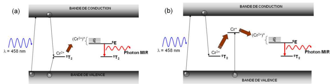
Figure V-18 : Deux mécanismes d'excitation possible des ions \text{Cr}^{2+} avec une énergie d'excitation supérieure au gap (a) : capture d'un exciton par l'ion dopant \text{Cr}^{2+} ; (b) capture des porteurs par les espèces ionisées ( \text{Cr}^{2+} , \text{Cr}^+ ).
