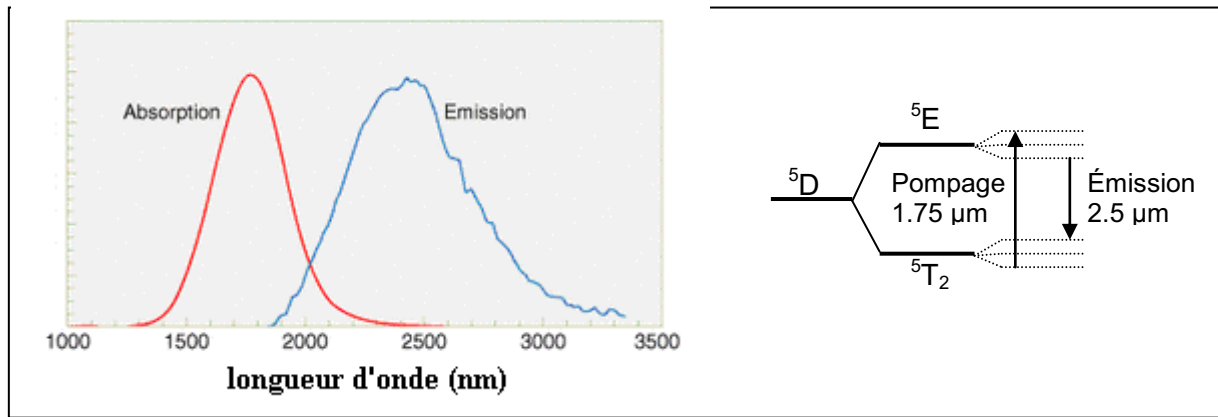
Figure I-9 : Spectres à température ambiante d'absorption et d'émission d'un cristal de \text{Cr}^{2+}:\text{ZnSe} et le diagramme d'énergie correspondant. Sur le schéma de droite, les sous niveaux d'énergie représentés correspondent à des niveaux vibrationnels, à ne pas confondre avec les sous niveaux Jahn-Teller.
