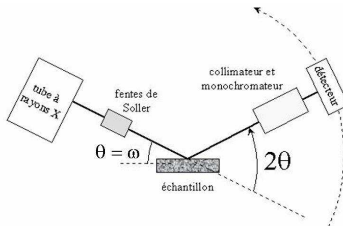
Figure II-11 : Dispositif expérimental de diffraction des rayons X.
