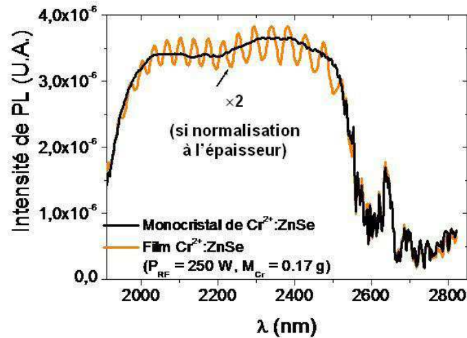
Figure V-9 : Comparaison des spectres de photoluminescence normalisés à l'épaisseur du film « optimisé » et du monocristal de référence acquis à température ambiante en excitant à 1.85 \mu\text{m} .
