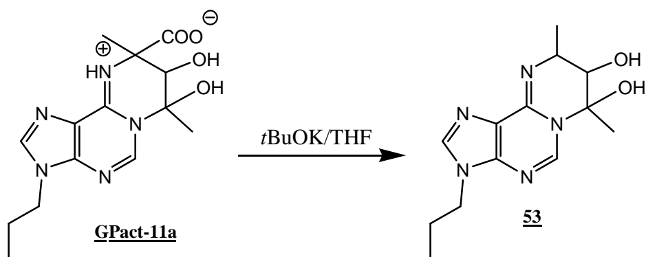
Schéma 20 : Formation du mélange d'isomères du produit de la famille III 53 à partir des adduits du MG sur la 9-propyladénine GPact-11a
