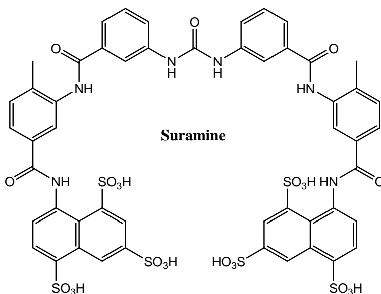
Figure 41 : Structure de la suramine
