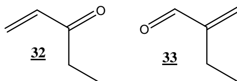
Figure 55 : Structures de la 1-éthylacroléine 32 et de la 2-éthylacroléine 33
