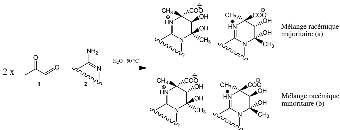
Schéma 1: Réaction entre le MG 1 et un \alpha -aminoazahétérocycle 2 et structures des différents isomères formés
