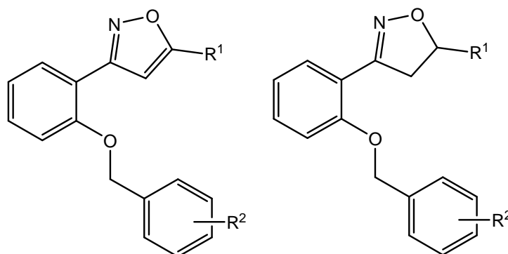
Figure 23 : Structures des dérivés de 3-(2-benzyloxyphenyl)isoxazoles et isoxazolines
