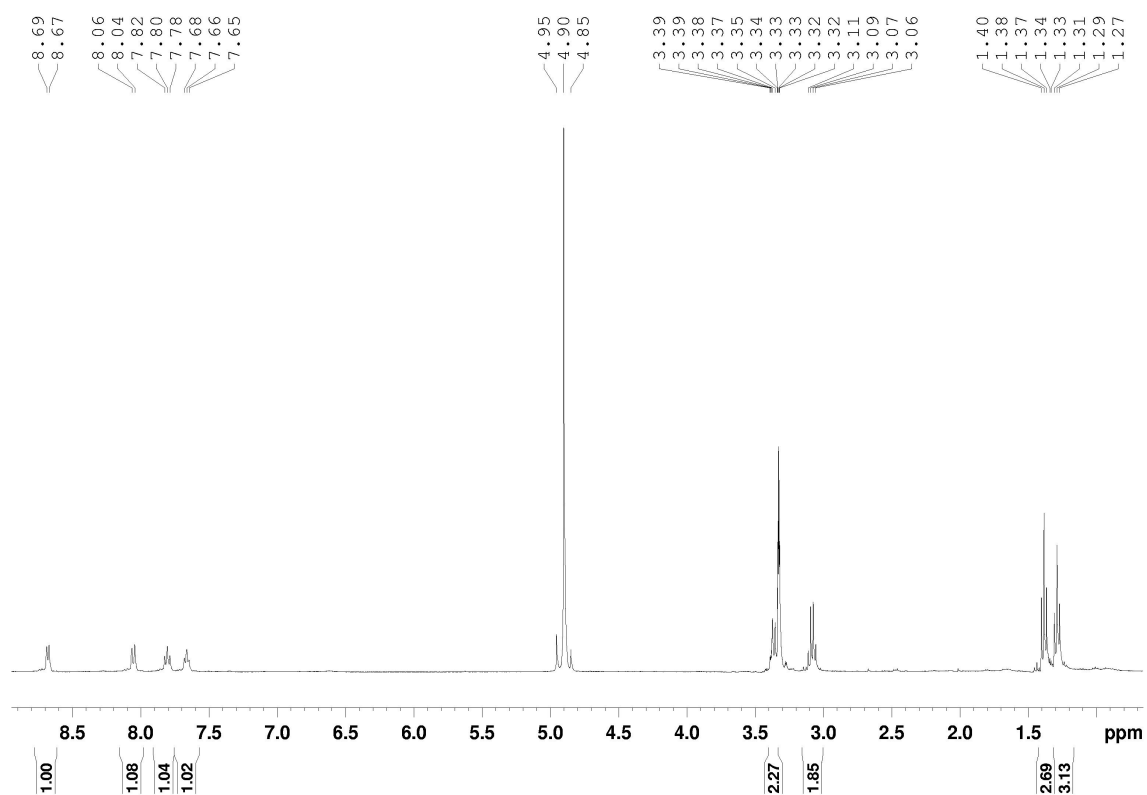
Figure 58 : Spectre de RMN ^1\text{H} à 400 MHz dans CD 3 OD à 21 °C du composé 48
