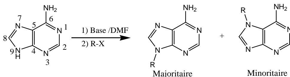
Schéma 34 : Voie d'accès aux dérivés de l'adénine modifiée en position 7
