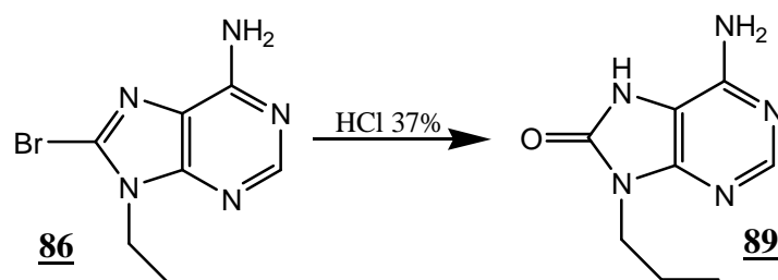
Schéma 40 : Synthèse de la 8-hydroxy-9-propyladénine 89 par hydrolyse acide de la 8-bromo-9-propyladénine 86
