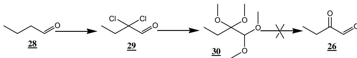
Schéma 6 : Synthèse de l'EG décrite par (Verhe, 1982)
