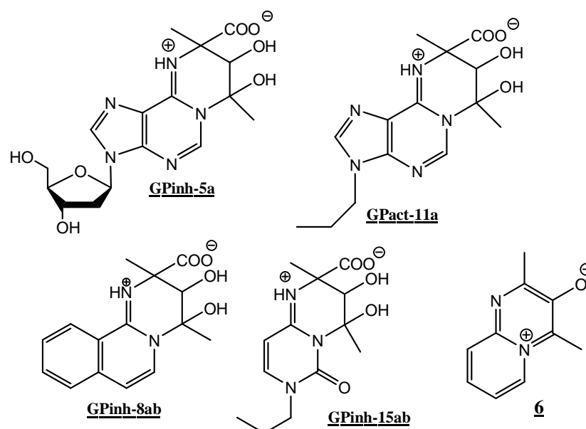
Figure 73 : Structures des composés évalués par des tests ADMET
