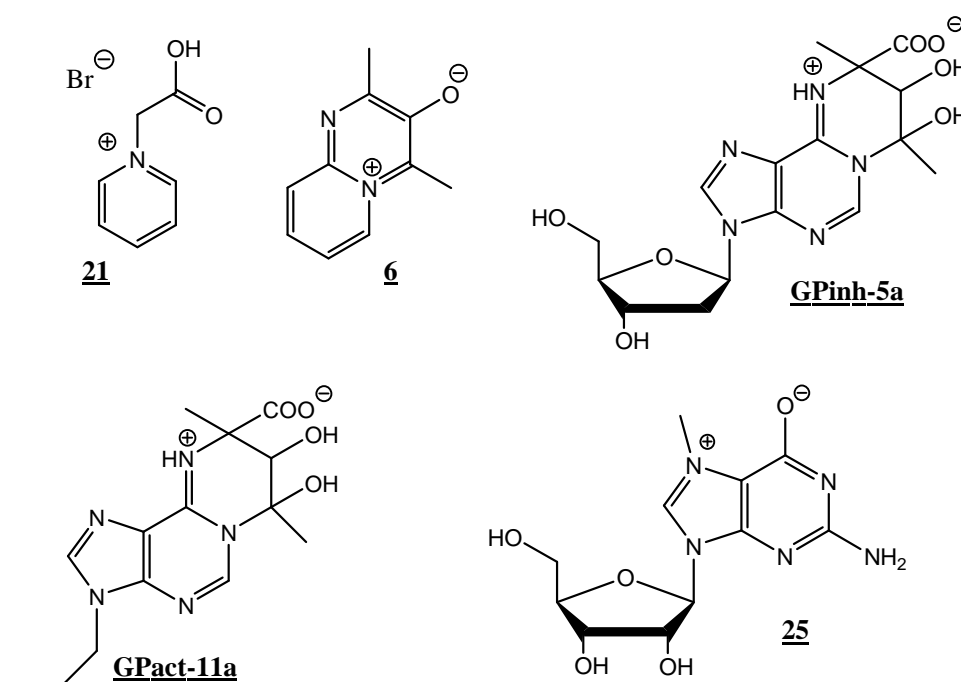
Figure 72 : Structures des composés évalués en tant que correcteur de la protéine delF508-CFTR
