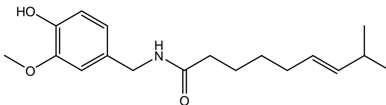
Figure 20 : Structure de la capsaïcine
