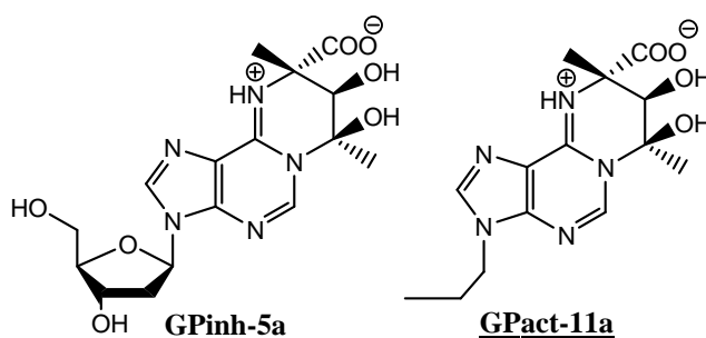
Figure 90 : Structures de deux modulateurs de la protéine CFTR mis en évidence : l'inhibiteur GPinh-5a et le potentiateur/activateur GPact-11a
