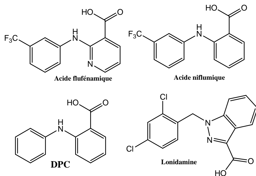
Figure 30 : Structures des acides carboxyliques aromatiques inhibant CFTR de façon non sélective
