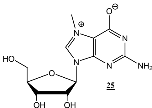
Figure 54 : Structure de la 7-méthylguanosine 25
