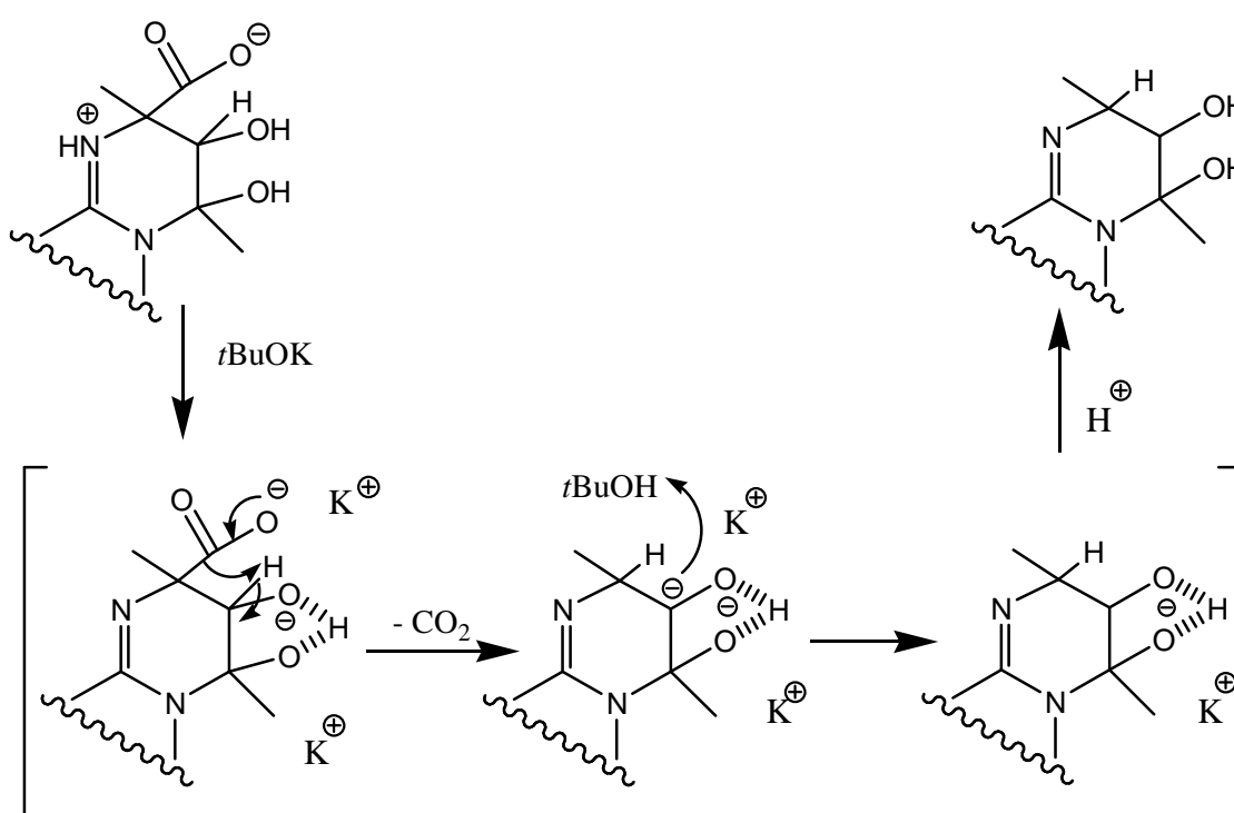
Schéma 26: Deuxième hypothèse de mécanisme de la réaction menant à la famille III
