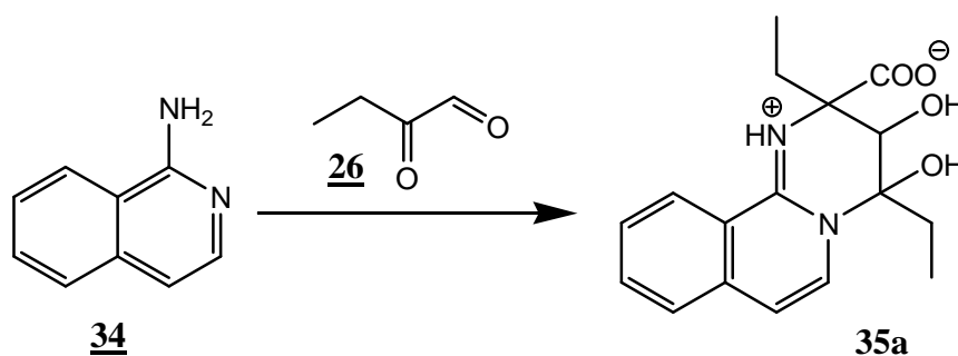
Schéma 9 : Réaction de l'EG 26 sur la 1-aminoisoquinoléine 34 conduisant aux adduits 35a
