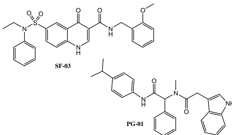
Figure 27 : Structures de SF-03 et de PG-01
