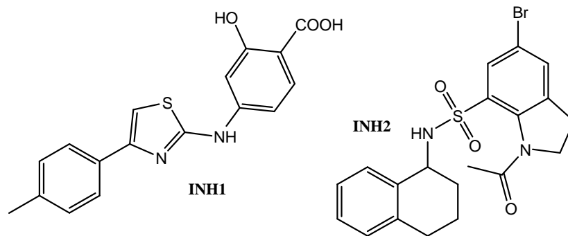
Figure 44 : Structure des composés INH1 et INH2
