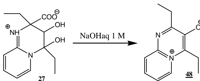
Schéma 17 : Formation du produit de la famille II 48 à partir des adduits EG-2-aminopyridine 27
