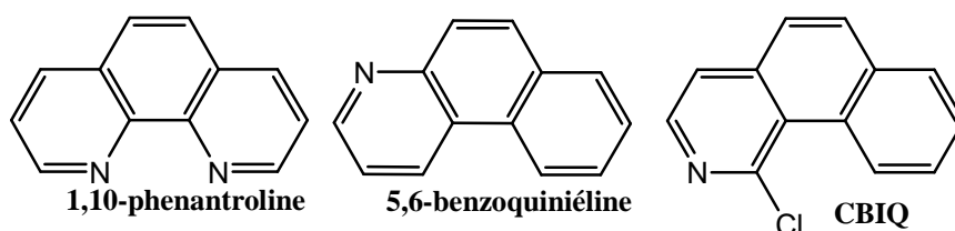
Figure 16 : Structure de la 1,10-phénantroline, du 7,8-benzoquinoléine et de CBIQ
