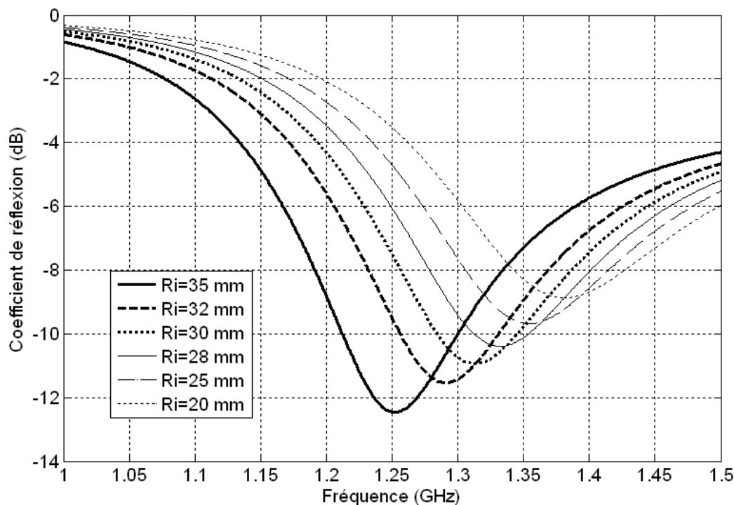
Figure II.13 Coefficients de réflexion simulés de la configuration 4 pour différents rayons de l'évidement
