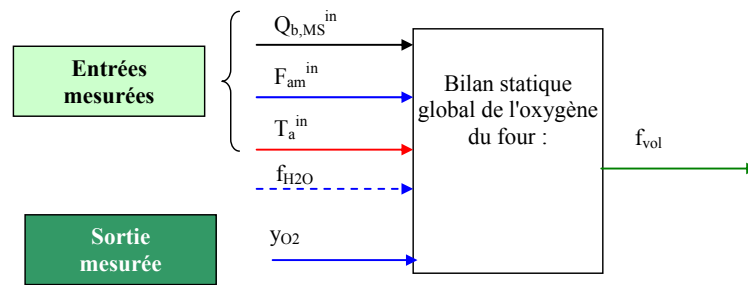
Figure 4.3. Modèle algébrique de reconstruction de la composition des boues
