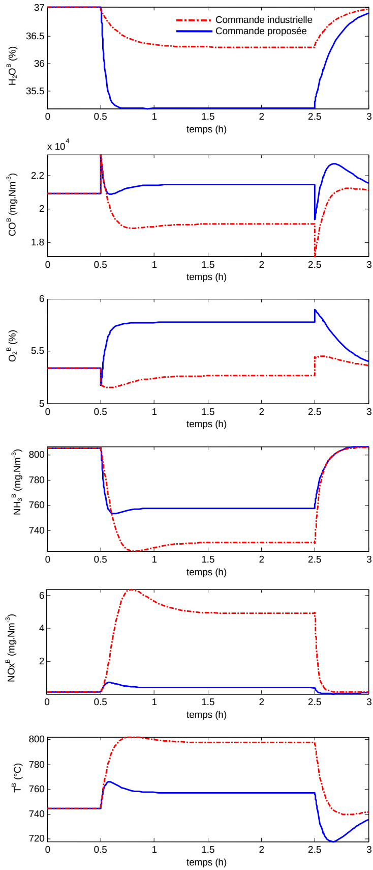
Figure E.8. Comparaison des variables d'état du lit bouillonnant pour les deux stratégies de commande (échelon sur f_{\text{CO}} )
