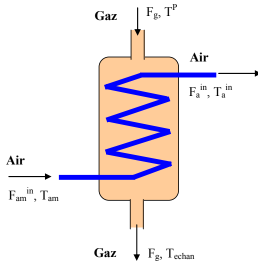
Figure 5.1. Schéma de principe de l'échangeur.
