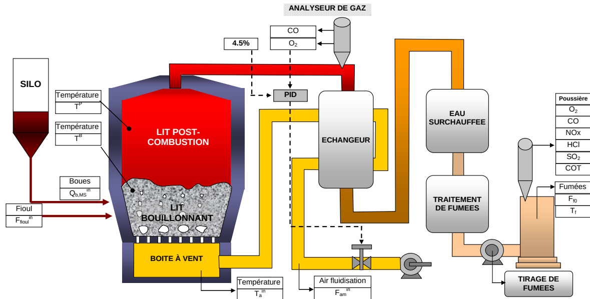
Figure C.1. Station d'incinération des boues d'épuration en lit fluidisé
