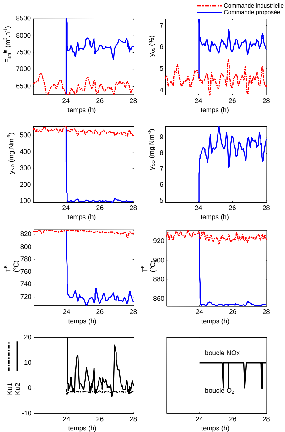
Figure F.1. Comparaison des stratégies de commande sur les mesures industrielles du fichier 3.
