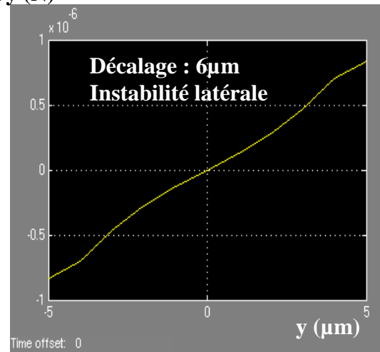
Figure 1-13 : dispositif magnétique de type RAIMI avec aimants fixes décalés vers l'extérieur (bobine non représentée) et énergie potentielle du système en fonction de la position latérale pour des aimants fixes de 10 \mu\text{m}
