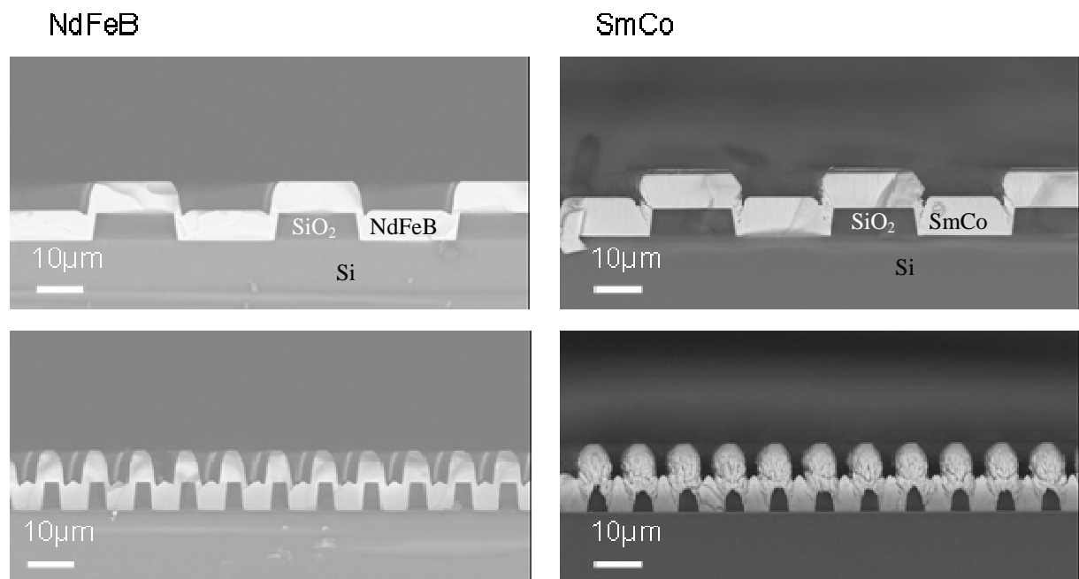
Figure 3-9 : vue MEB de dépôts de NdFeB et SmCo sur substrats avec caissons (SEM cross section view of NdFeB and SmCo films deposited on patterned substrate)
