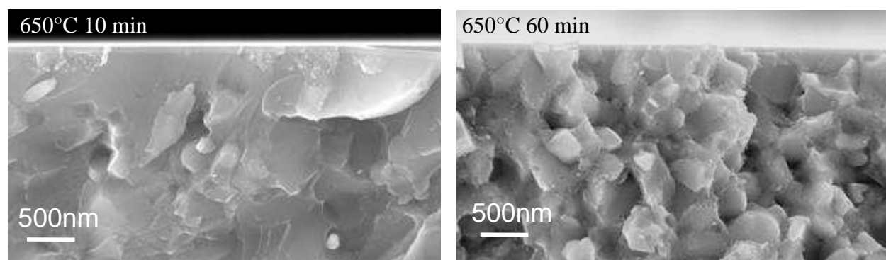
Figure 2-24 : microstructure observée par MEB d'un film de NdFeB déposé à froid et recuit à 650°C pendant, respectivement, 10 et 60 minutes (SEM view of the microstructure of NdFeB films deposited cold and annealed at 650°C for 10 and 60 min)
