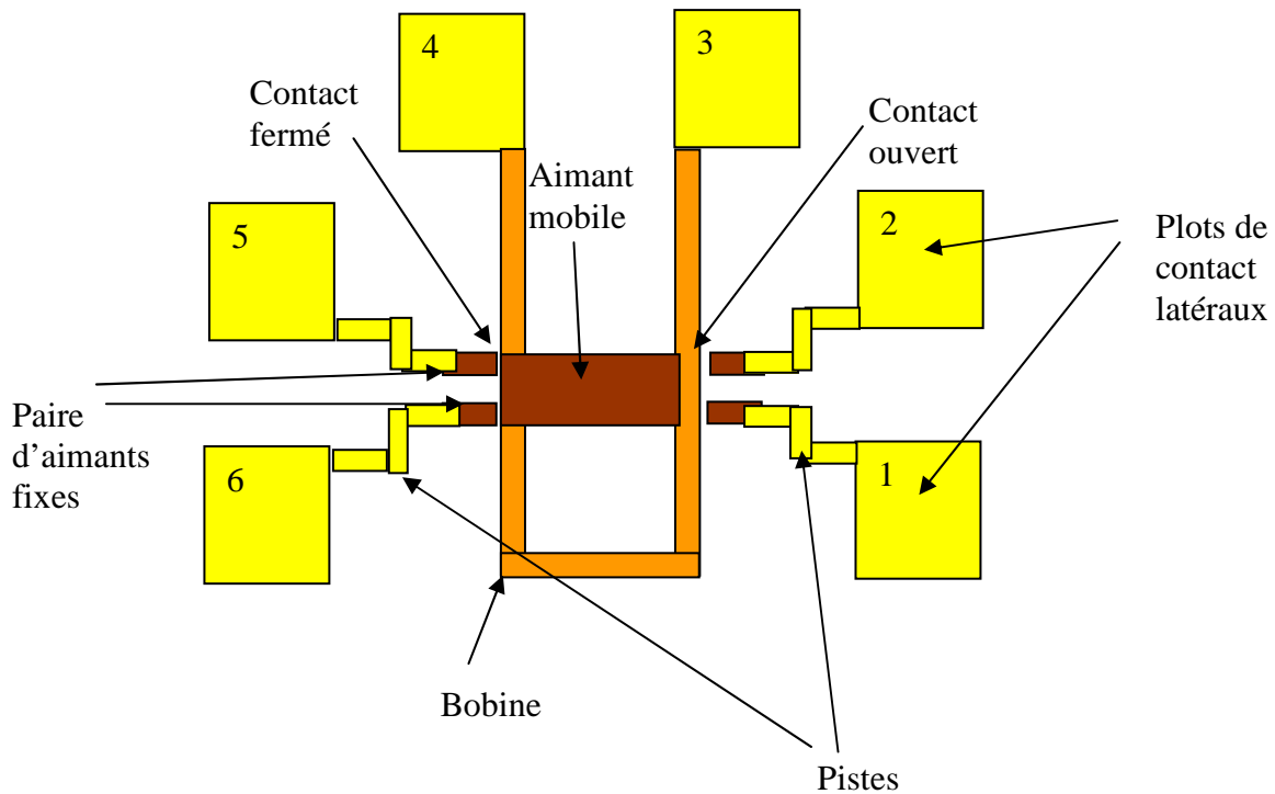
Figure 0-16 : schéma d'un actionneur RAIMI vue de dessus (Scheme of top view of RAIMI MEMS)
