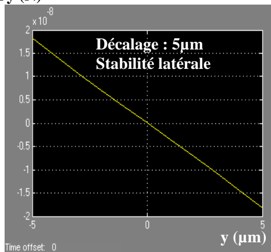
Figure 1-13 : dispositif magnétique de type RAIMI avec aimants fixes décalés vers l'extérieur (bobine non représentée) et énergie potentielle du système en fonction de la position latérale pour des aimants fixes de 10 \mu\text{m}
