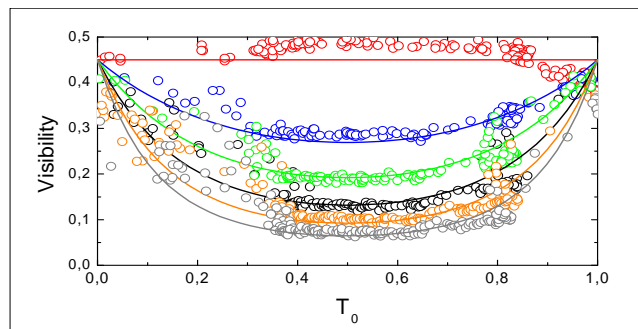
FIGURE 2.10 – (couleur sur la figure) Dépendance de la visibilité en fonction de T_0 pour V_2=0, 21, 31, 42, 53 et 63 \mu V de haut en bas. Les lignes en trait plein sont les fits aux données expérimentales en utilisant l'équation 2.3 avec V_\varphi = 7.2 \mu V et T=25mK .
