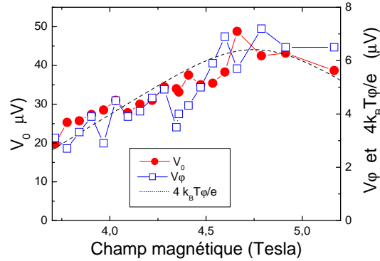
FIGURE 2.11 – (couleur sur la figure) V_0 et V_\varphi en fonction du champ magnétique. La courbe en pointillée est le comportement général de 4k_B T_\varphi/e (échelle à droite) mesuré sur le même échantillon.
