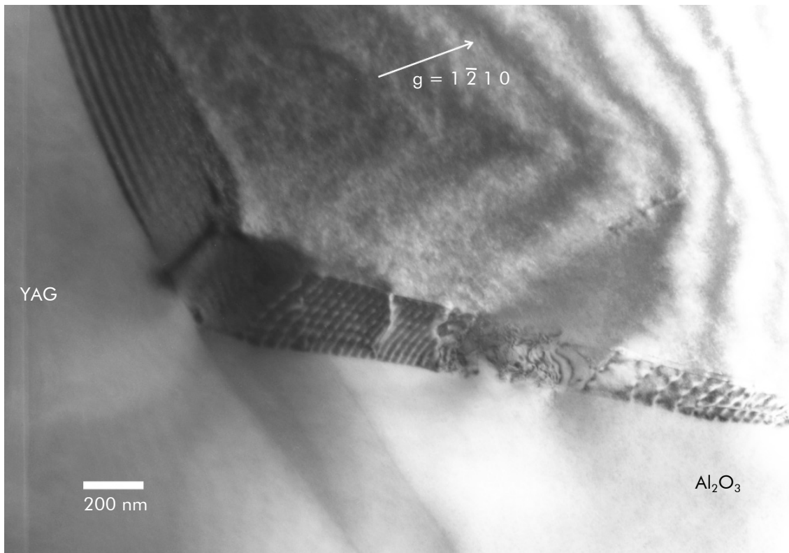
Figure 6.17 Micrographie MET du composite \text{Al}_2\text{O}_3 - YAG déformé à 1470^\circ\text{C} sous 70\text{ MPa} : empilement de dislocations dans la phase \text{Al}_2\text{O}_3 , contre une interface \text{Al}_2\text{O}_3/\text{YAG} .
