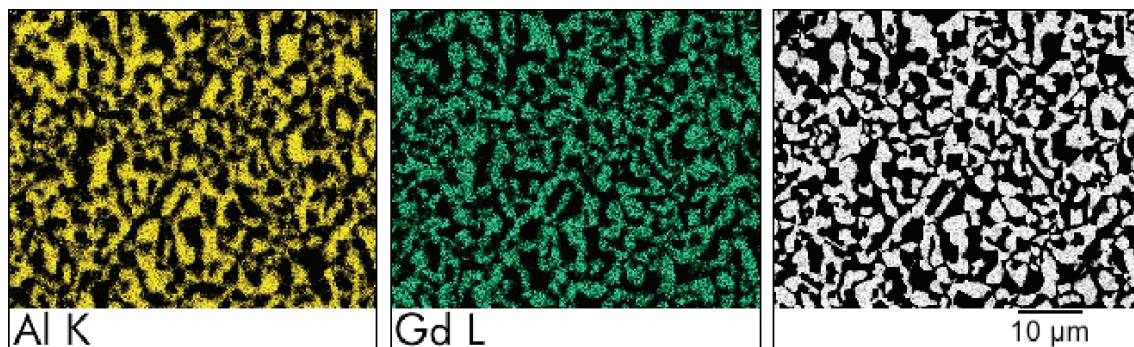
Figure 3.15 Cartographies élémentaires EDX effectuées, pour l'aluminium et le gadolinium, sur le composite in situ \text{Al}_2\text{O}_3 - GdAP.
