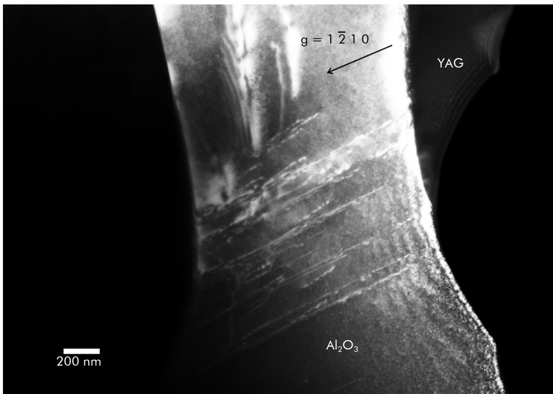
Figure 6.18 Micrographie MET en faisceau faible du composite \text{Al}_2\text{O}_3 - YAG déformé à 1470^\circ\text{C} sous 70\text{ MPa} : bande de glissement dans un domaine de phase \text{Al}_2\text{O}_3 .
