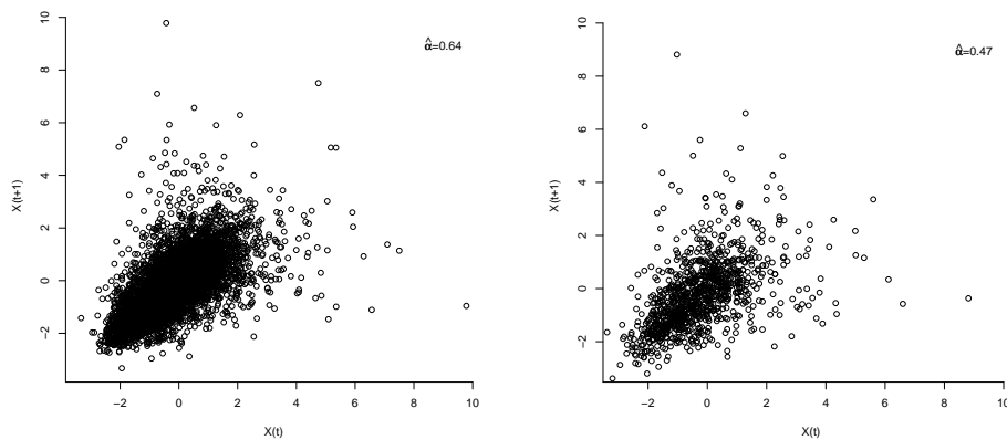
FIG. 4.13 – « Scatter plots » des valeurs successives, i.e. (X_t, X_{t+1}) , correspondant aux maxima journaliers (à gauche) et hebdomadaires (à droite) de CO_2 . L'unité est le ppm.
