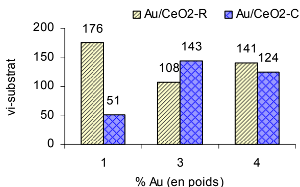
Figure IV.15 : Vitesses initiales de conversion de l'acide acétique ( v_{i\text{-substrat}} : \text{mole}_{\text{acide acétique}} \text{ mole}_{\text{Au}}^{-1} \text{ h}^{-1} ) en fonction du pourcentage d'or et de la nature du prétraitement (R : réduction ; C : calcination)
