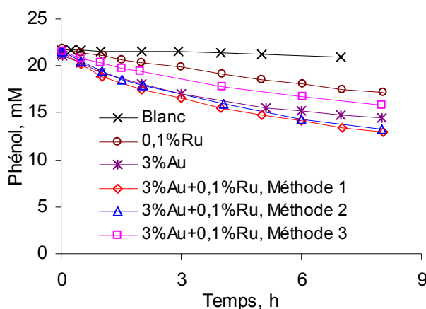
Figure VI.2 : OVHC du phénol sur catalyseurs mono- et bimétalliques à base d'or et de ruthénium supportés sur TiO 2 P25 (150 mL de phénol 2,07 g L -1 , 140°C, 50 bar de pression totale, 0,5 g de catalyseur)
