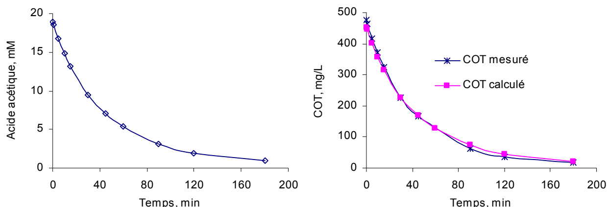
Figure IV.13 : OVHC de l'acide acétique sur 3%Au/CeO 2 préparé par DPA sous ultrasons, (150 mL d'acide acétique 1,2 g L -1 , 190°C, 50 bar de pression totale, 0,3 g de catalyseur)
