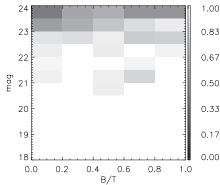
FIG. 10.5 – Complétude pour les sources étendues d'après les simulations analytiques de galaxies.
