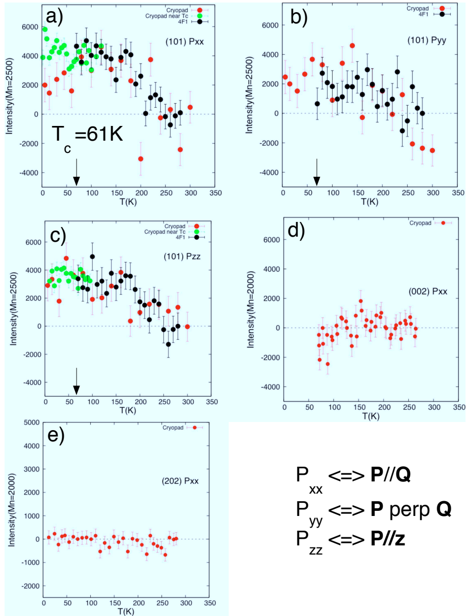
FIG. 5.8: Intensité magnétique déduite sur la raie (101) mesurée sur IN22 en configuration CRYOPAD pour différentes polarisations : a) P_{xx} ( P // Q ), b) P_{yy} ( P // Q_{\perp} ) et c) P_{zz} ( P // z ). d) Intensité magnétique mesurée sur la raie (0,0,2) pour la polarisation P_{xx} ( P // Q ). e) Intensité magnétique mesurée sur la raie (2,0,2) pour la polarisation P_{xx}
