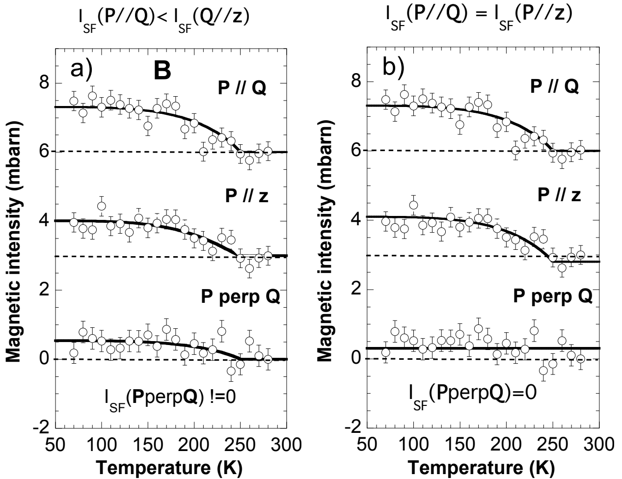
FIG. 5.5: Dépendance en température de l'intensité magnétique mesurée sur le pic de Bragg (0,1,1) de l'échantillon (B) pour trois polarisations différentes des neutrons : P//Q , P//z et P//q ⊥ . La ligne noire correspond à l'ajustement de chacun des canaux par la fonction : I_{mag}(T) = (1 - (\frac{T}{T_{mag}})^\alpha)^\beta , les paramètres \alpha, \beta et T_{mag} sont les mêmes pour les trois canaux. La ligne rouge correspond au cas où le moment serait purement le long de l'axe c.
