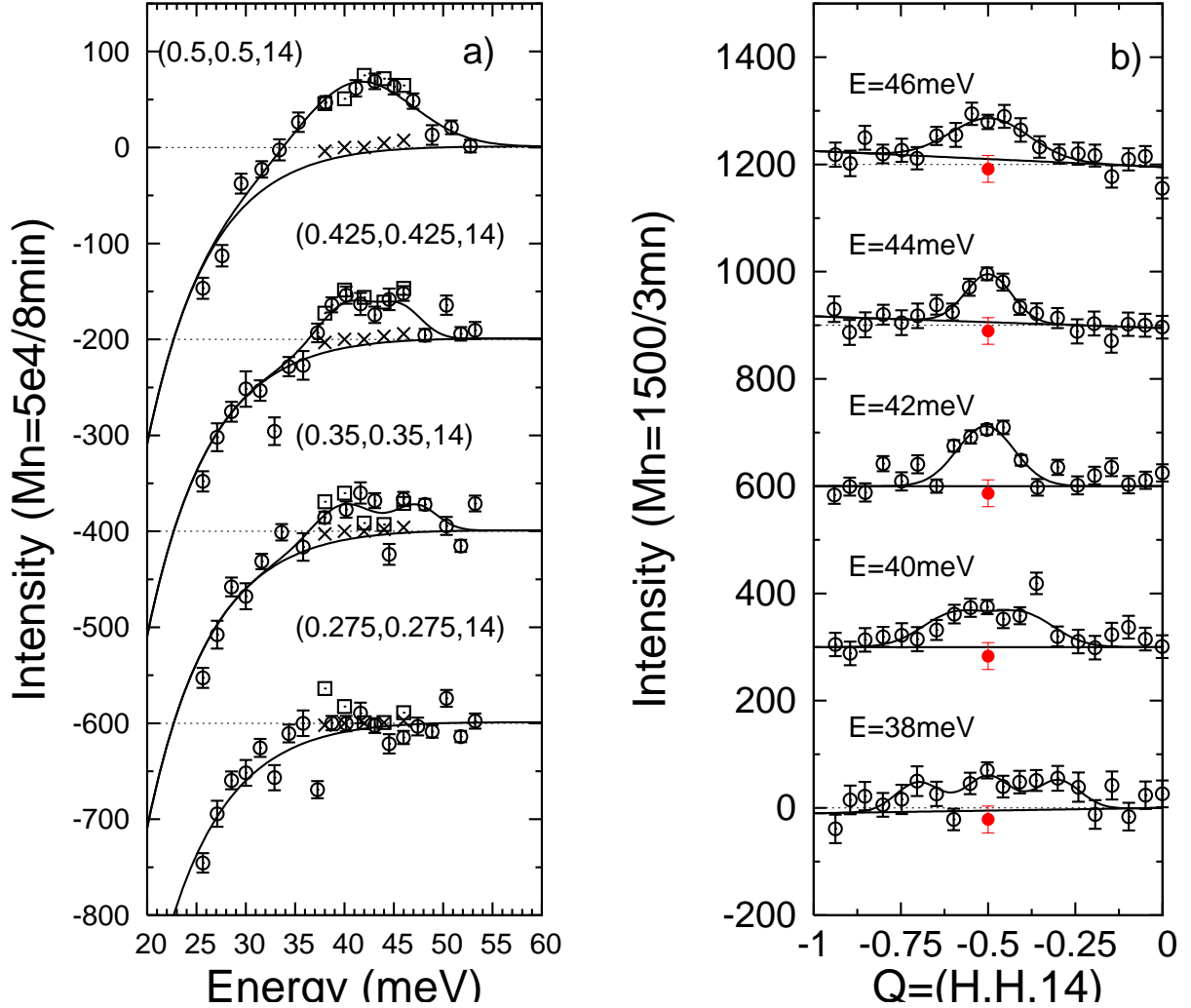
FIG. 3.6: Bi-2212 T_c=87K (légèrement surdopé) : a) Différences entre les coupes en énergie à T=10K et T=100K pour Q=(0.5,0.5,14.1) , (0.425,0.425,14.1) , (0.35,0.35,14.1) et (0.275,0.275,14.1) . La ligne noire correspond à un ajustement gaussien sur un bruit de fond déterminé par l'évolution de la différence en Q=(0.275,0.275,14.1) . Les points carrés et croix correspondent au signal mesuré le long des coupes à énergie constante (b). b) Différences entre les coupes le long de la direction (H,H,14) à T=10K et T=100K pour des énergies E=38,40,42,44 et 46meV . La ligne noire correspond à un ajustement gaussien sur un bruit de fond pris linéaire ou constant. Les points rouges correspondent au bruit de fond déduit des coupes en énergie (a)
