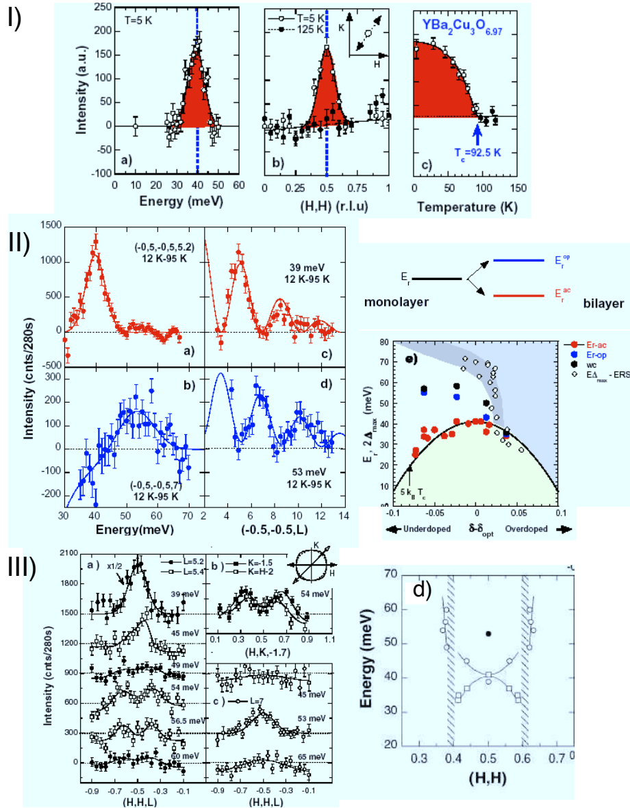
FIG. 1.7: I) Présentation du pic de résonance magnétique mesuré dans le composé \text{YBa}_2\text{Cu}_3\text{O}_{6.97} de T_c = 92.5\text{ K} par DIN : a) Intensité mesurée à basse température T = 5\text{ K} en fonction de l'énergie au vecteur d'onde AF, b) Intensité le long de la direction (H,H) pour une énergie de 41 meV à basse (point blanc) et haute température (point noir) c) Evolution en température mesurée aux vecteurs d'ondes Q = (0.5, 0.5, 4.7) pour une énergie de 41 meV. II) Différence entre les scans au vecteur d'onde AF à basse température et juste au dessus de T_c pour un échantillon \text{YBa}_2\text{Cu}_3\text{O}_{6.85} de T_c = 89\text{ K} a) et c) Pics de résonance magnétique dans le canal acoustique avec sa modulation typique en sinus carré b) et d) Même chose dans le canal optique. e) Dépendance en dopage de l'énergie caractéristique du mode acoustique (en rouge) et du mode optique (en bleu). Les deux modes se trouvent en dessous de 2\Delta_m qui représente l'énergie minimum pour créer une excitation élémentaire au vecteur d'onde AF. 2\Delta_m peut être mesuré par ARPES, SIS ou encore Raman. III) Différence d'intensité entre basse température ( T = 10\text{ K} ) et T_c plus 10K dans un échantillon \text{YBa}_2\text{Cu}_3\text{O}_{6.85} de T_c = 89\text{ K} , le long de la direction (H,H) pour différentes énergies a) L = 5.2 ou 5.4 (canal acoustique) c) L = 7 (canal optique) et b) coupe à énergie constante pour deux directions de l'espace réciproque (1,0,0) et (1,1,0) d) Dispersion des excitations magnétiques dans la phase supraconductrice déduite des mesures reportées en a).
