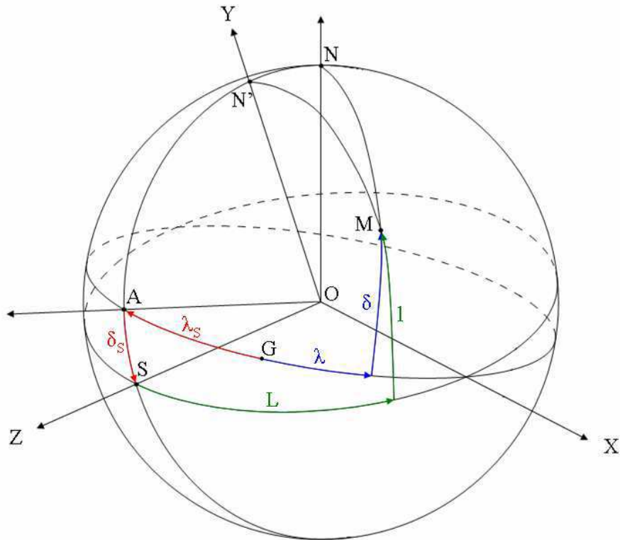
FIG. A.3: Schéma représentant le repère OXYZ , des longitudes et latitudes apparentes (L,l) et le repère des longitudes et latitudes planétaires (\lambda,\delta) . Le point M est le point dont on cherche les coordonnées. Le point S est le point sub-terrestre. Le point G est le point d'intersection de l'équateur et du méridien de référence : c'est l'origine des longitudes et latitudes planétaires. Le point N est le pôle Nord. Le point N' est le point d'intersection entre l'axe OY et le méridien central. Enfin, le point A est le point d'intersection entre l'équateur et le méridien central.
