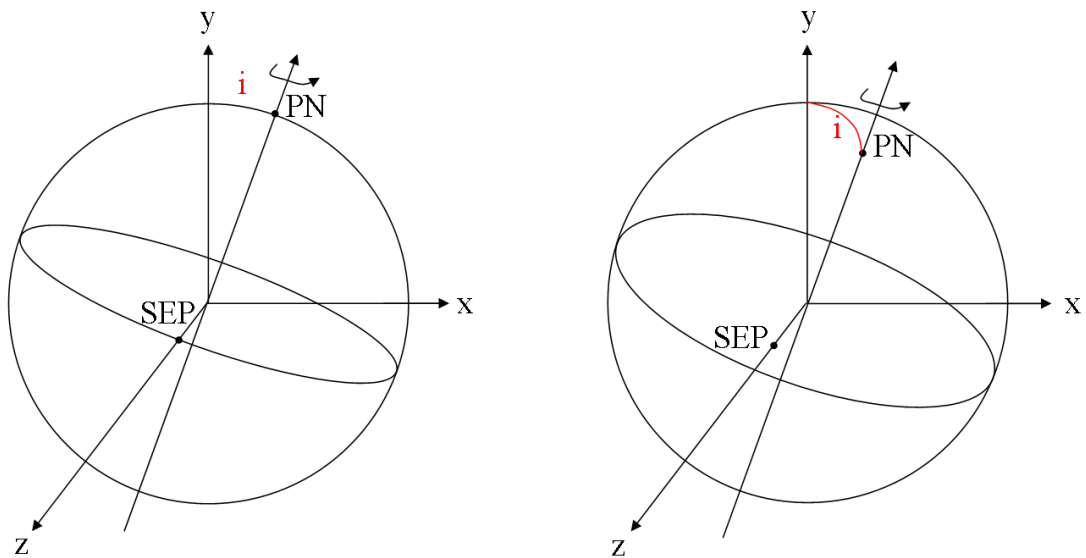
FIG. 4.5: Au gauche, le cas d'un axe de rotation de la planète qui se trouve dans le plan xOy (orthogonal aux lignes de visée). Quand l'axe de rotation n'est pas dans le plan xOy (à droite), la prise en compte du smearing nécessite une modélisation des points émetteurs du disque par leurs coordonnées planétaires (L,l) . C'est surtout le cas si la planète est résolue spatialement et que le télescope pointe un pôle par exemple. Le point sub-terrestre est noté SEP et le pôle Nord est noté PN.
