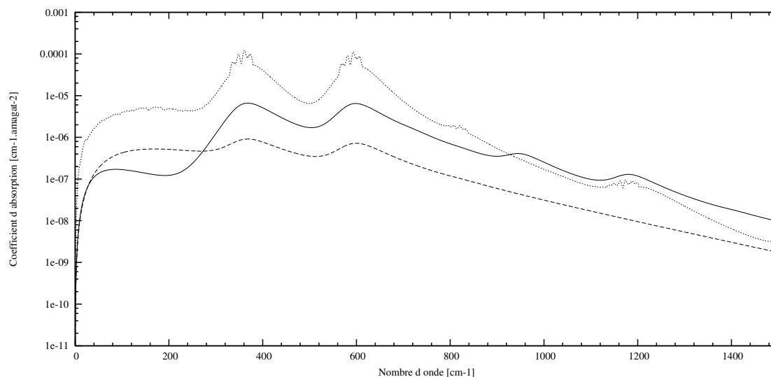
FIG. 1.2: Spectre des coefficients \kappa_{\text{H}_2-\text{H}_2} (trait plein), \kappa_{\text{H}_2-\text{He}} (tirets) et \kappa_{\text{H}_2-\text{CH}_4} (pointillés) en fonction du nombre d'onde [ \text{cm}^{-1} ], pour une température de 100 K.
