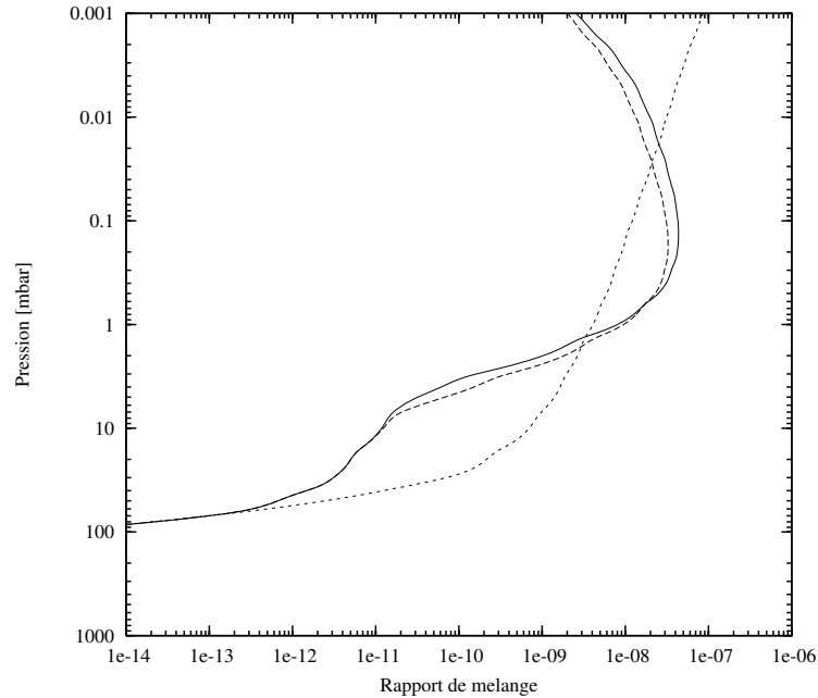
FIG. 3.4: Profil vertical du rapport de mélange de l'eau en fonction de la pression. Le modèle SL9 où p_0=0.2 mbar et q_0=(1.8\pm 0.2)\times 10^{-7} à l'époque des observations SWAS 1999 est tracé en trait plein. Le même modèle, tracé à l'époque des observations SWAS 2001, figure en tirets longs. Enfin, le modèle IDP, avec un flux stationnaire de \phi_{\text{H}_2\text{O}}^{\text{IDP}}=3.4\times 10^6 \text{cm}^{-2}\cdot\text{s}^{-1} est tracé en tirets courts. La densité de colonne est de n_{\text{H}_2\text{O}}=3.5\times 10^{15} \text{cm}^{-2} pour le modèle SL9 au moment des impacts et n_{\text{H}_2\text{O}}=2.6\times 10^{15} \text{cm}^{-2} pour le modèle IDP.
