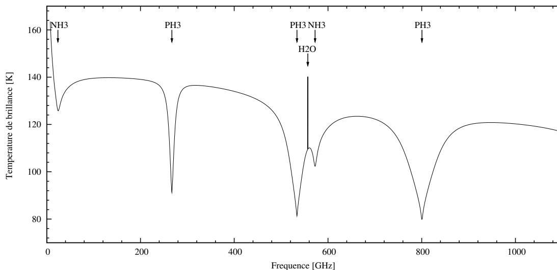
FIG. 1.7: Spectre simulé de la planète Saturne, en fonction de la fréquence, entre 0 GHz et 1100 GHz, qui tient uniquement compte de la présence d'ammoniac ( \text{NH}_3 ), de phosphine ( \text{PH}_3 ) et d'eau ( \text{H}_2\text{O} ). Le modèle utilisé pour simuler ce spectre sera vu dans la partie II.
