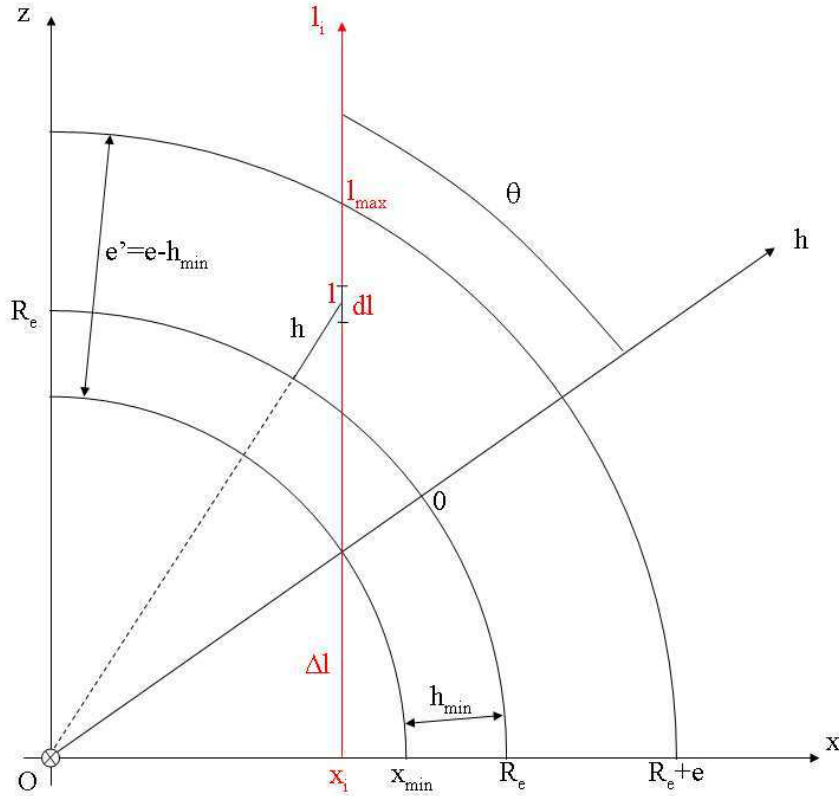
FIG. 2.3: Schéma qui permet de définir les variables qui sont nécessaires à la détermination de l'épaisseur d'atmosphère qu'une ligne de visée l_i traverse.
