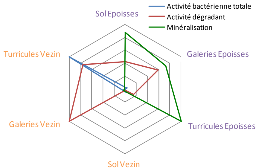
Figure V-2 : Un exemple de synthèse des résultats obtenus durant le travail de thèse dans les microsites des sols d'Epoisses et de Vezin (violet et orange). L'activité bactérienne totale correspond au nombre de gènes codant pour l'ARNr 16S exprimés 7 jours après l'addition de 1.5 mg d'atrazine par kg de sol sec, l'activité des dégradants au nombre de gènes atzD exprimés 7 jours après l'addition de 1.5 mg d'atrazine par kg de sol sec et la minéralisation au taux de minéralisation de 14 C-atrazine dans les 3 jours suivant son apport à une concentration de 1.5 mg par g de sol sec.
