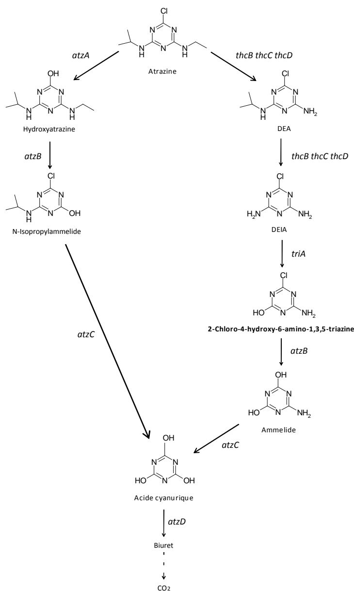
Figure V-3 : Voies de dégradation potentiellement utilisées par les bactéries des sols d'Époisses et de Vezin.
