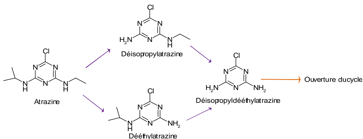
Figure I-14 : Dégradation de l'atrazine par la souche Nocardia . Les flèches violettes représentent des réactions biotiques et la flèche orange une réaction abiotique (d'après Giardina et al., 1982).
