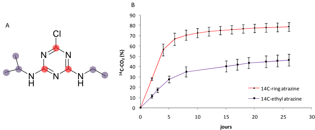
Figure II-13: A. Molécule d'atrazine et les carbones marqués pour la minéralisation, B. Minéralisation de l'atrazine avec le marquage 14 C sur les chaînes ou sur le cycle.
