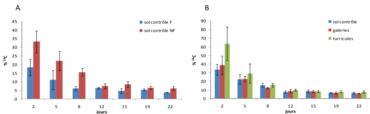
Figure II-17 : A. Pourcentage de ^{14}C retrouvé dans le sol contrôle fumigé et non fumigé, B. Pourcentage de ^{14}C retrouvé dans le sol contrôle, les galeries et les turricules non fumigés
