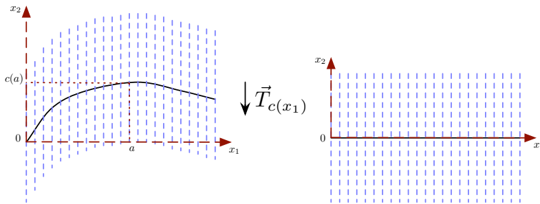
FIGURE 1.8 – Redressement d'un contour plutôt horizontal par translation suivant le vecteur \vec{T}_{c(x_1)} .
