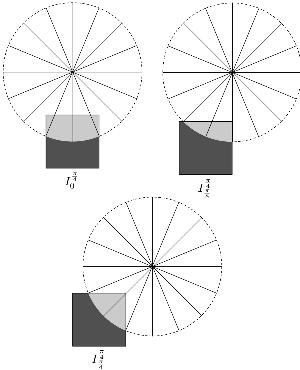
FIGURE 2.21 – Illustration de la génération des images de tests contenant une portion de disque de longueur d'arc \frac{\pi}{4} .
