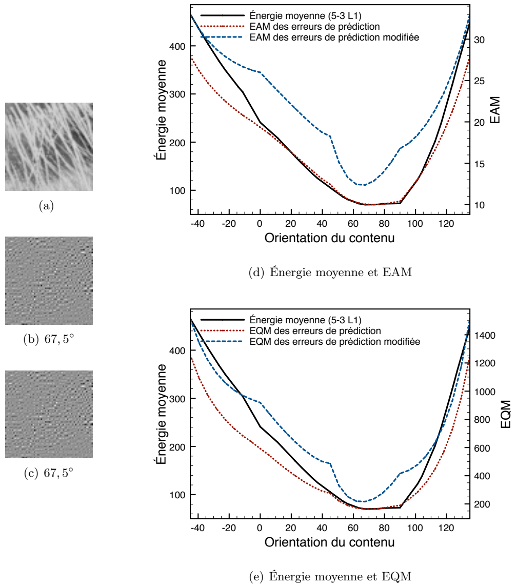
FIGURE 3.5 – Énergie de l’image baboon_mouth_hair (a) de dimension 64 \times 64 , reconstruite à partir des coefficients des hautes fréquences spatiales uniquement en fonction de l’orientation de filtrage, et mesures d’erreurs de prédiction selon 32 orientations uniformément réparties sur [-45^\circ, 135^\circ[ . (b) et (c) représentent les sous-bandes reconstruites des hautes fréquences dans la direction de filtrage qui minimise l’EAM des erreurs de prédiction respectivement non modifiée et modifiée.
