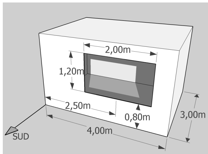
Figure IV.6 : Géométrie du cas test étudié
