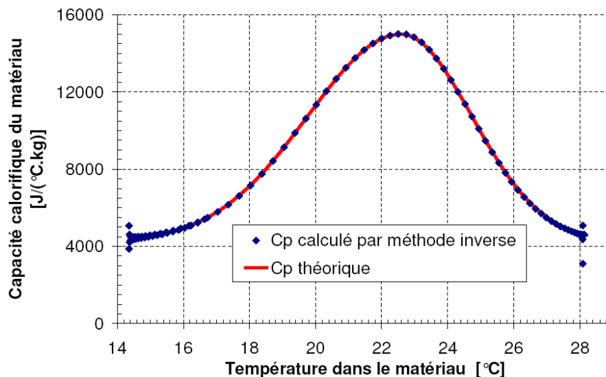
Figure IV.22 : Capacité calorifique obtenue par méthode inverse ou par le modèle
