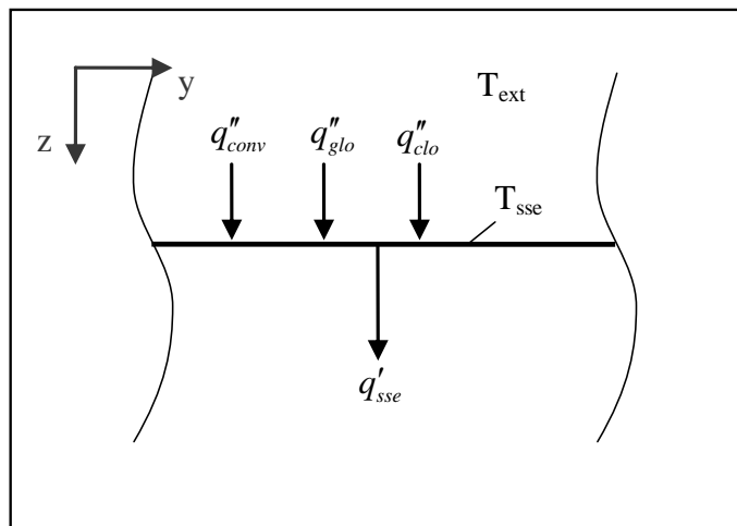
Figure III.18 : Bilan des échanges en surface du sol
