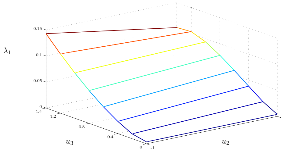
FIG. 4.2 – Variation du paramètre \lambda_1 du modèle réduit moyen [voir équation (4.5)]
