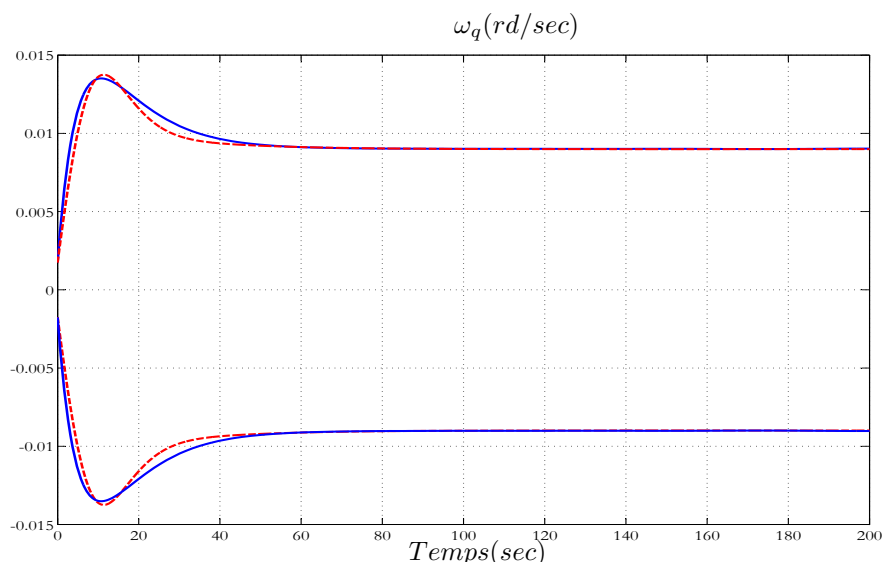
FIG. 4.14 – Evolution de \omega_q pour les modèles continu et réduit (traits interrompus et continus respectivement) en appliquant les entrées de commande ( u_3 = 0.6 , u_2 = -1 ( V_1 = 24 \text{ cm/sec} ), u_1 = 0 , \alpha = \pm 14^\circ , \beta = 0 )
