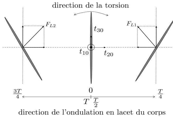
FIG. 3.31 – Mouvement sinusoïdale de torsion appliqué à la partie arrière du corps avec son ondulation en lacet. La figure montre la position de cette partie arrière ainsi que son mouvement de torsion pour une période d'ondulation. F_{L1} et F_{L2} sont les forces latérales exercées par le fluide sur la partie arrière du corps au maximum de l'ondulation. Dans le cas de cette figure, l'effet résultant est une force poussant le robot vers le haut avec tangage vers le bas.
